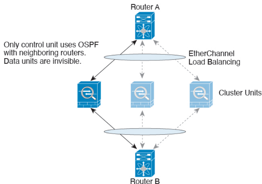
图 16: 动态路由
