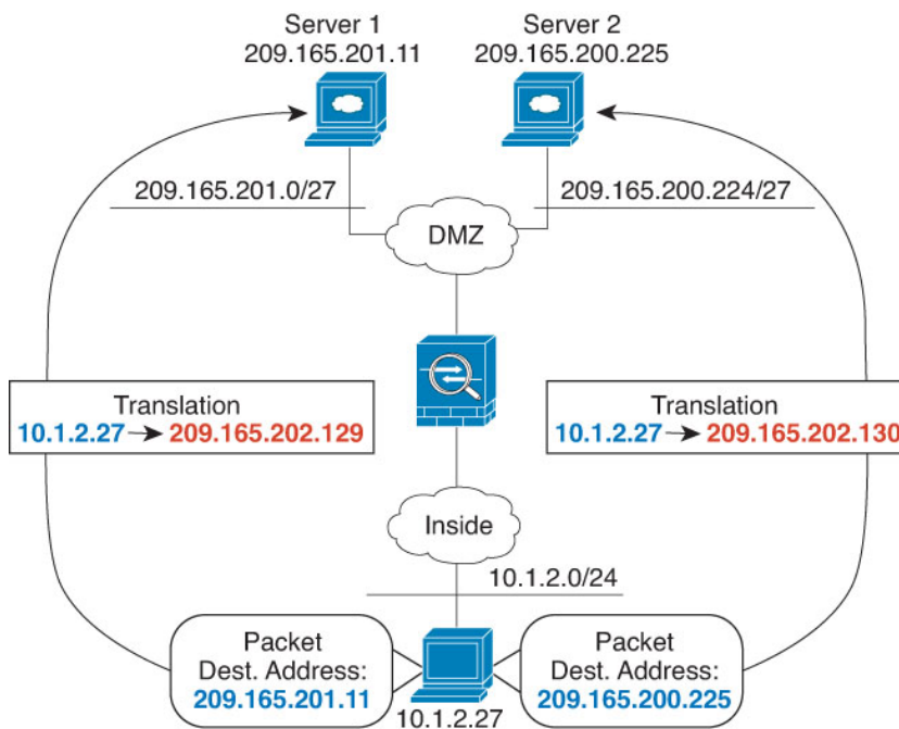
图 376: 具有不同目标地址的手动 NAT
