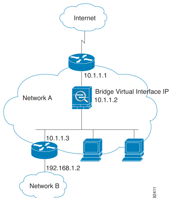
图 95: 透明防火墙网络
