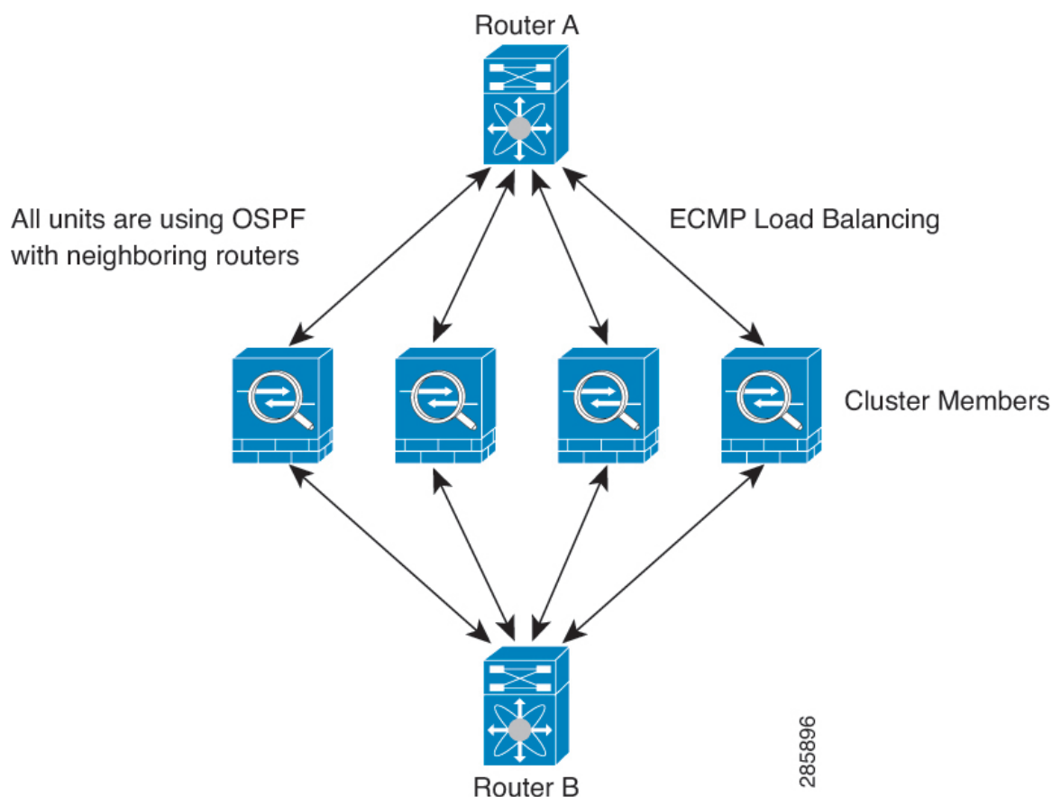
图 241: 独立接口模式下的动态路由
