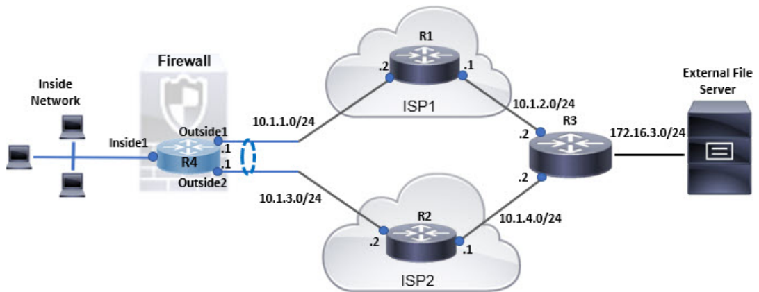
图 384: ECMP 的配置示例
