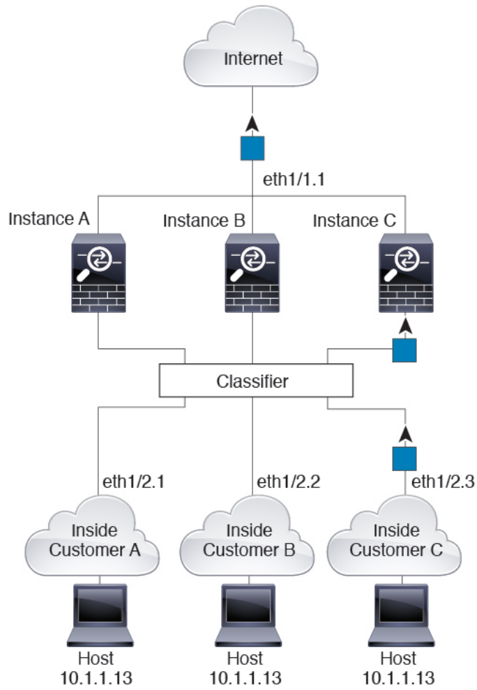
图 115: 来自内部网络的传入流量
