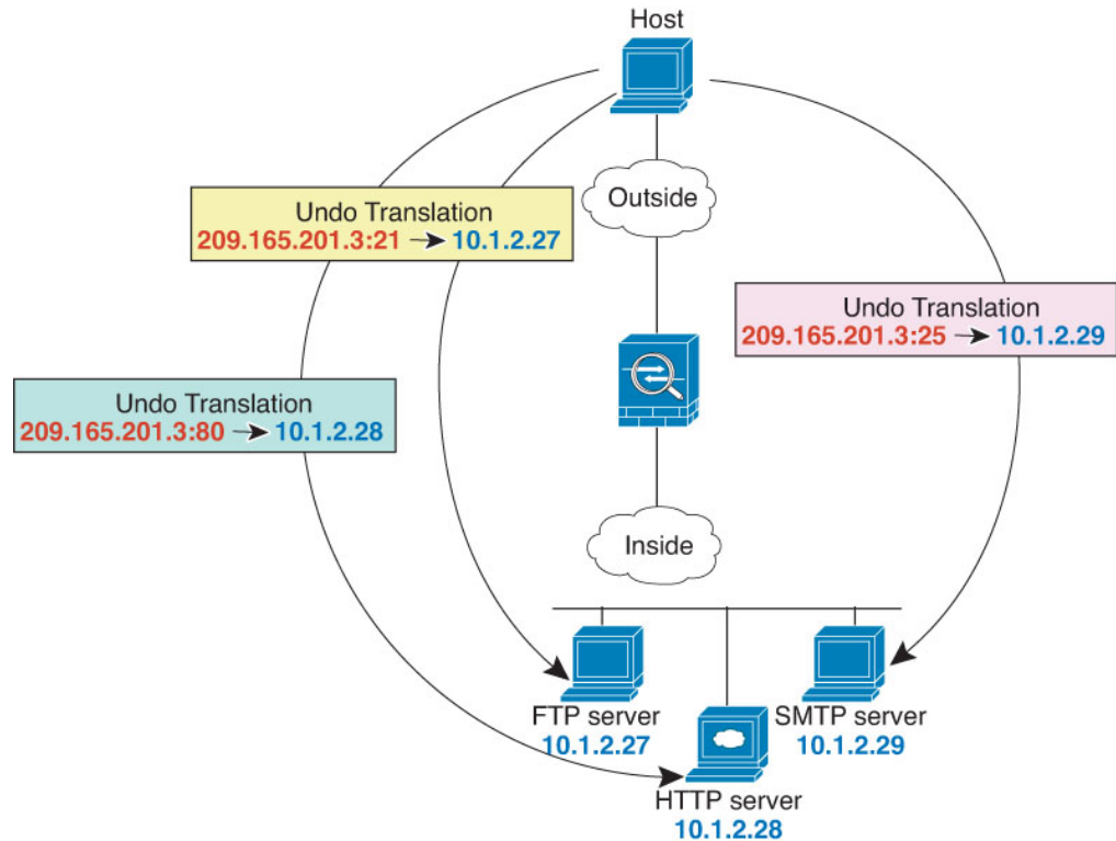
图 375: 支持端口转换的静态 NAT
