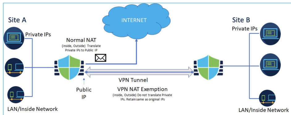
图 361: 具有 NAT 豁免的站点间 VPN 拓扑
