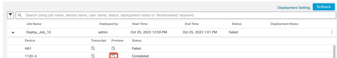
图 90: 预览图标
