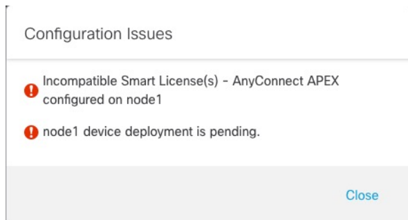
图 178: 配置问题
