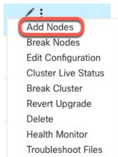
图 222: 添加节点
