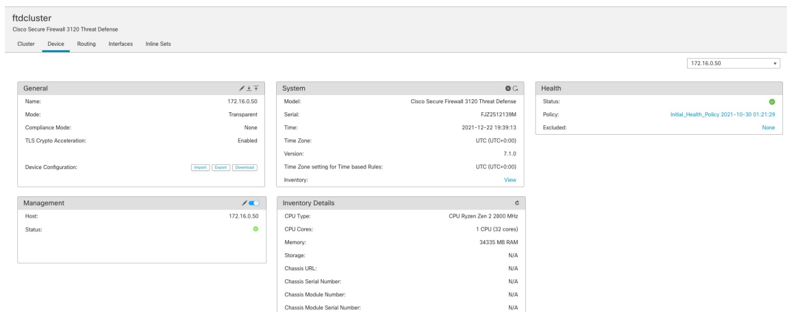
图 217: 选择节点
