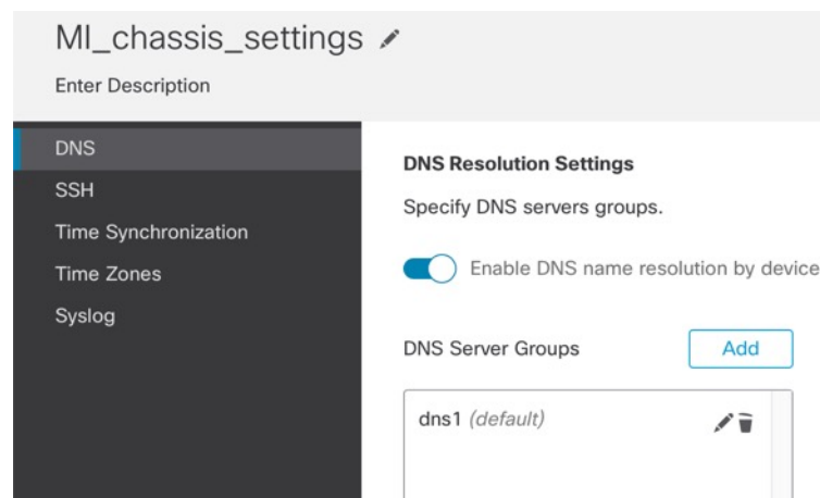
图 151: DNS
