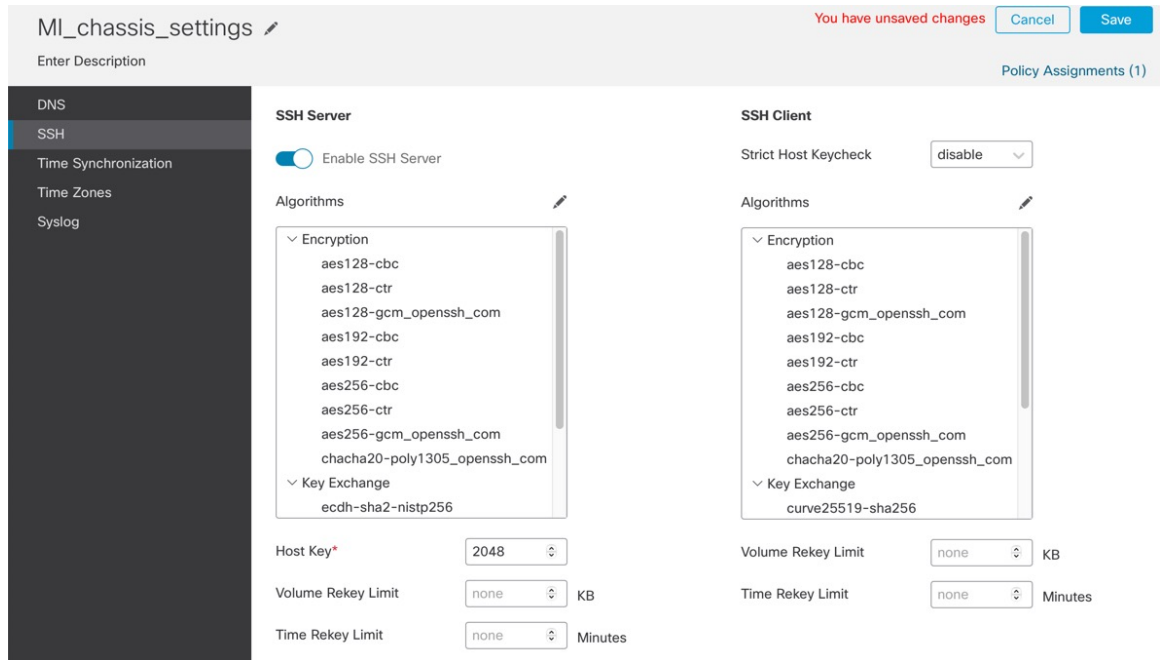
图 156: SSH
