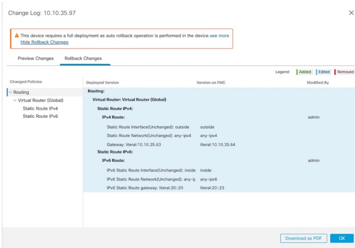
图 69: 回滚更改
