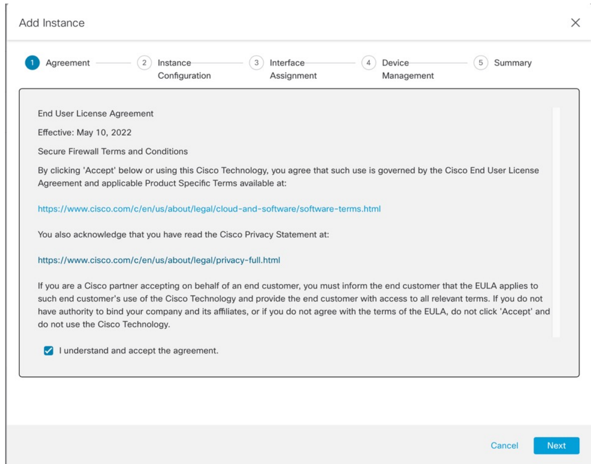
图 138: 协议
