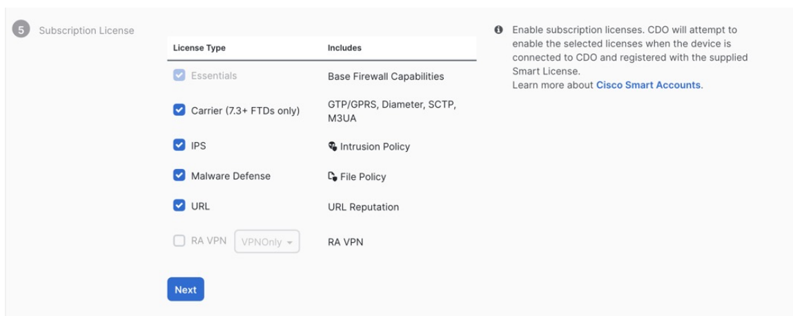
图 20: 订用许可证
