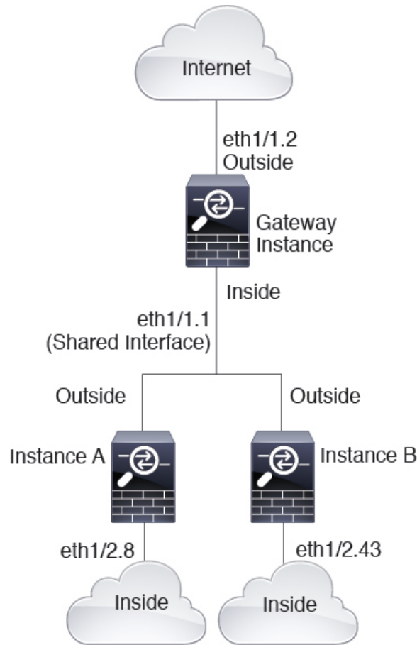
图 108: 级联实例
