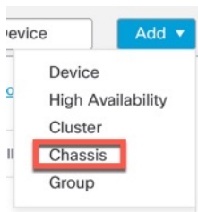
图 121: 添加机箱
