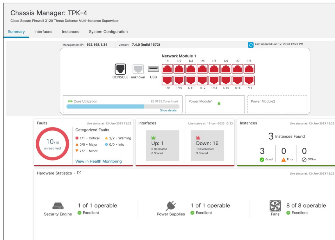
图 122: 机箱摘要
