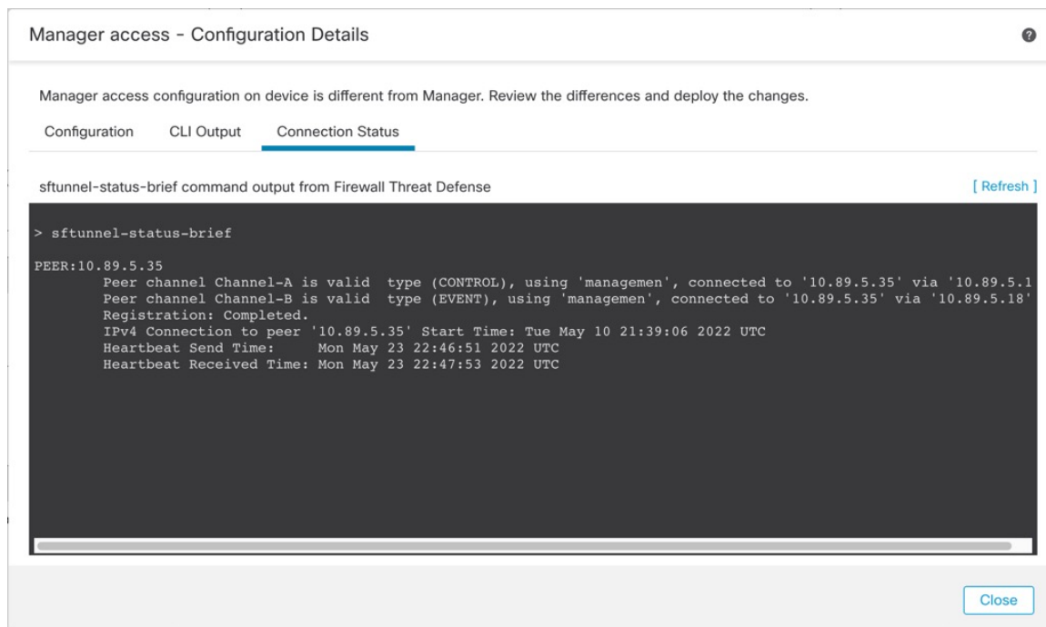
图 61: 连接状态
