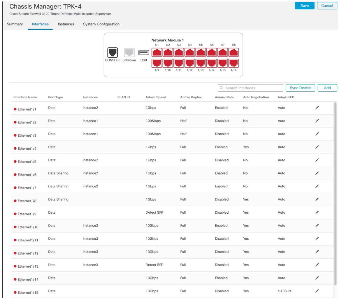
图 133: 接口
