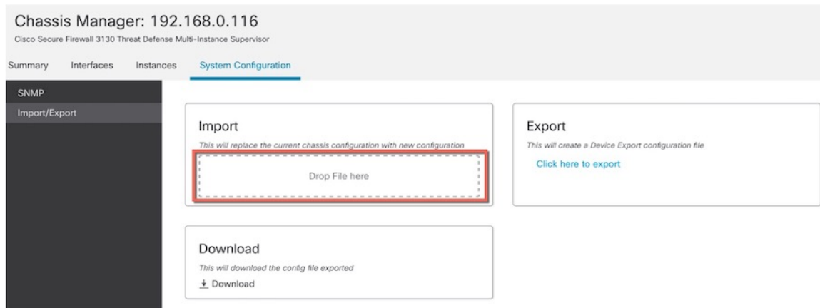
图 150: 导入
