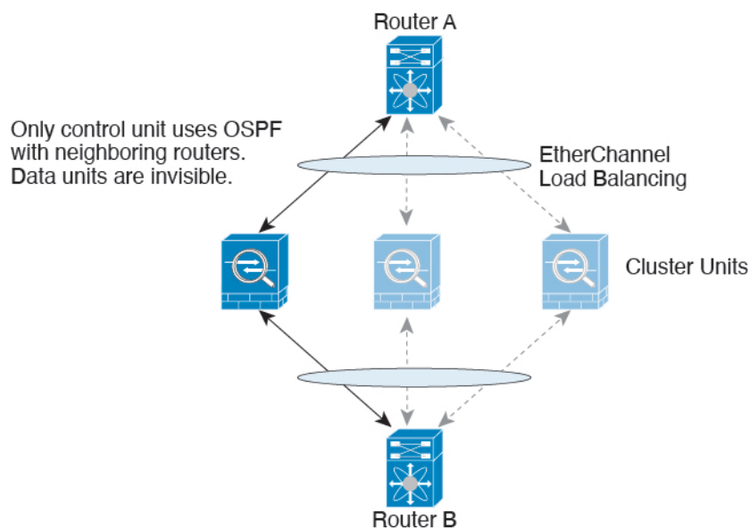
图 288: 动态路由
