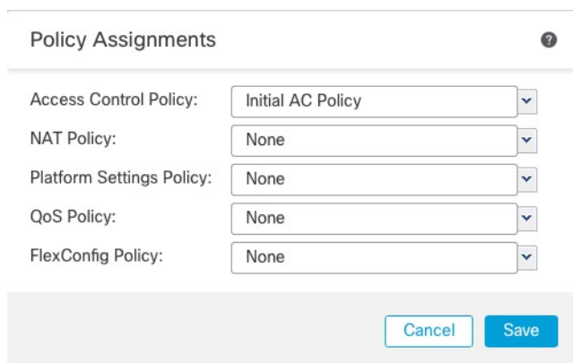
图 66: 策略分配
