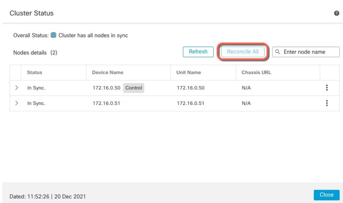
图 201: 协调全部
