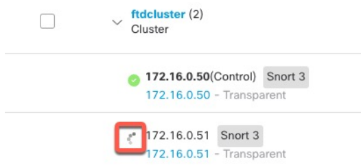
图 191: 节点注册
