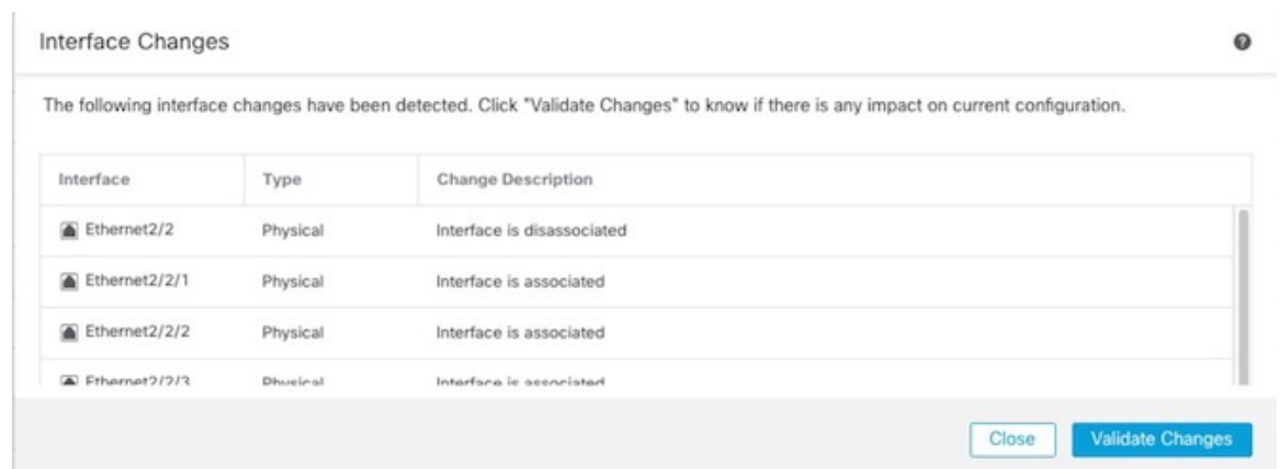
图 300: 接口更改
