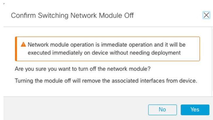
图 317: 确认禁用
