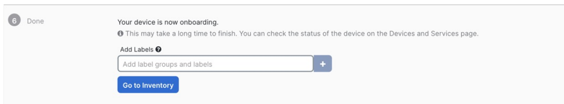
图 21: 完成
