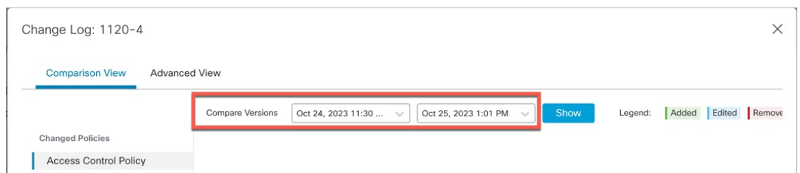
图 91: 比较版本
