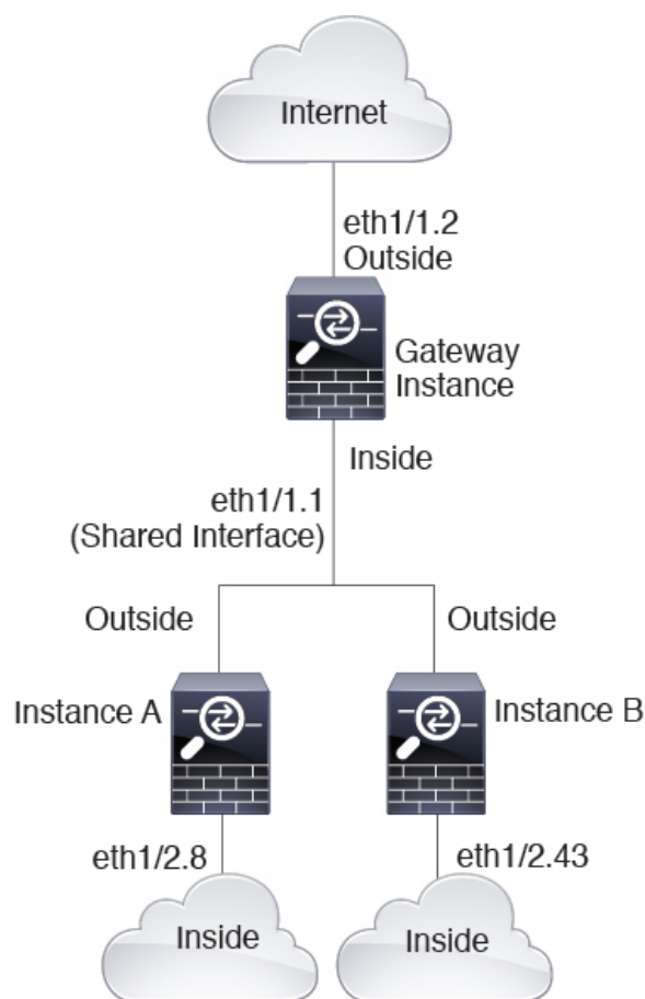
图 118: 级联实例
