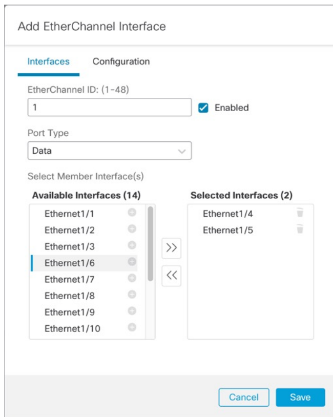
图 130: 接口设置
