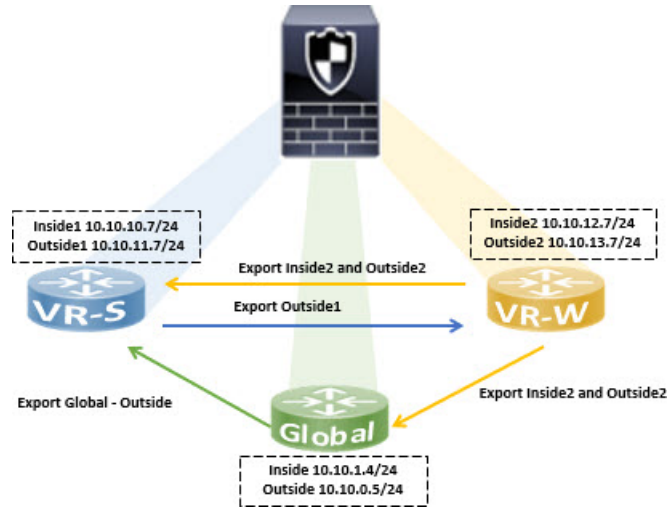
图 383: 使用 BGP 设置来互连虚拟路由器
