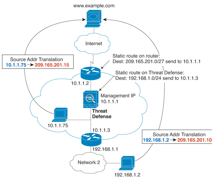
图 359: NAT 示例：透明模式
