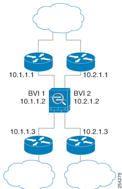
图 96: 具有两个网桥组的透明防火墙网络
