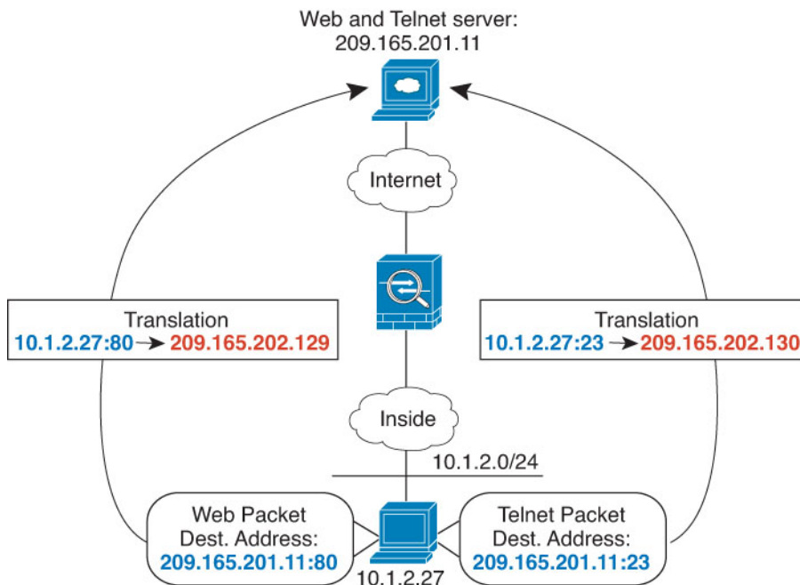
图 377: 具有不同目标端口的手动 NAT
