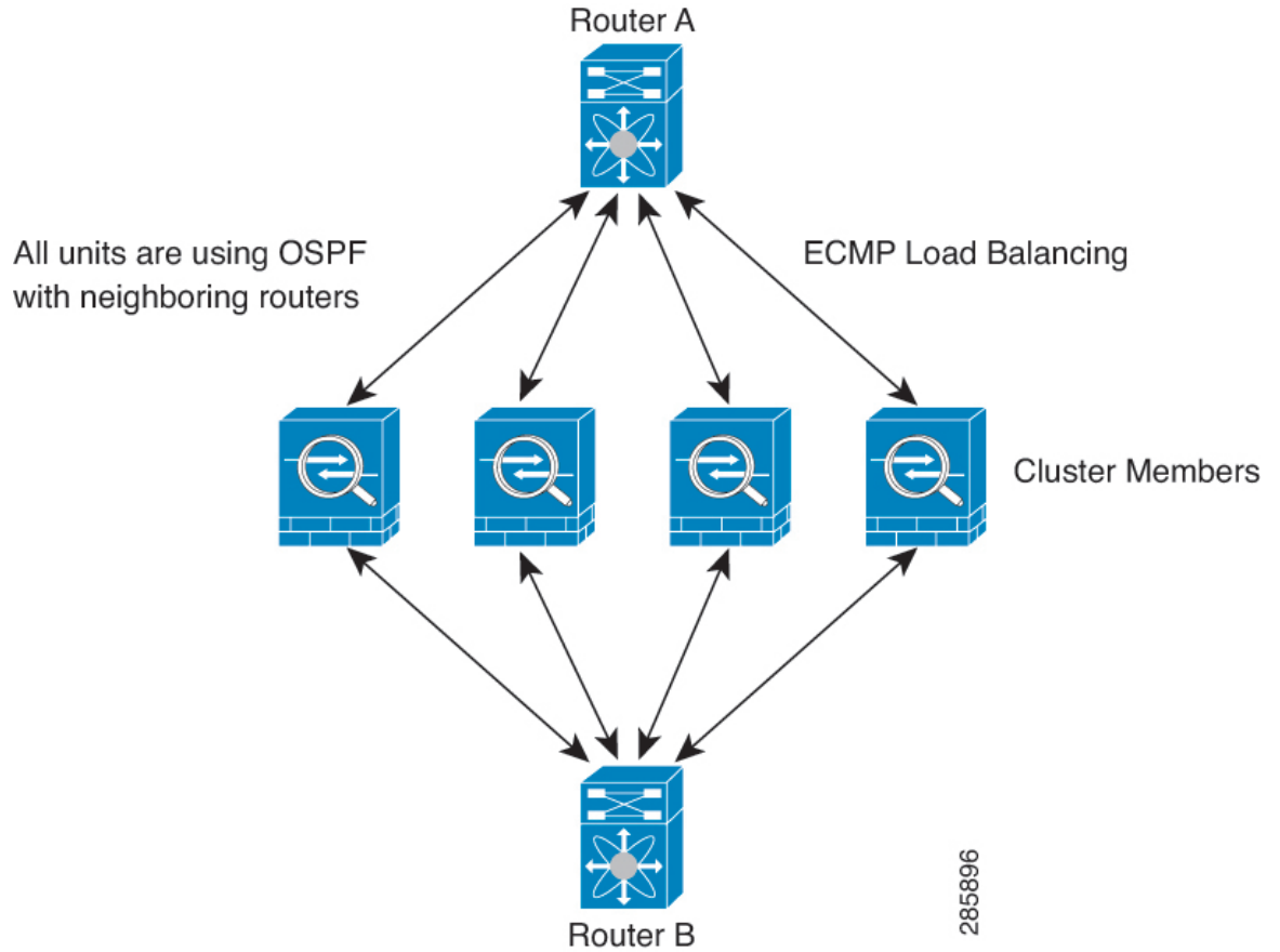
图 380: 独立接口模式下的动态路由
