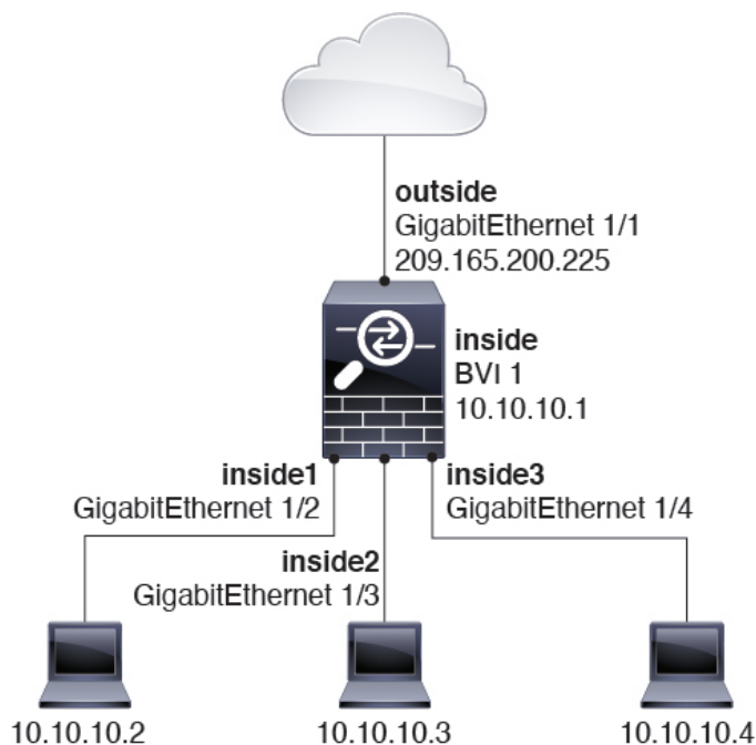
图 97: 具有内部网桥组和外部路由接口的路由防火墙网络
