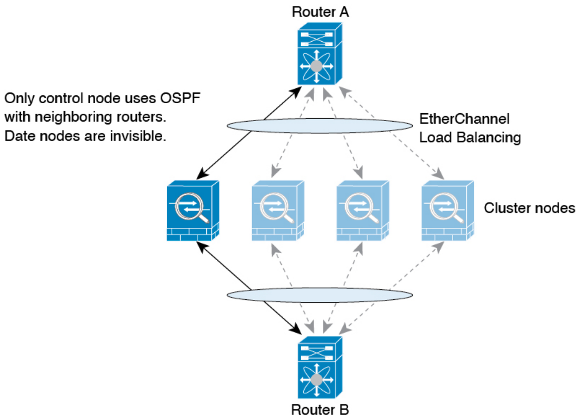
图 208: 跨区以太网通道模式下的动态路由
