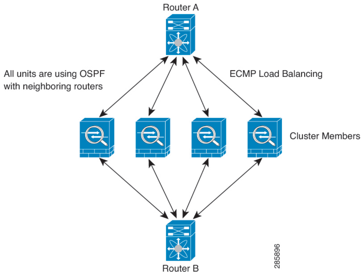
图 271: 独立接口模式下的动态路由
