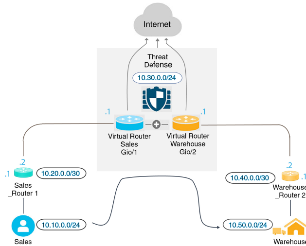
图 381: 互联两个虚拟路由器 - 示例
