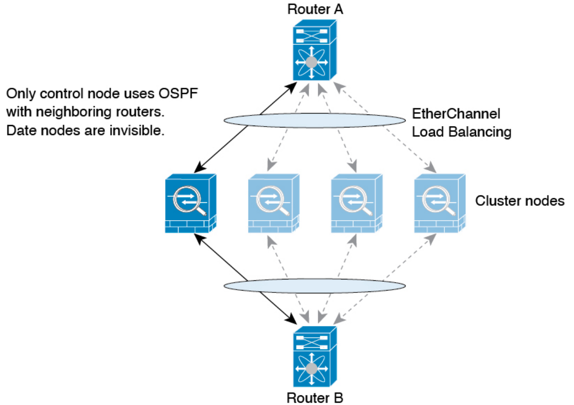
图 379: 跨区以太网通道模式下的动态路由
