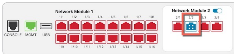
图 297: 分支端口
