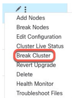
图 194: 中断集群
