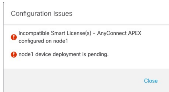
图 211: 配置问题
