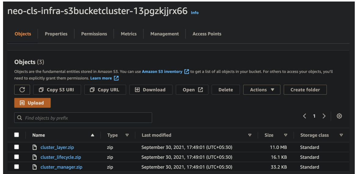
图 245: S3 桶
