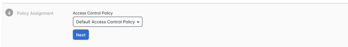
图 19: 策略分配
