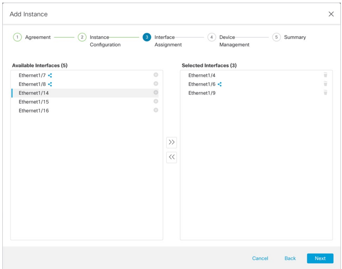
图 141: 接口分配
