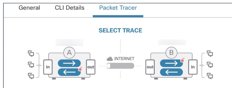
图 398: Packet Tracer
