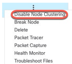
图 196: 禁用集群
