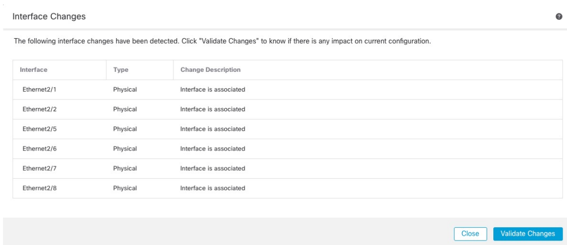
图 322: 接口更改
