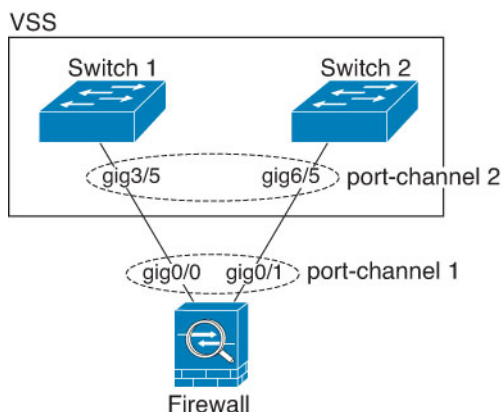
图 290: 连接至 VSS/vPC
