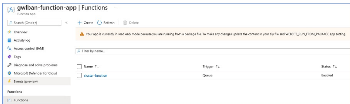
图 253: 功能
