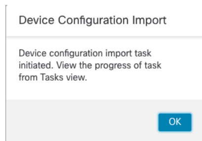
图 38: 确认导入
