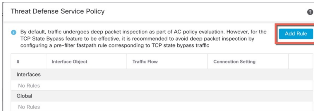
图 340: 添加规则
