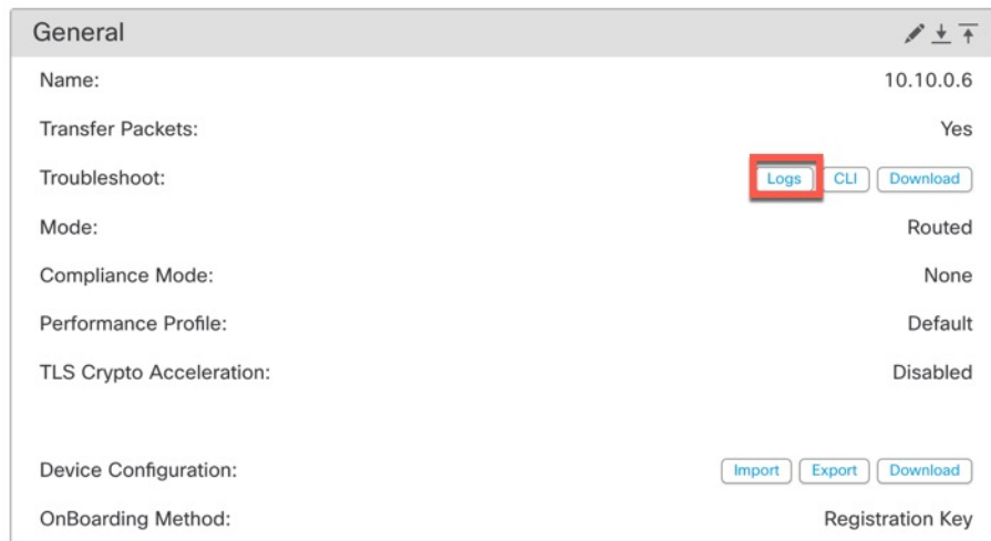
图 26: 日志
