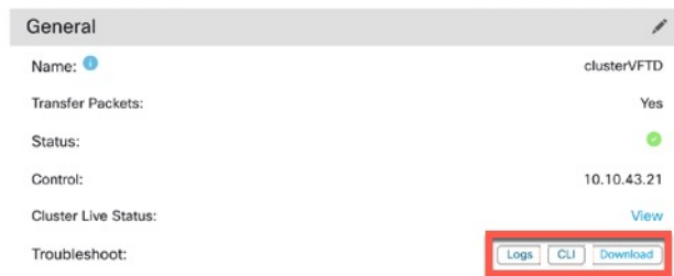
图 281: 故障排除
