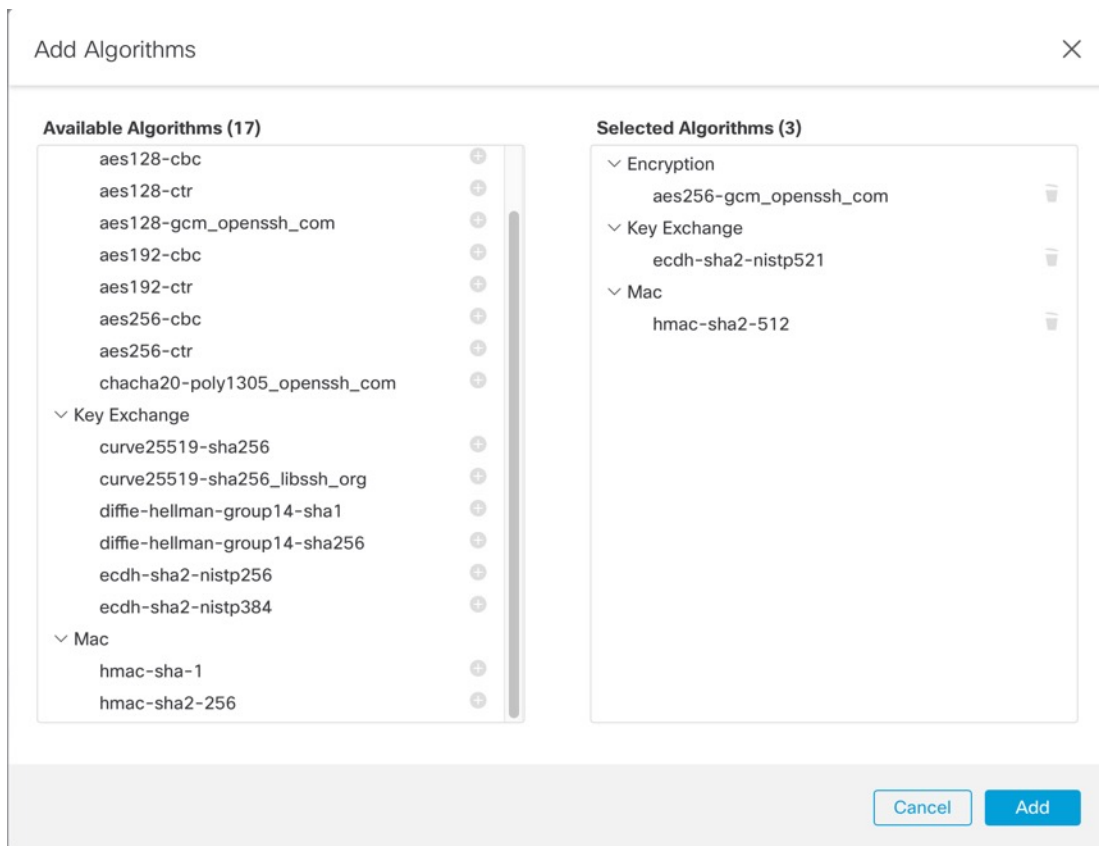
图 155: 添加算法
