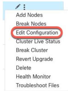
图 198: 编辑配置
