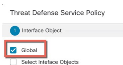
图 341: 全局策略
