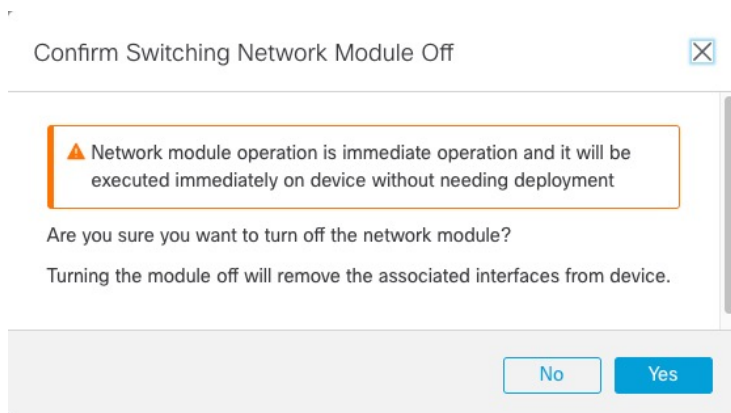
图 325: 确认禁用
