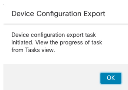
图 32: 确认导出
