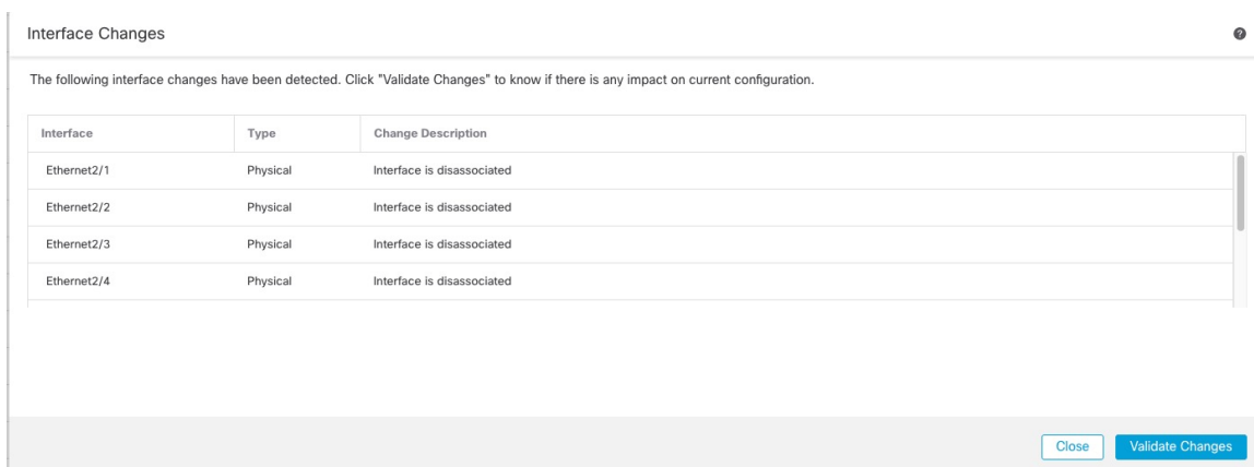
图 328: 接口更改
