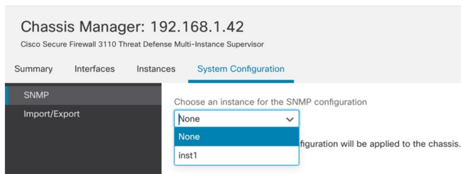
图 145: SNMP
