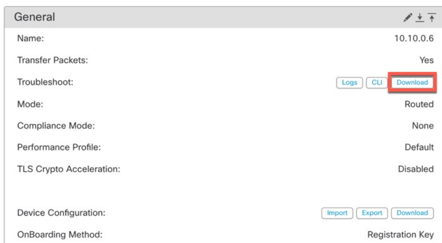
图 28: 下载
