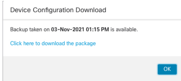
图 34: 下载软件包
