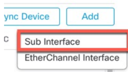
图 134: 添加子接口
