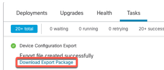
图 33: 导出任务
