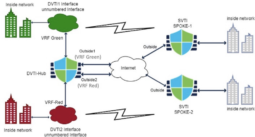
图 382: 具有多个虚拟路由器和动态 VTI 的站点间 VPN
