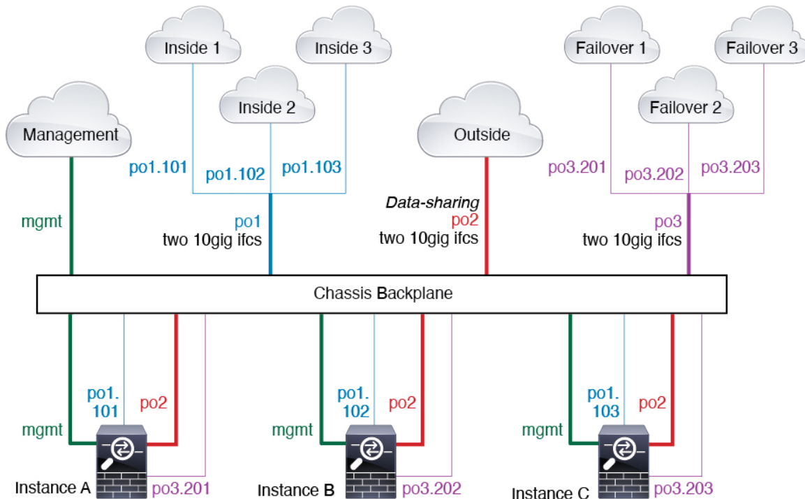
图 119: 典型多实例部署
