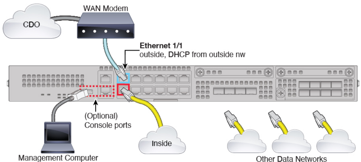
图 40: Firepower 2100 的布线
