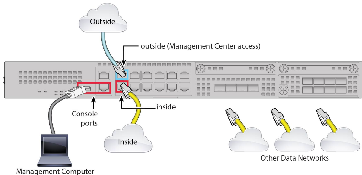
图 17: 远程管理部署的布线
