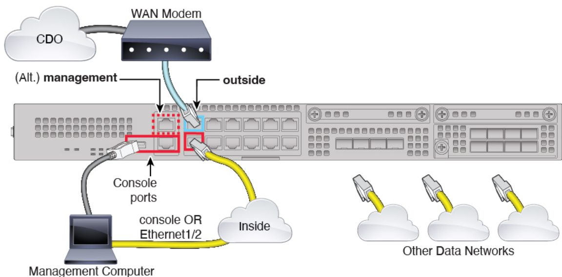
图 42: Firepower 2100 的布线
