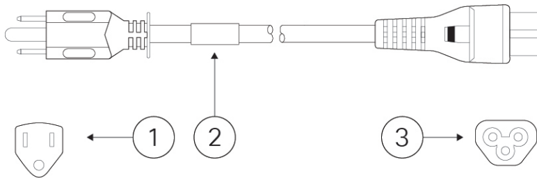
图 13: 加拿大 (CAB-AC-C5)
