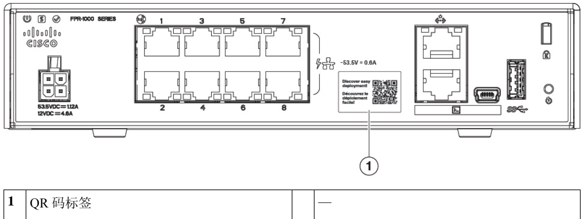
图 4: Firepower 1010 二维码标签
