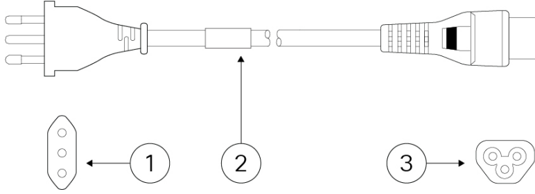
图 17: 意大利 (CAB-AC-C5-ITA)
