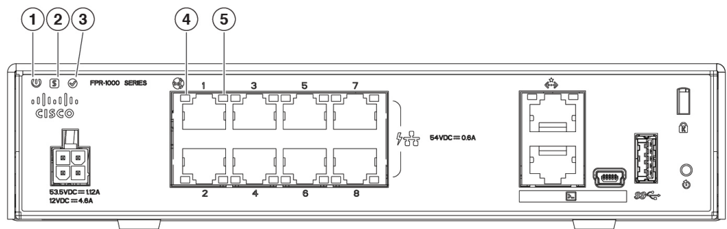
图 9: 后面板 LED
