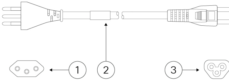
图 12: 巴西 (CAB-AC-C5-BRA)
