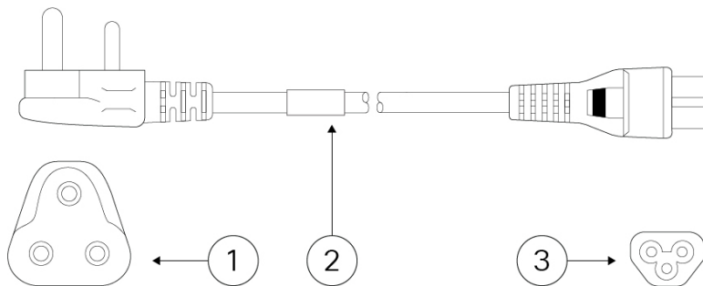
图 16: 印度 (CAB-AC-C5-IND)
