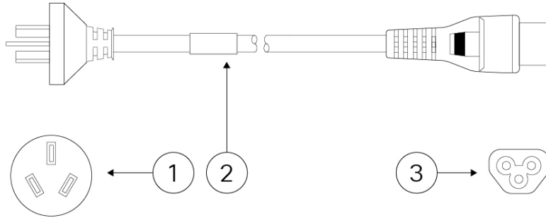
图 14: 中国 (CAB-AC-C5-CHI)
