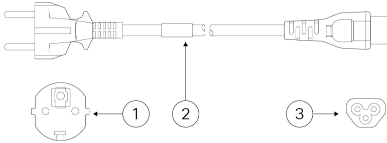
图 15: 欧洲 (CAB-AC-C5-EUR)
