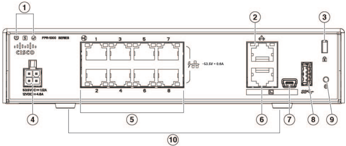
图 7: Firepower 1010 和 1010E 后面板
