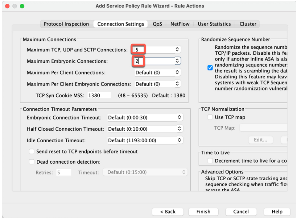
图 4: 规则操作
