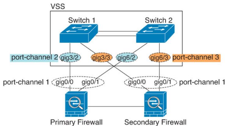
图 54: 主用/备用故障切换和 VSS/vPC
