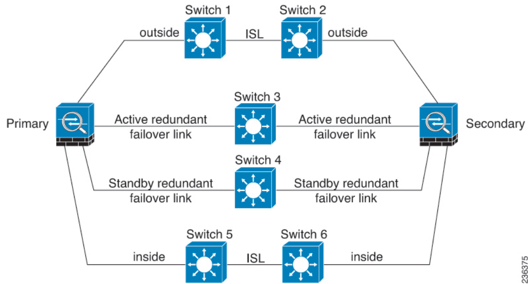
图 45: 使用交换机间链路连接
