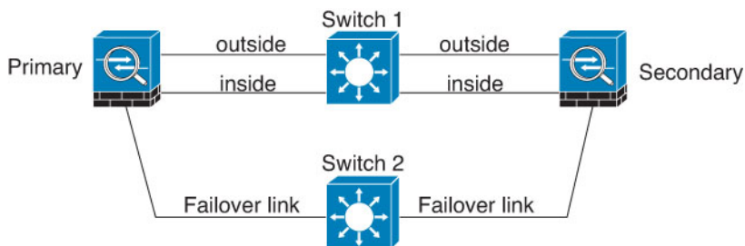
图 42: 通过缆线连接
