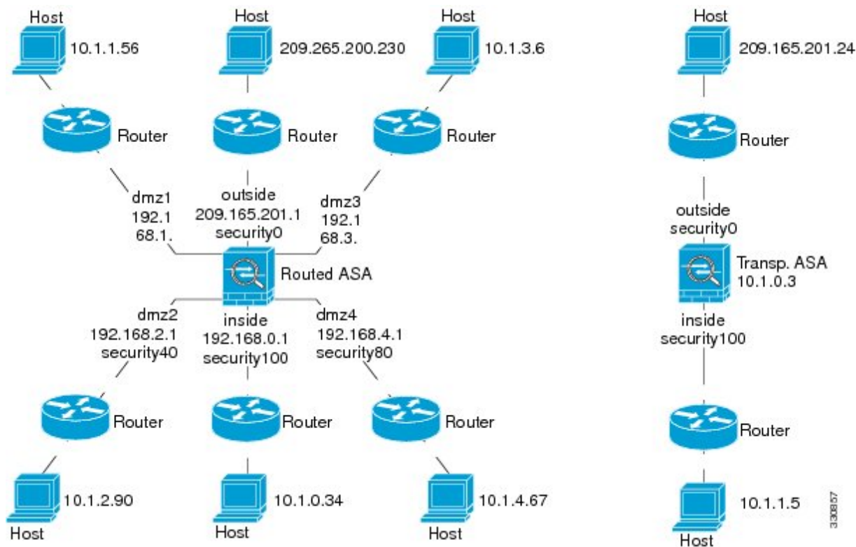
图 69: 接口、路由器和主机的网络图
