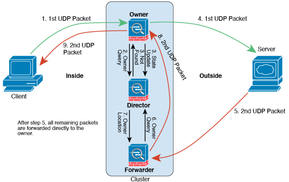
1. 图 50: ICMP 和 UDP 数据流
