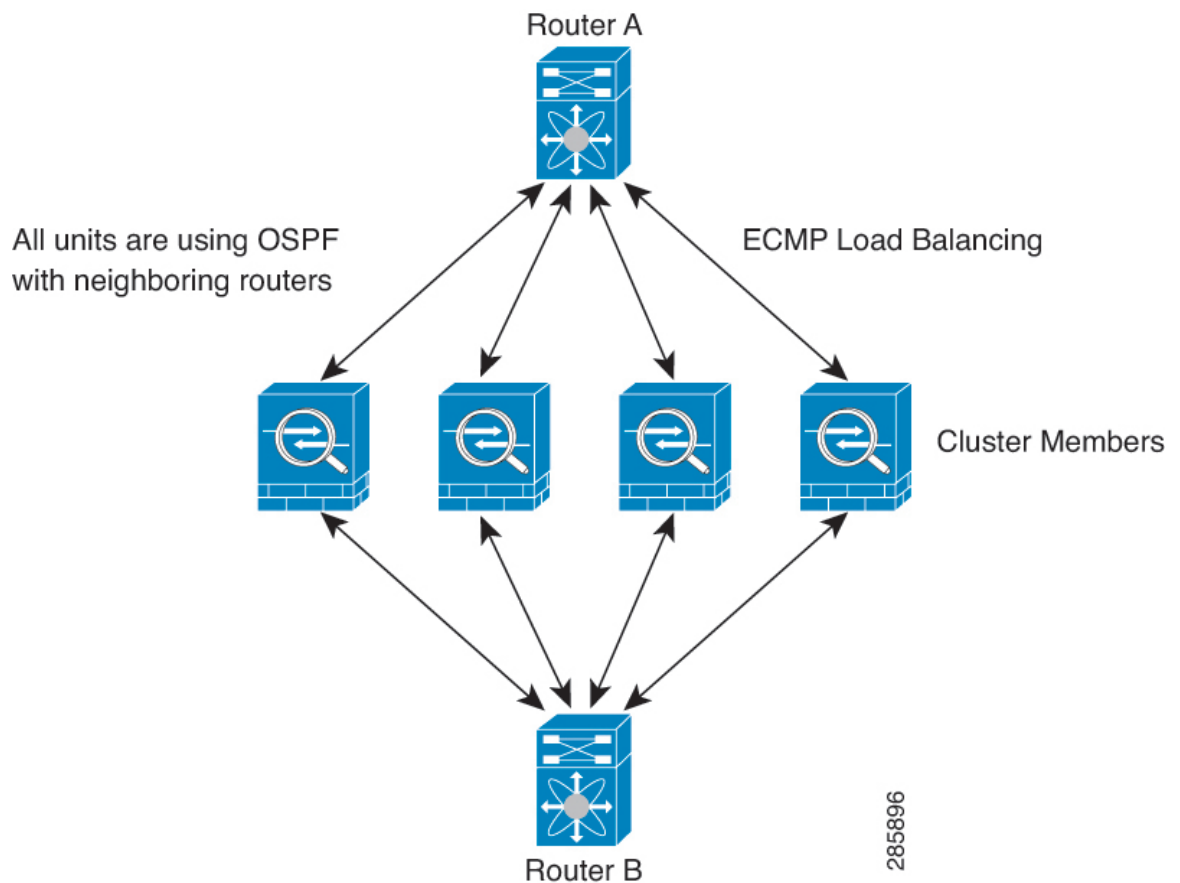
图 49: 独立接口模式下的动态路由
