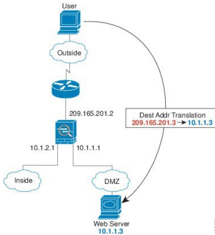
图 23: 外部到 DMZ
