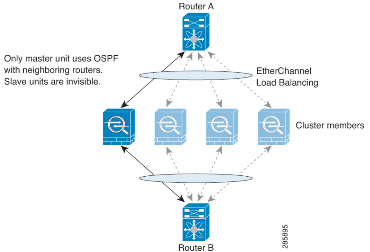
图 56: 跨区以太网通道模式下的动态路由
