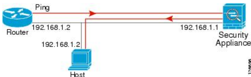
图 71: IP 寻址问题引发的 Ping 故障
