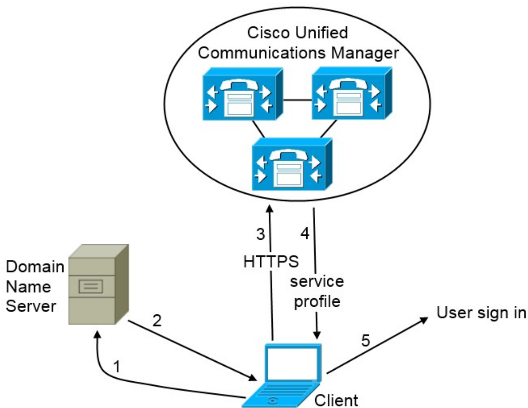
그림 8: UDS SRV 레코드 로그인 흐름
