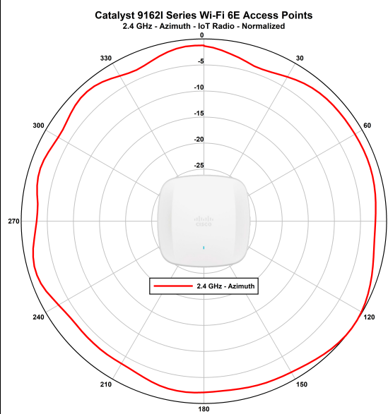
図 15: CW91621 - IoT アンテナ正規化放射パターン (2.4 GHz 水平)
