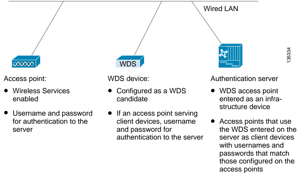
図 12-3 WDS に参加するデバイスの設定
