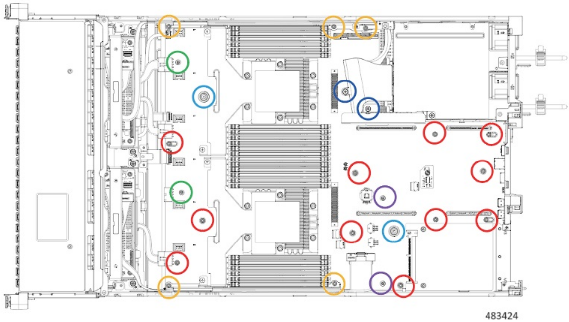
図 1: UCS C245 M8 Main PCBA を取り外すためのネジの位置
