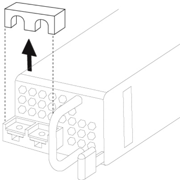
図 46: プラスチックカバーの取り外し
