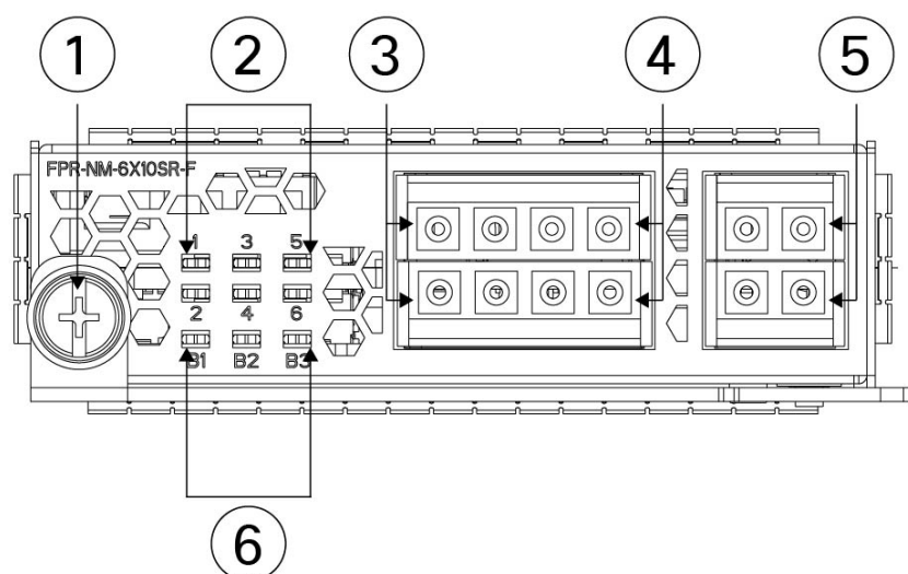
図 12: FPR4K-NM-6X1SX-F、FPR4K-NM-6X10SR-F、FPR4K-NM-6X10LR-F
