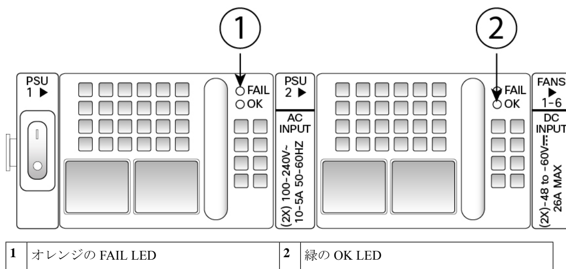
図 13: 電源モジュールの LED
