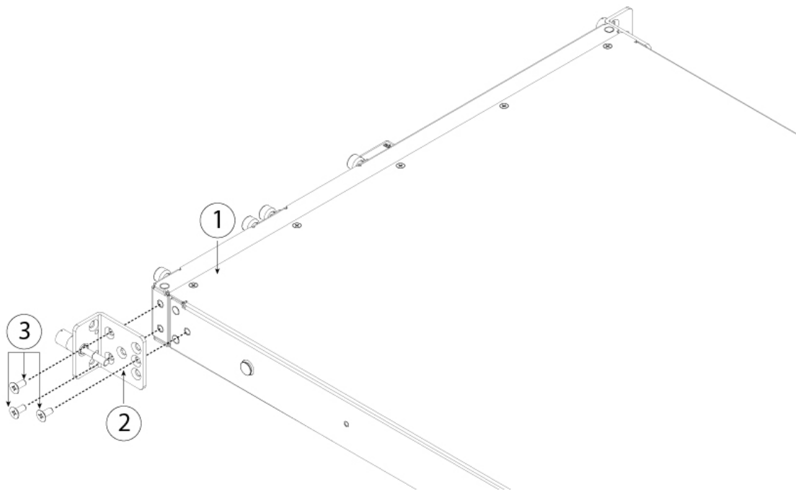
図 35: シャーシ側面へのラックマウント ブラケットの取り付け
