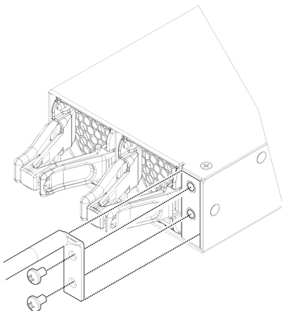
図 40: アース ラグの取り付け
