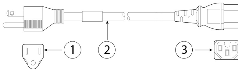
図 29: 北米 CAB-TA-NA
