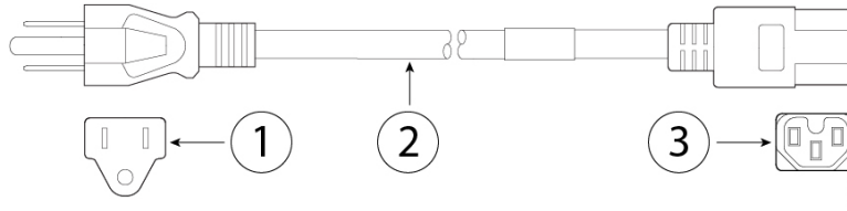
図 33: 台湾 CAB-9K10A-TWN
