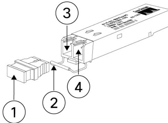
図 15: SFP
