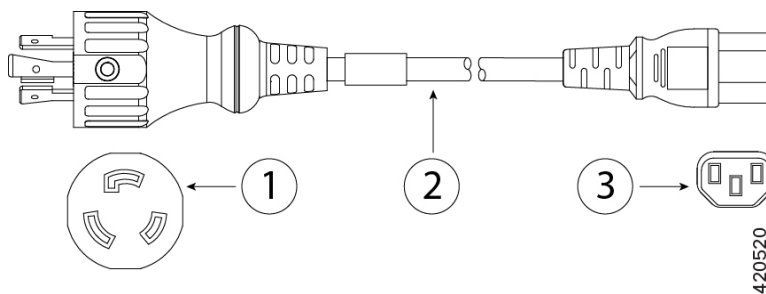
図 27: 日本 CAB-L620P-C13-JPN
