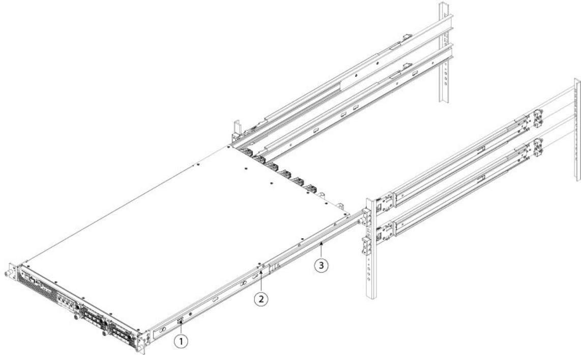
図 38: 内側レールのリリースクリップ
