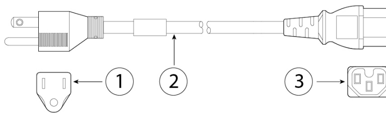
図 28: 日本 CAB-TA-JP
