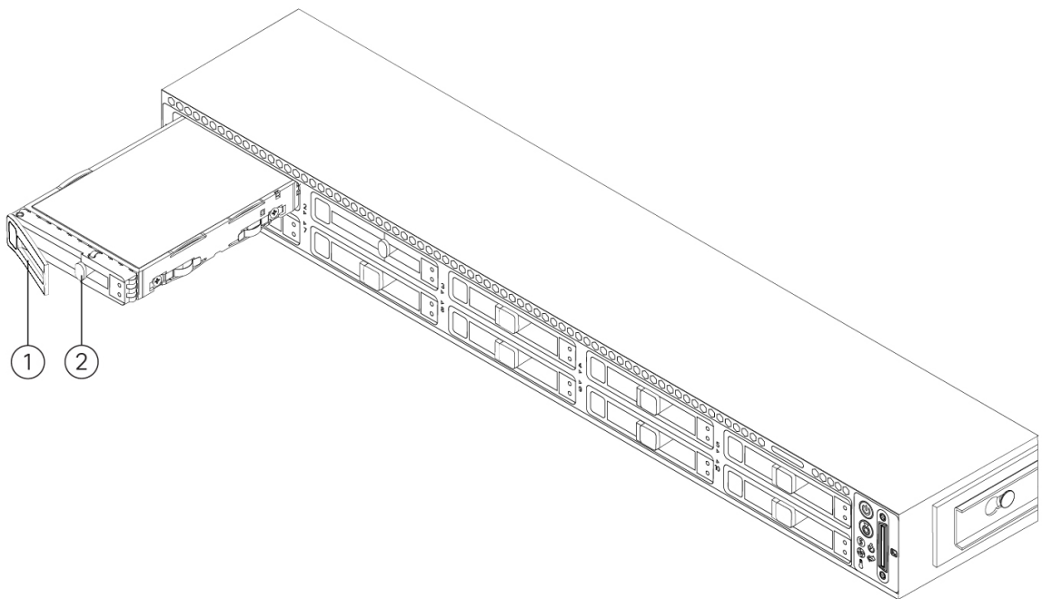
図 36: ドライブの取り外し
