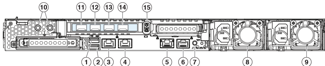
図 9: C395 および C695 の背面パネル
