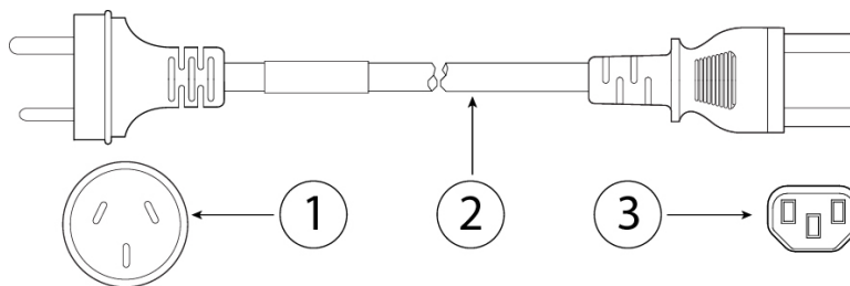
図 18: 中国 (CAB-250V-10A-CH)
