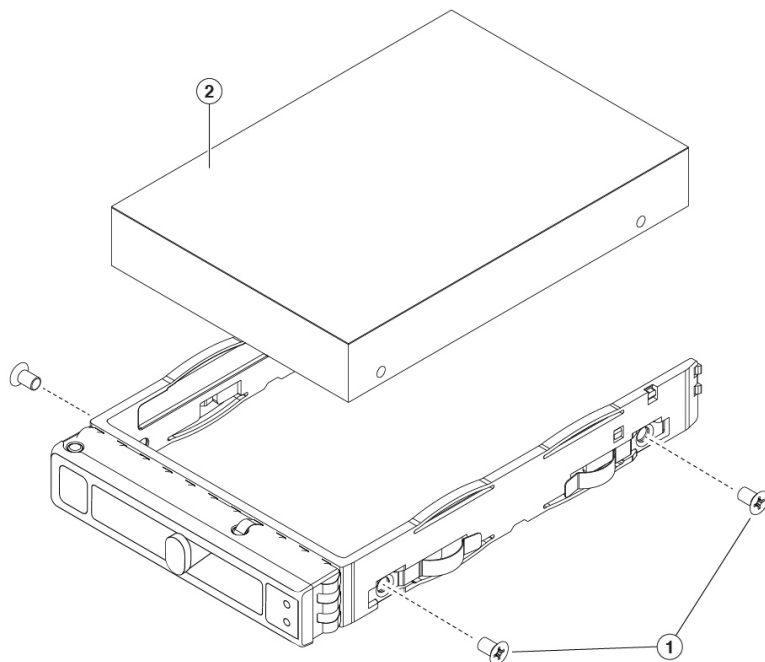
図 37: ドライブトレイの取り外し
