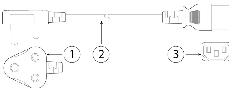
図 20: インド (CAB-250V-10A-ID)
