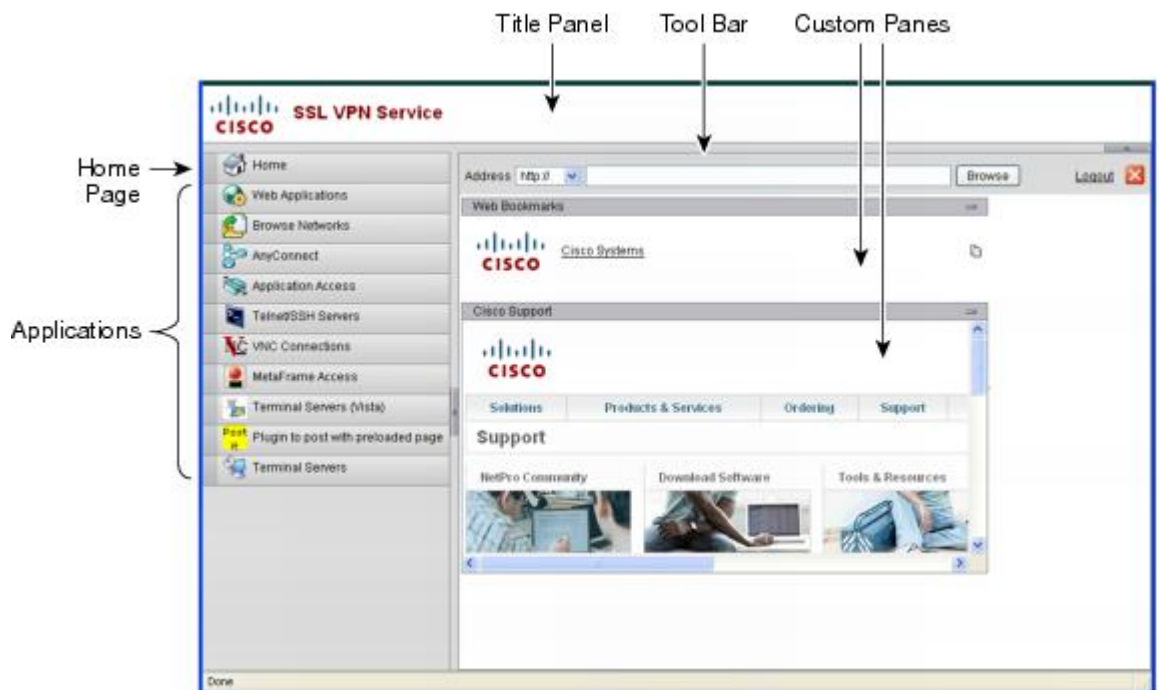
図 20: ポータル ページのカスタマイズ可能なコンポーネント
