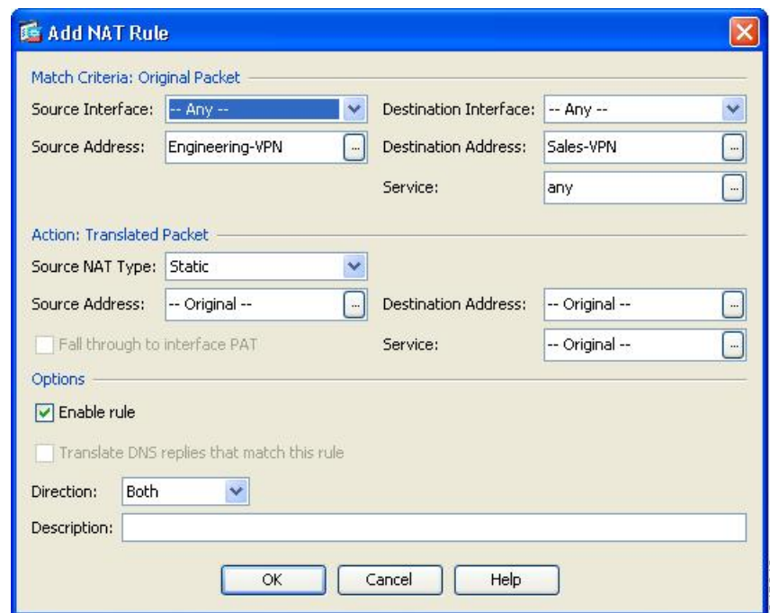
図 2: [Add NAT Rule] ダイアログ ボックス
