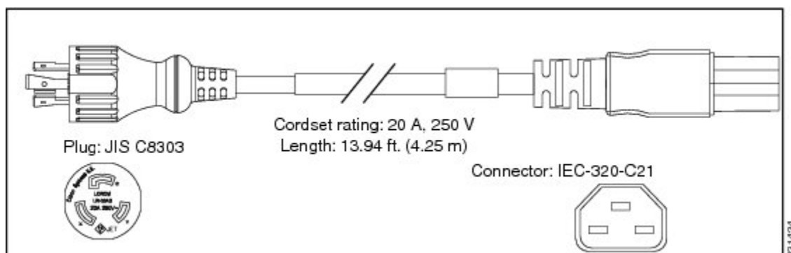
図 52: AC 電源コード PWR-CAB-AC-JPN=
