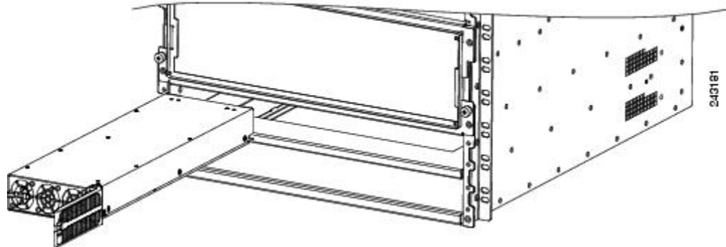
図 214:バージョン1 ACまたは DC電源モジュールの取り外しまたは取り付け
