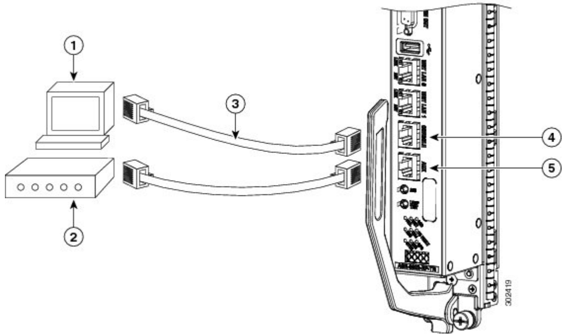
図 193: RP コンソール ポートおよび補助ポートの接続
