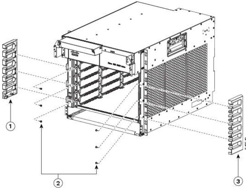
図 145: Cisco ASR 9010 ルータへのシャーシサイドブラケットの取り付け
