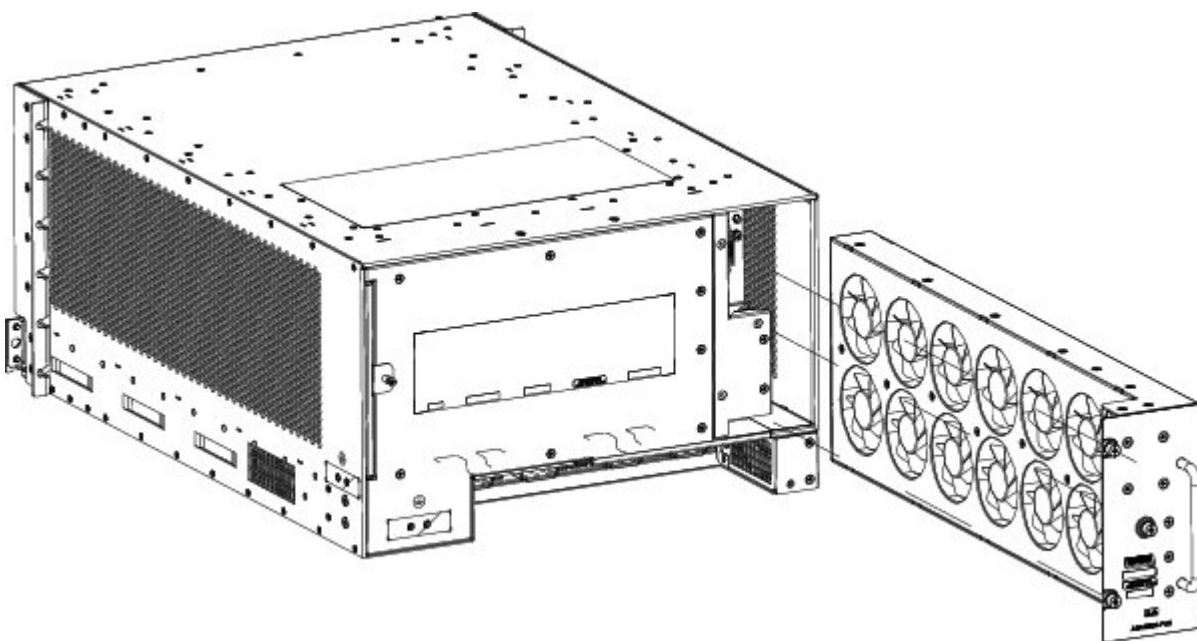
図 86: Cisco ASR 9904 ルータ シャーシでのファントレイの取り外し/取り付け
