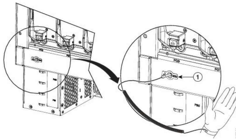
図 8: 静電気防止用リストストラップの Cisco ASR 9922 ルータシャーシへの接続
