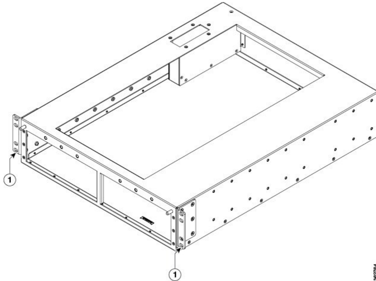
図 152: 事前に取り付けられた前面取り付けブラケット付きのプレナム
