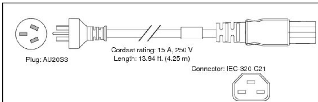
図 46: AC 電源コード PWR-CAB-AC-AUS=
