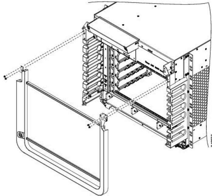
図 148: Cisco ASR 9006 ルータへのオプション アクセサリ扉の取り付け
