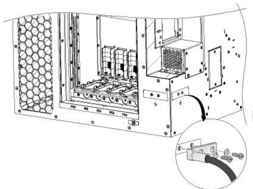
図 135: Cisco ASR 9906 ルータの NEBS ボンディングとアース
