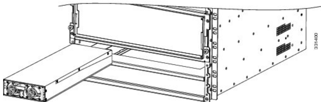
図 215:バージョン2またはバージョン3のACまたはDC電源モジュールの取り外し/取り付け
