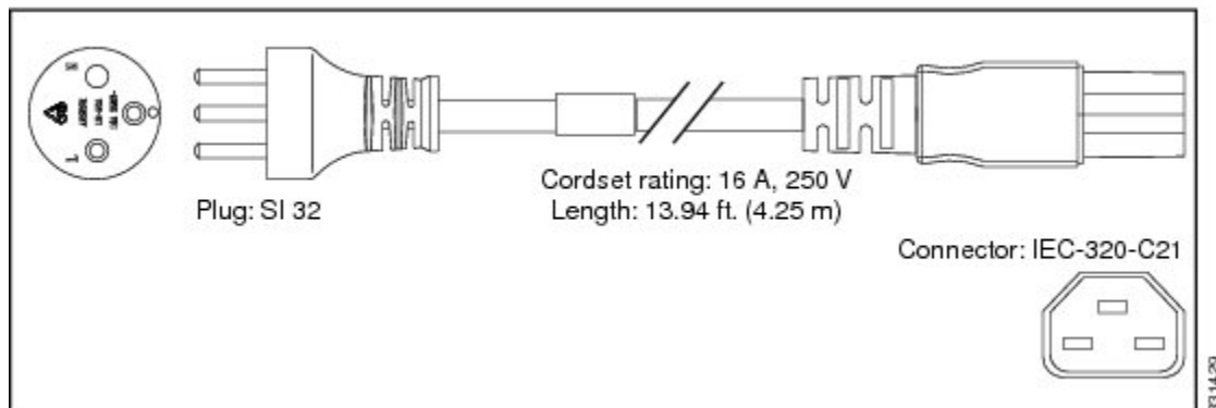
図 45: AC 電源コード PWR-CAB-AC-USA=
