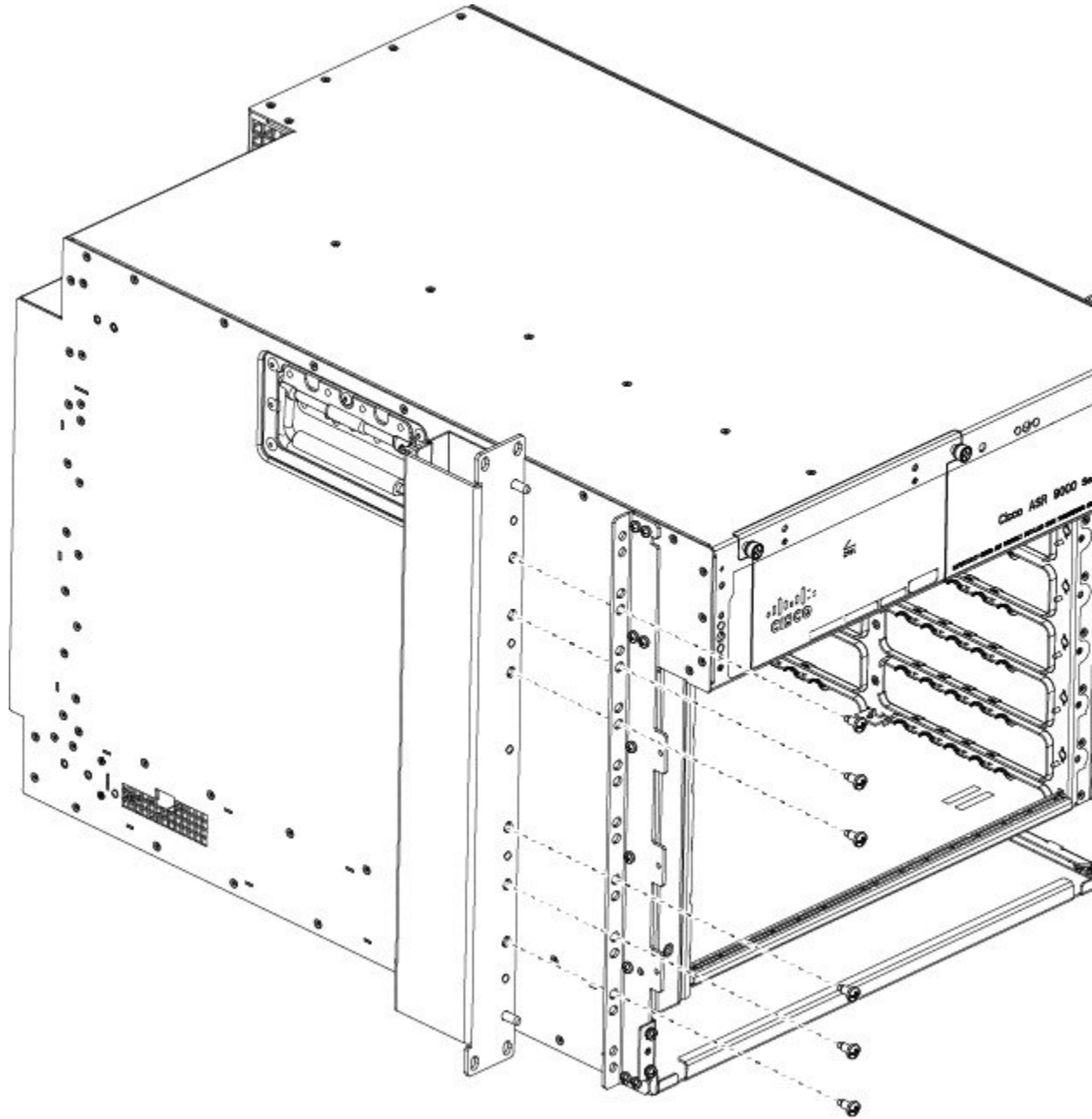
図 150: Cisco ASR 9006 ルータシャーシの左側へのサポートブラケットの取り付け
