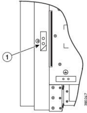
図 162: Cisco ASR 9904 ルータのジャケッティアース
