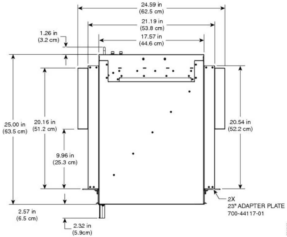
図 163: Cisco ASR 9904 ルータのエアージャケットの寸法: 上面図
