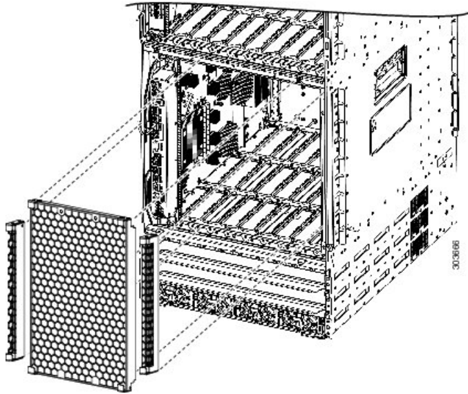
図 212: Cisco ASR 9922 ルータシャーシの中央のエア フィルタの取り外し : パージョン 1
