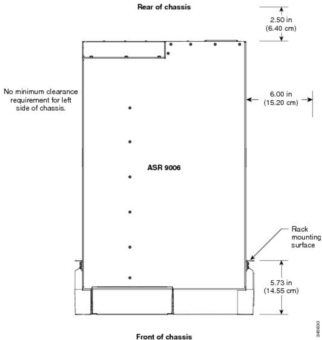
図 23:4 ポスト密閉型ラックに Cisco ASR 9006 ルータを取り付ける場合のスペース要件
