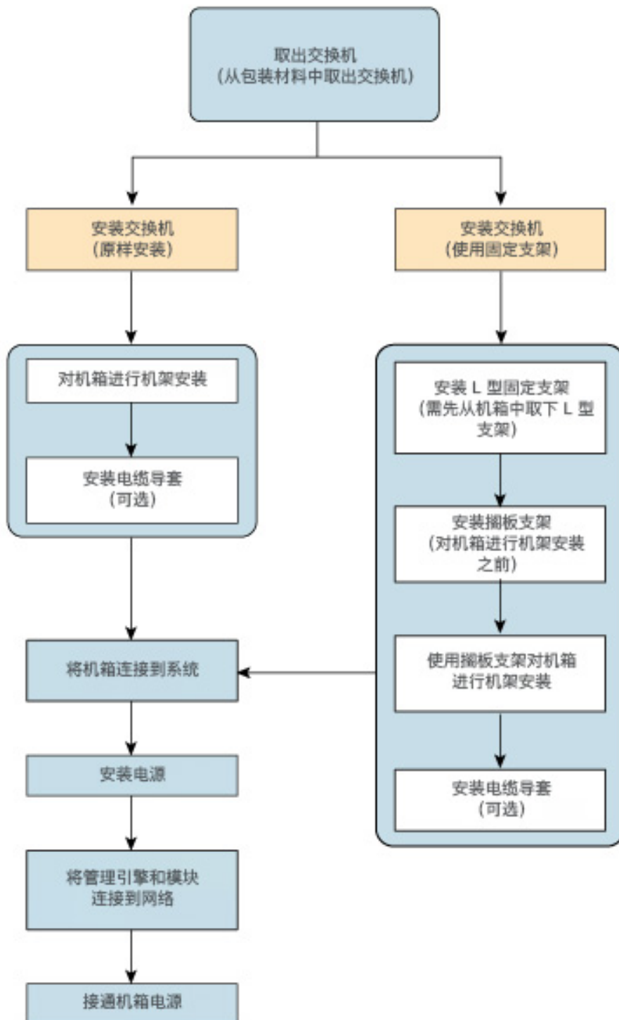
图 9: 安装任务
