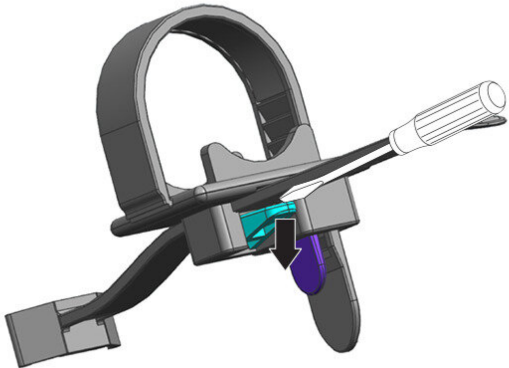
图 33: 带夹锁扣 - 细节
