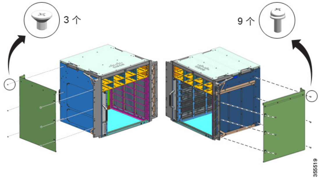
图 25: 安装墙盖
