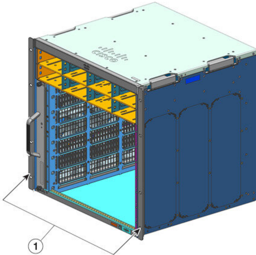
图 12: 机箱附带的 L 型支架
