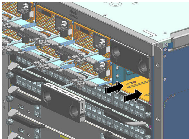
图 38: 已安装的电源空白盖板
