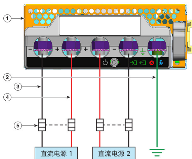
图 7: C9400-PWR-3200DC 安装示例：不同的直流电源
