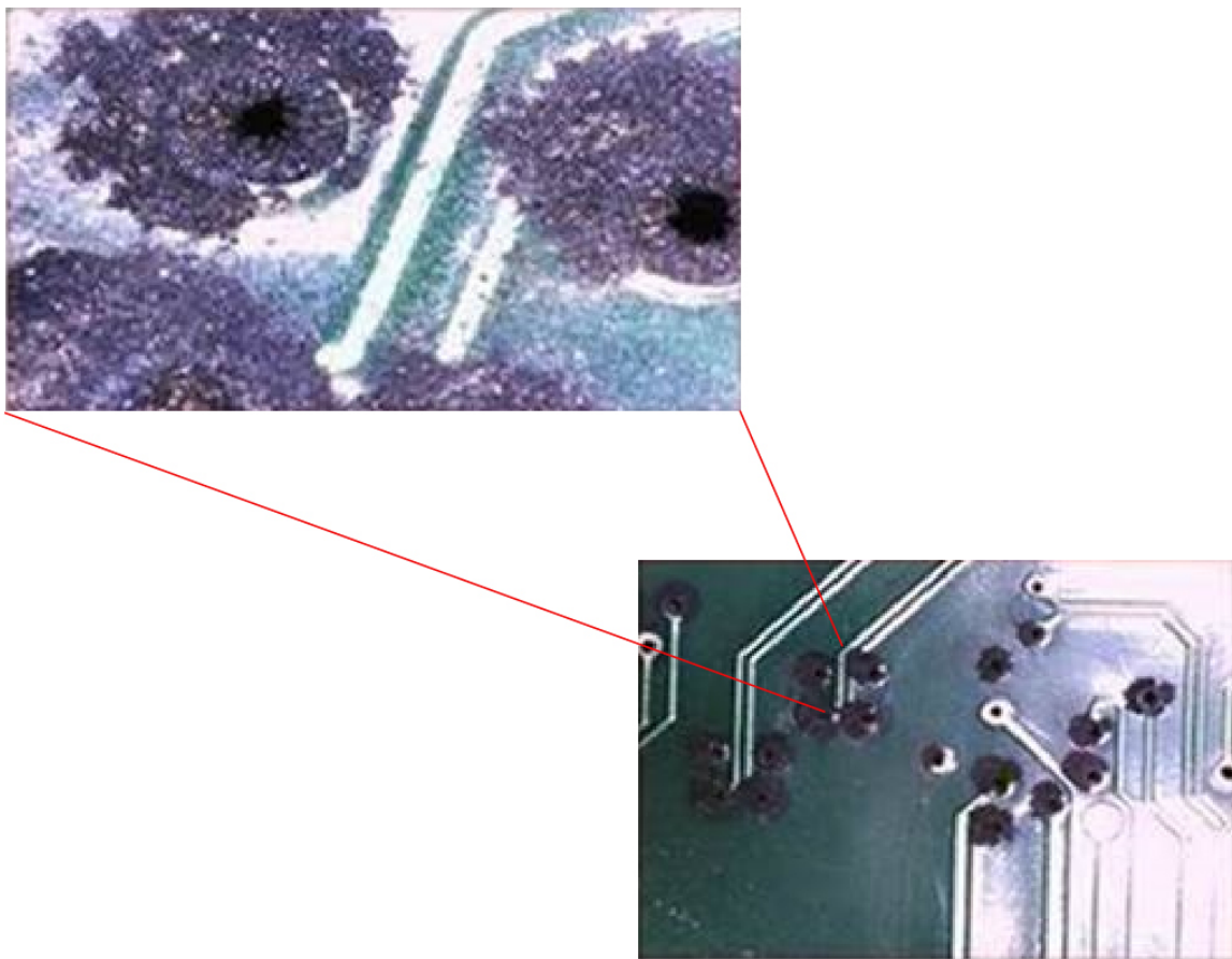
图 6: 金属触点发生腐蚀的 PCB
