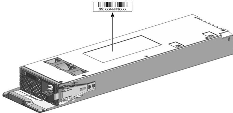
图 42: 电源模块序列号位置
