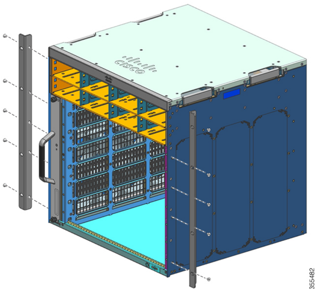
图 22: 卸下安装吊耳
