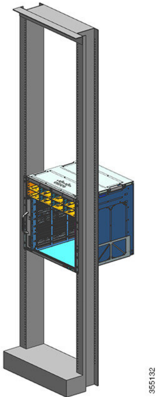
图 21: 机箱已固定到机架立柱上
