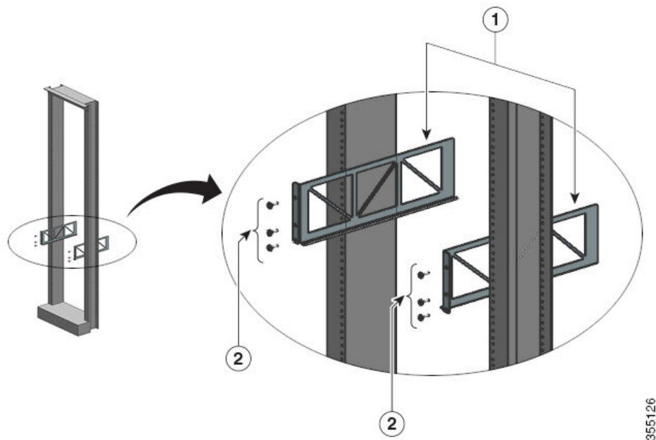
图 16: 安装搁板支架
