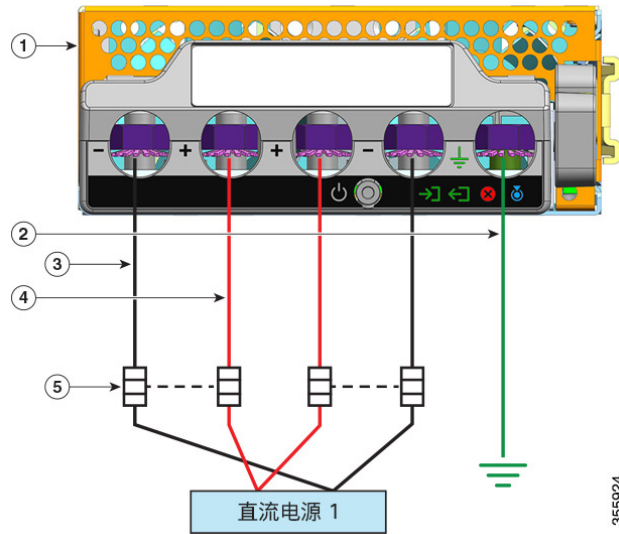
图 8: C9400-PWR-3200DC 安装示例 - 单个直流电源
