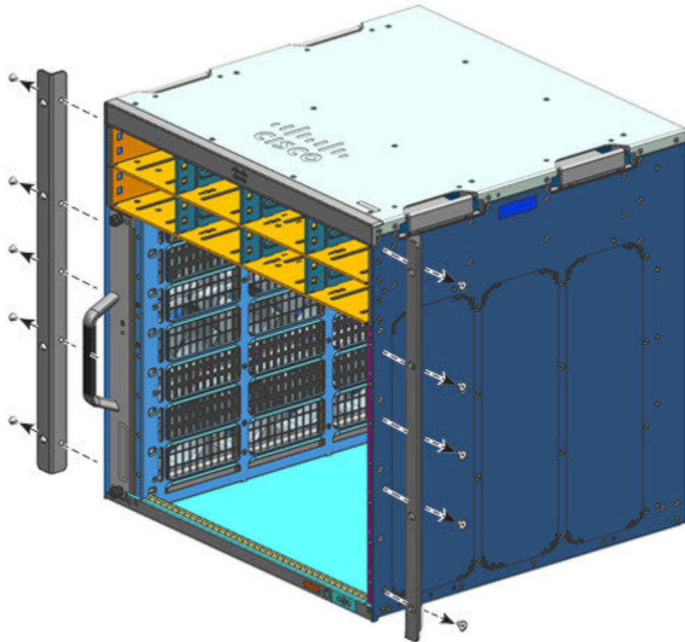
图 13: 卸下机箱附带的 L 型支架
