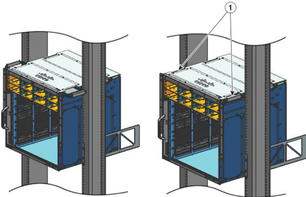
图 19: 将机箱向内滑动 - 第 2 部分
