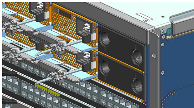
图 38: 已安装的电源空白盖板
