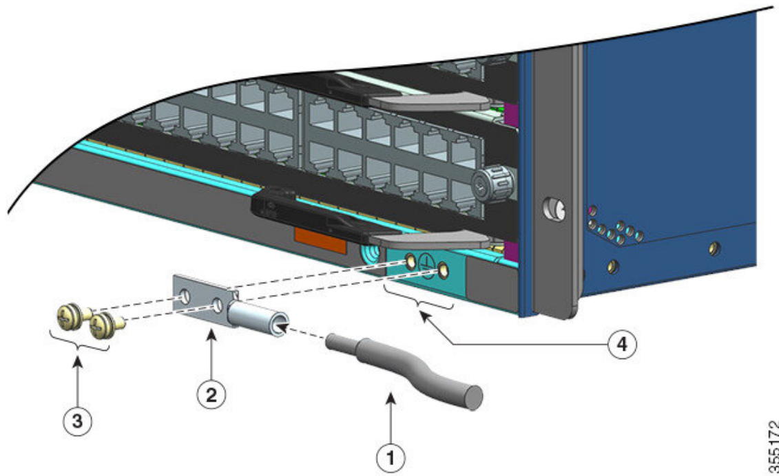
图 29: 定位和连接系统接地
