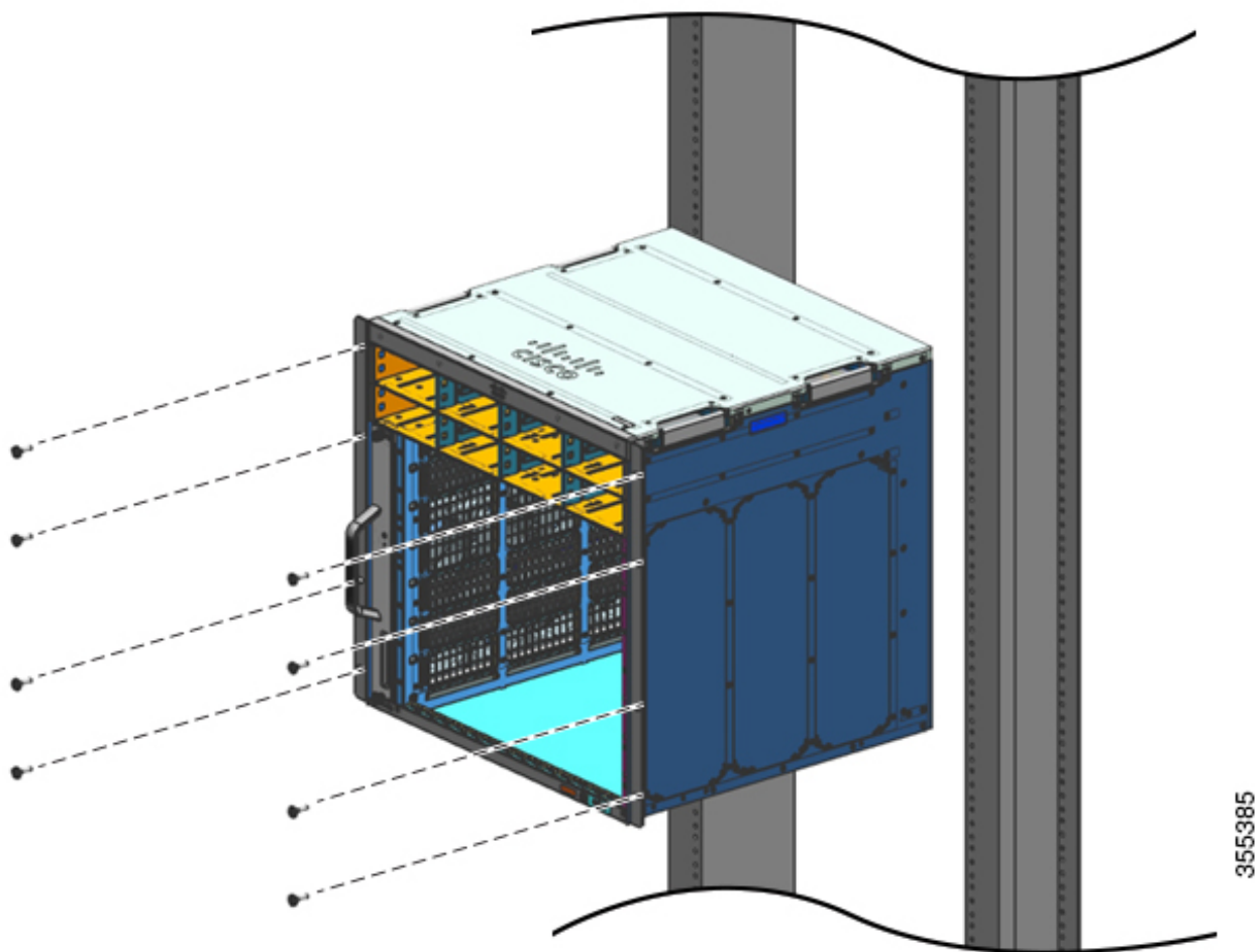
图 10: 将机箱固定到机架立柱上
