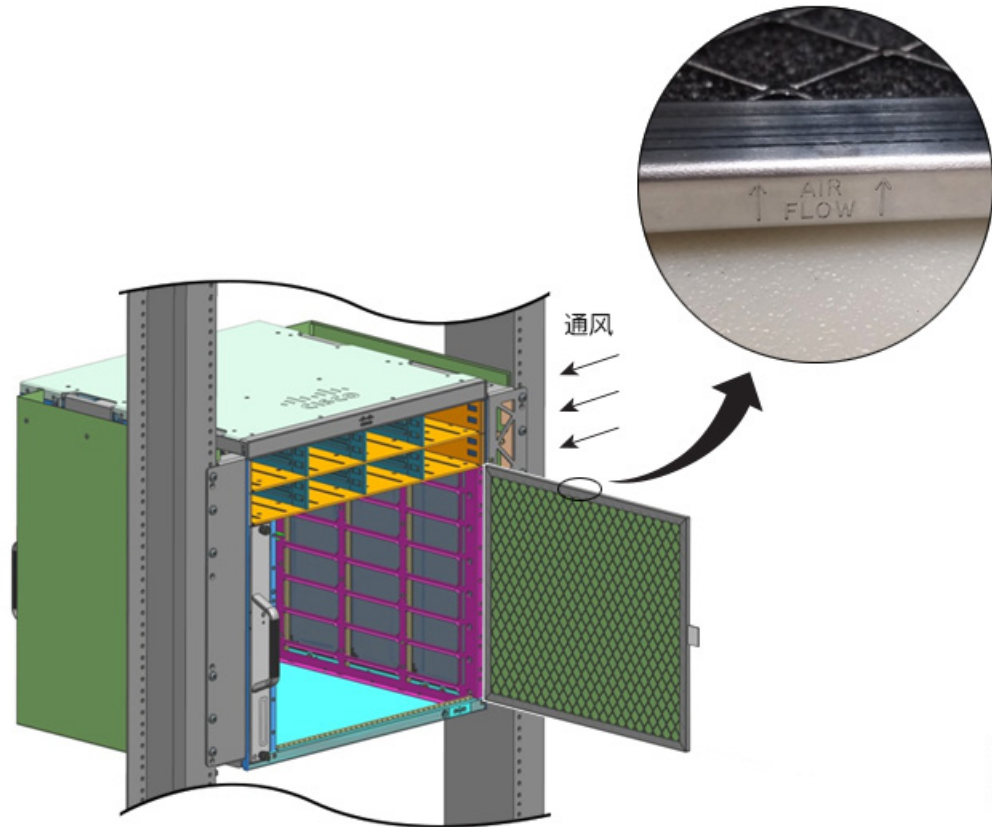
图 27: 符合 NEBS 标准的空气过滤器
