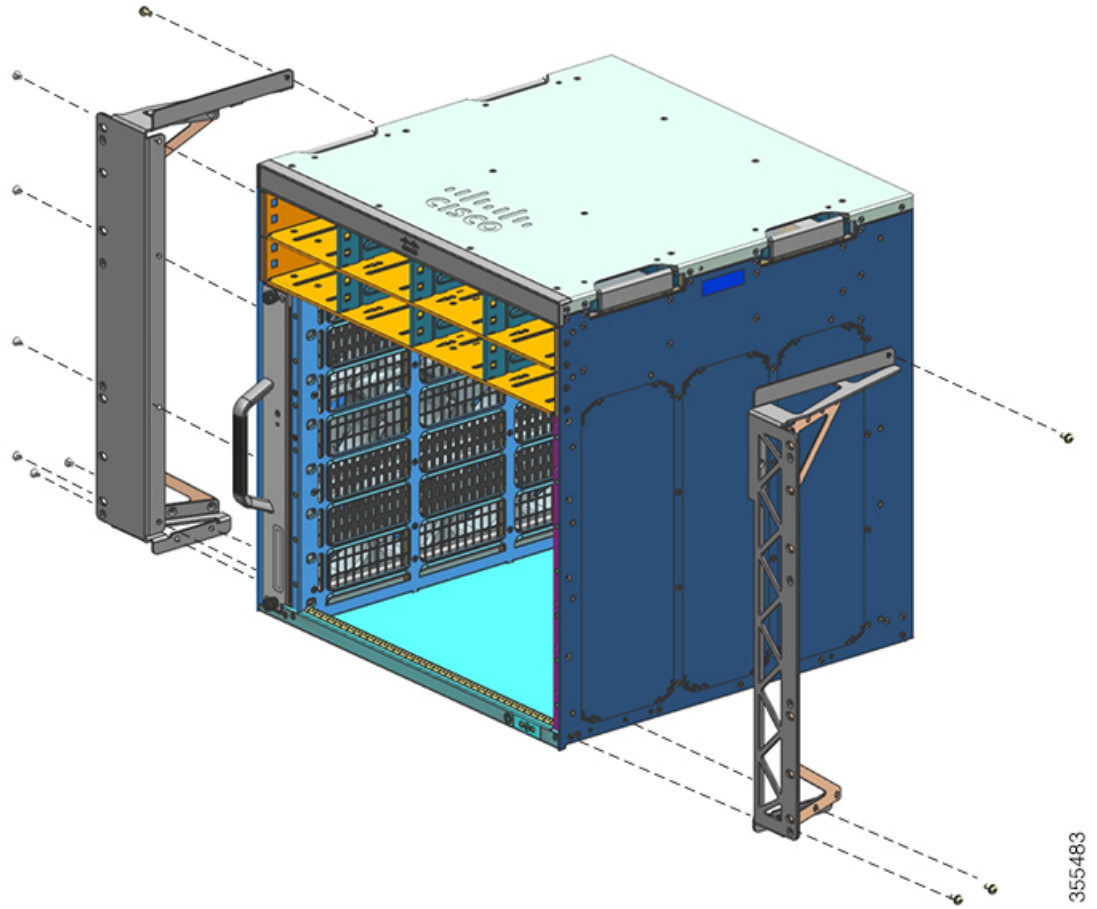
图 23: 安装机架耳架
