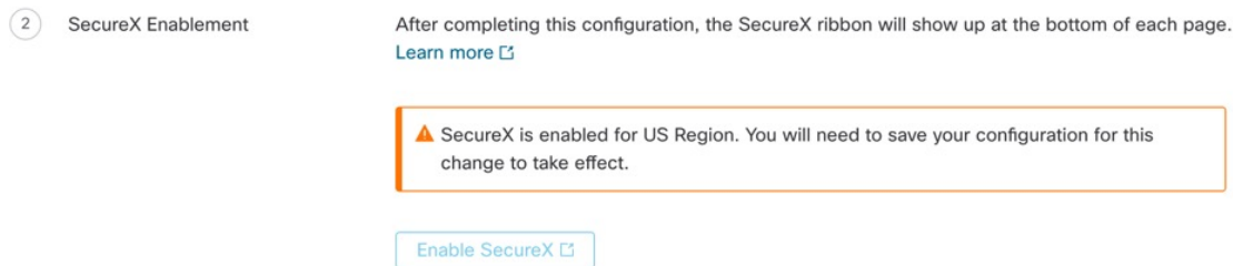
图 4: 成功消息
