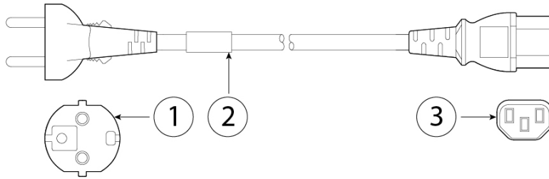
图 20: 欧洲 (CAB-ACE)
