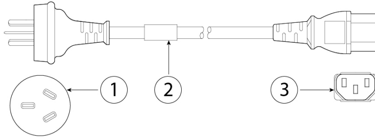
图 19: 中国 (CAB-ACC)
