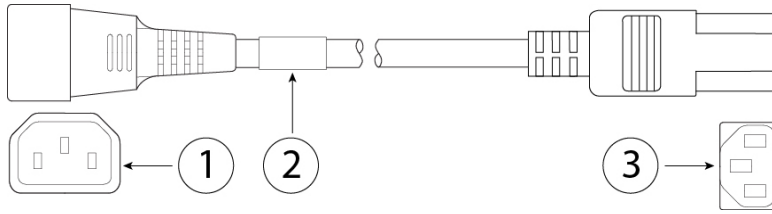
图 29: 跳线 (CAB-C13-C14-2M)
