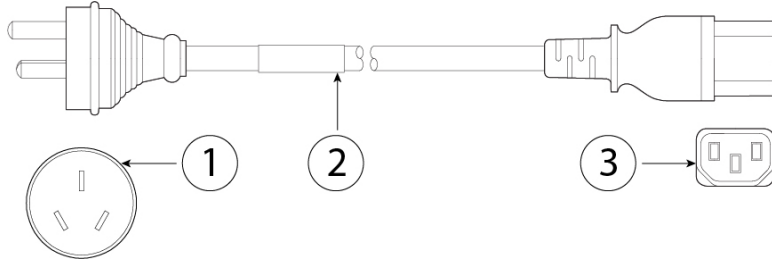
图 16: 阿根廷 (CAB-ACR)
