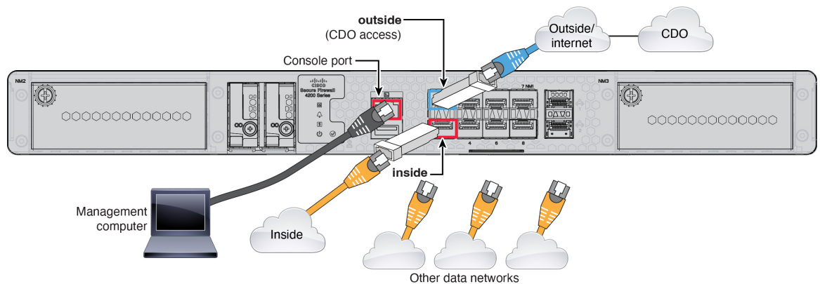
图 4: 布线 Cisco Secure Firewall 4200
