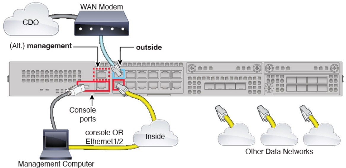
图 10: Firepower 2100 的布线
