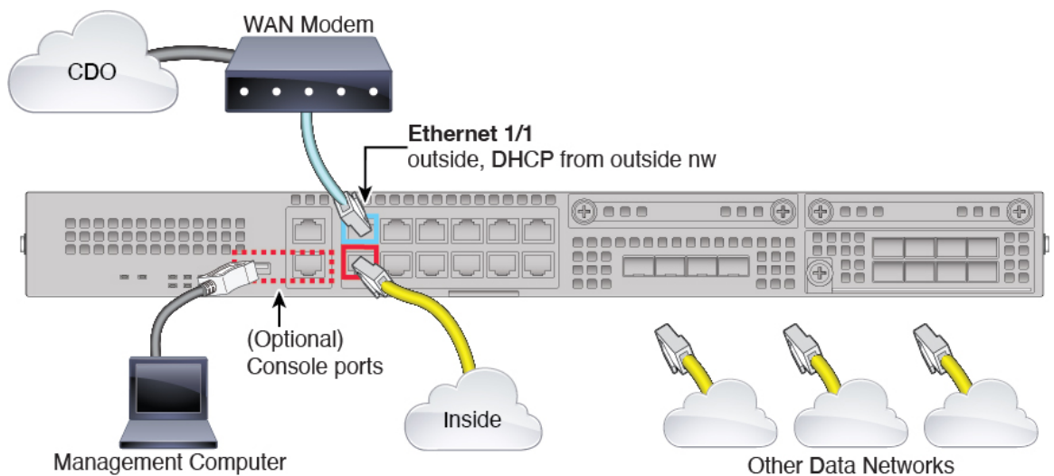
图 8: Firepower 2100 的布线
