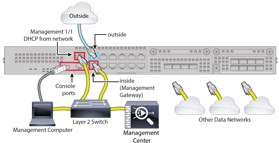
图 4: 进行边缘部署布线
