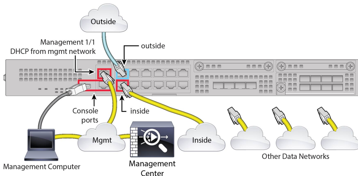
图 3: 连接单独管理网络的电缆
