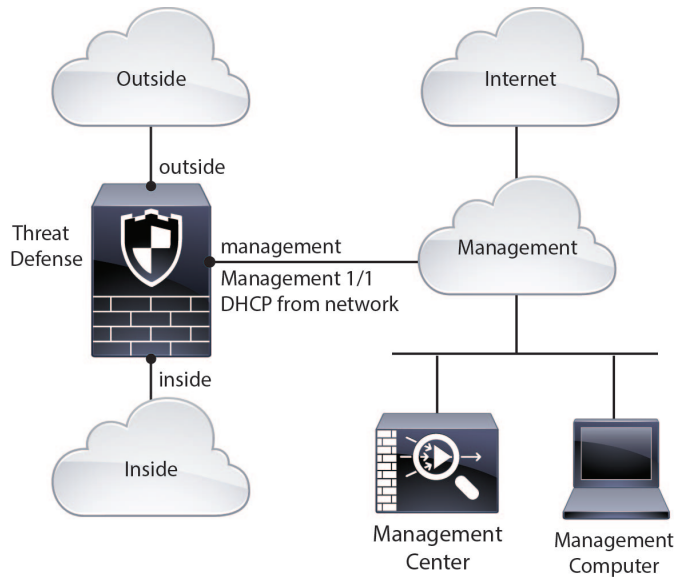
图 1: 单独的管理网络
