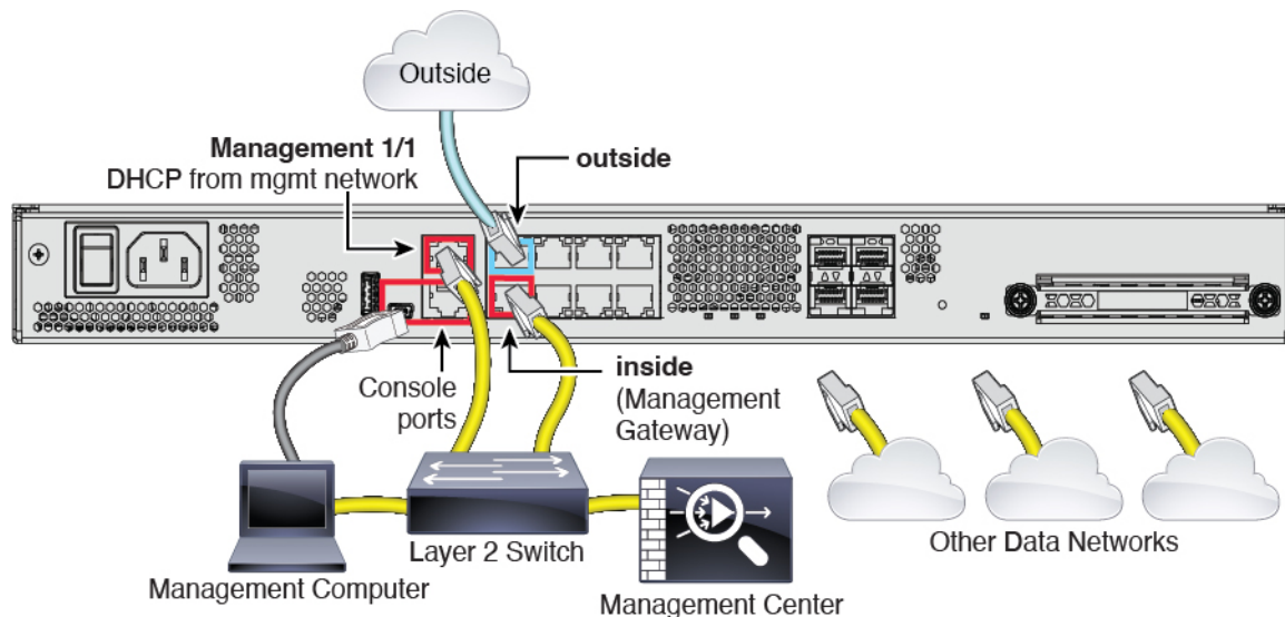
图 4: 进行边缘部署布线
