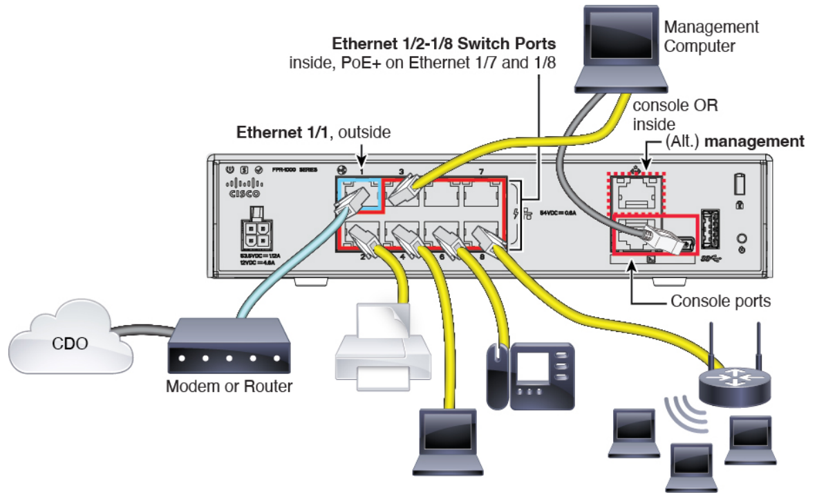
图 10: Firepower 1010 的布线
