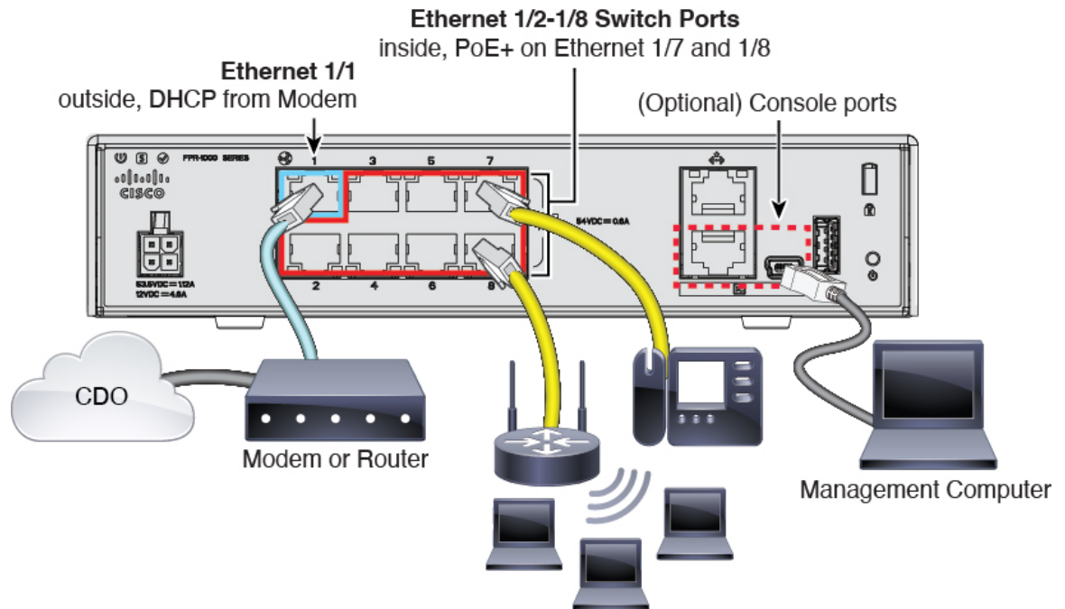
图 8: Firepower 1010 的布线
