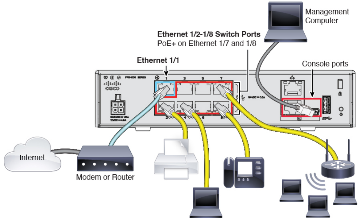
图 18: 远程管理部署的布线
