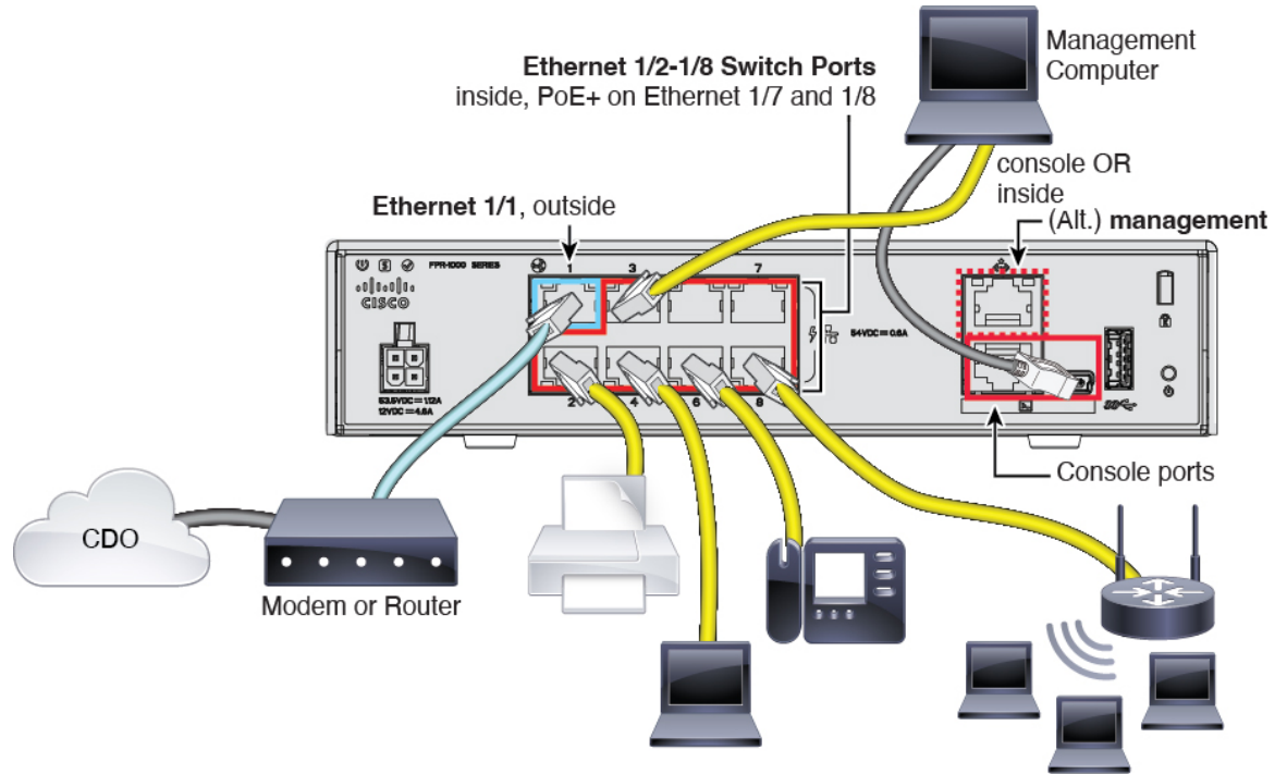
图 44: Firepower 1010 的布线
