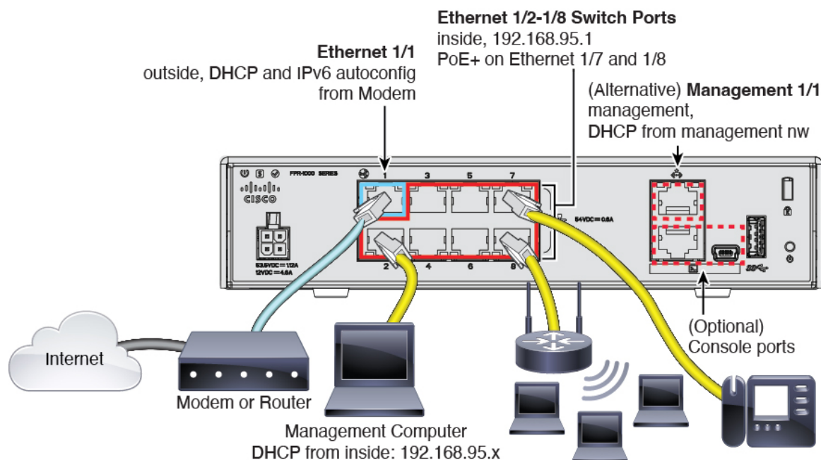
图 26: Firepower 1010 的布线
