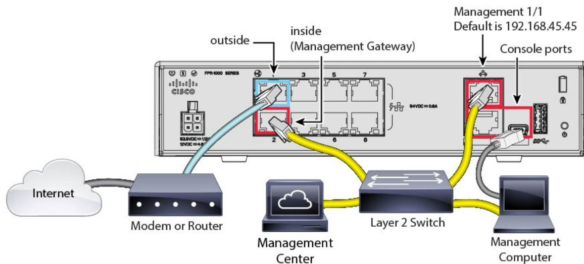
图 4. Firepower 1010 的布线
