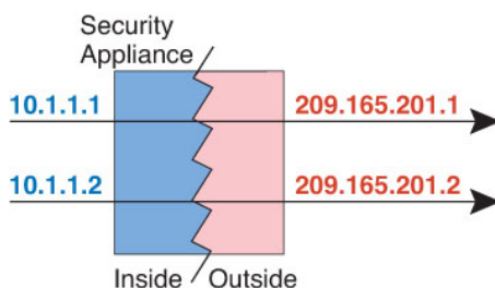
图 3: 动态 NAT
