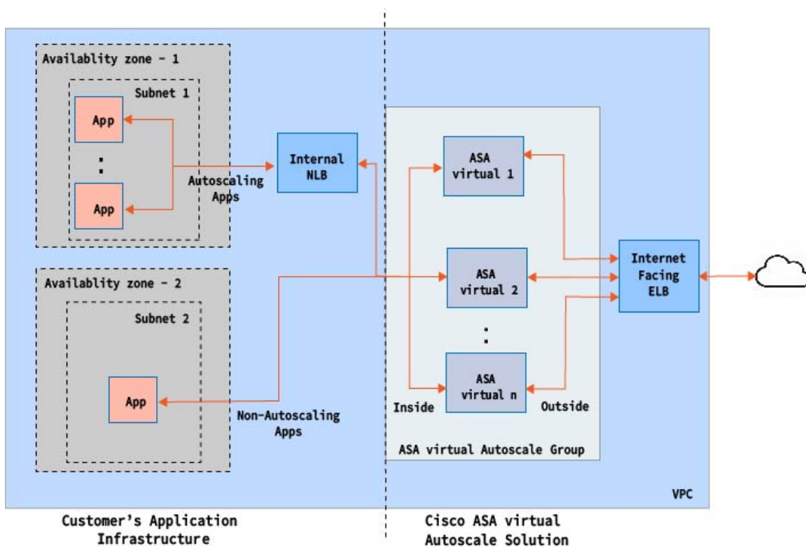
图 1: ASA 虚拟 Auto Scale 使用案例图
