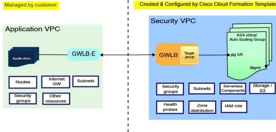
图 2: ASA 虚拟 AWS GWLB Auto Scale 使用案例图
