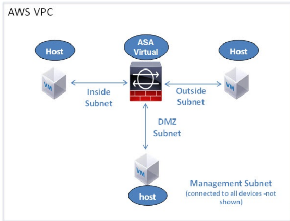
图 1: AWS 上的 ASA 虚拟部署示例
