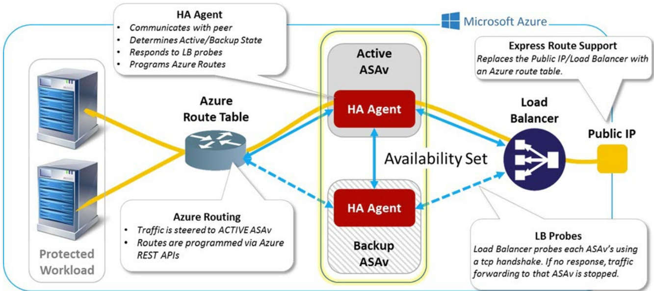
图 1: Azure 中的 ASAv 高可用性部署
