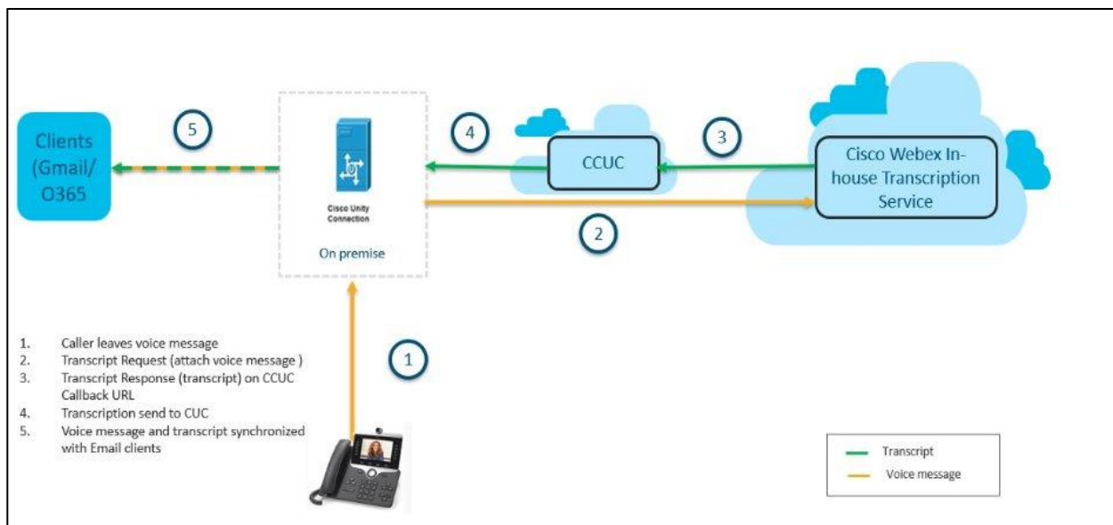
图1. 数据流图
