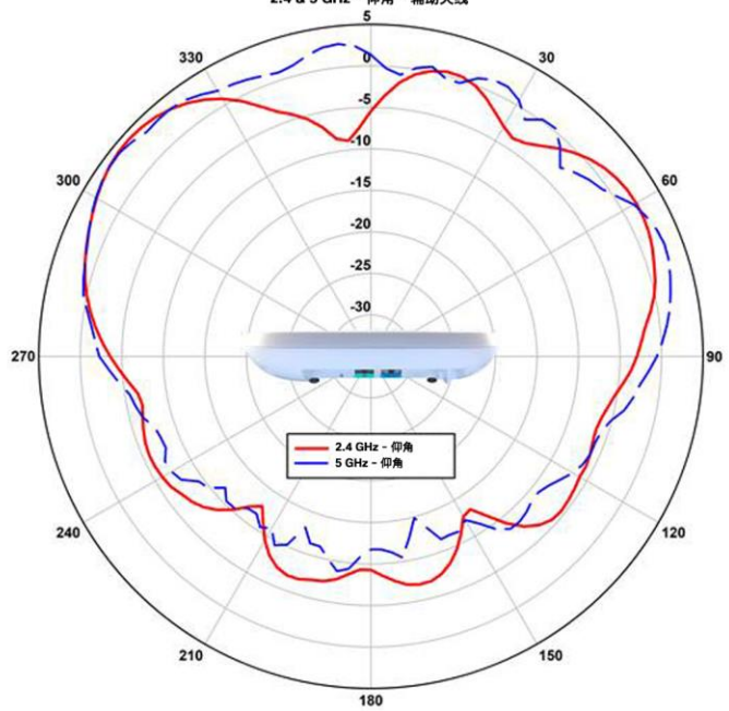
思科 C9130AXI 天线方向图 2.4 & 5 GHz - 仰角 - 辅助天线
