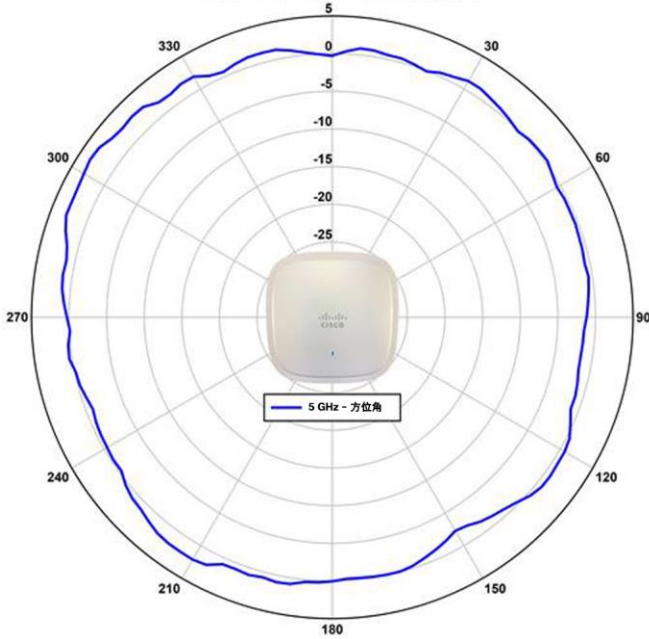
思科 C9130AXI 天线方向图 5 GHz - 方位角 - 双频天线元件
