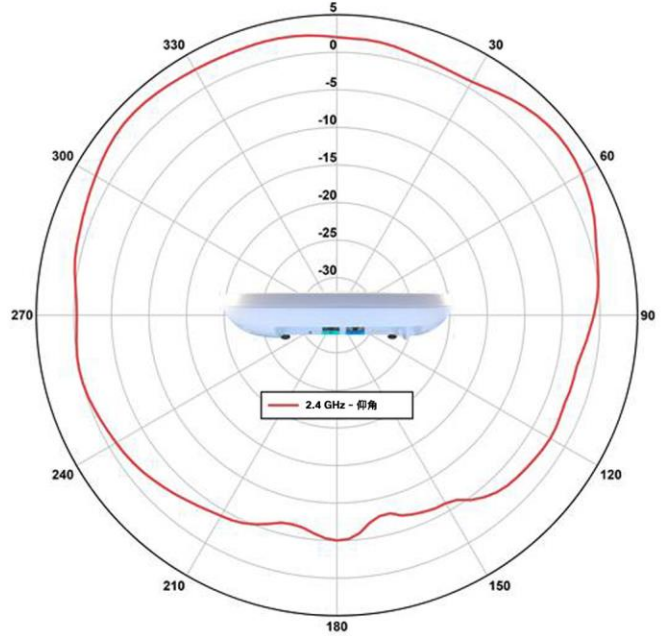
思科 C9130AXI 天线方向图 2.4 GHz - 仰角 - 双频天线元件
