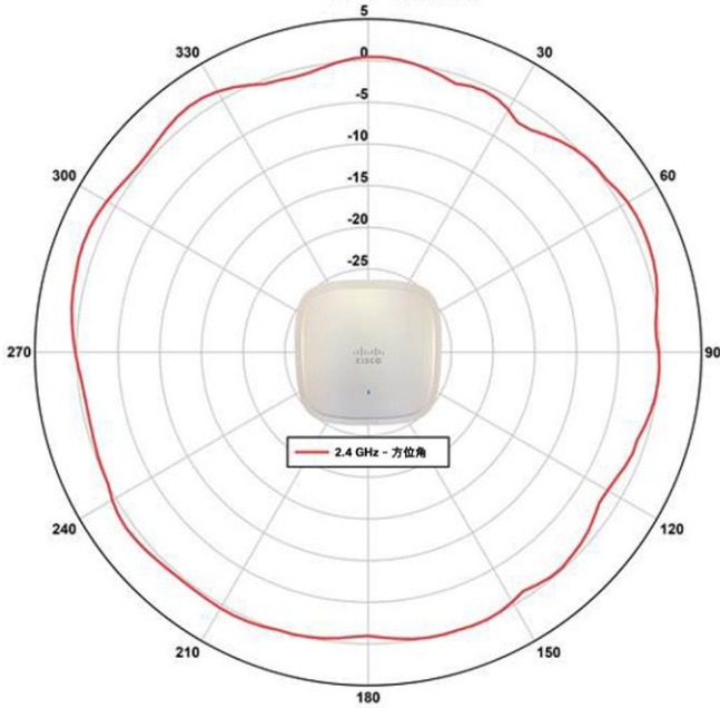
思科 C9130AXI 天线方向图 2.4 GHz - 方位角 - 双频天线元件
