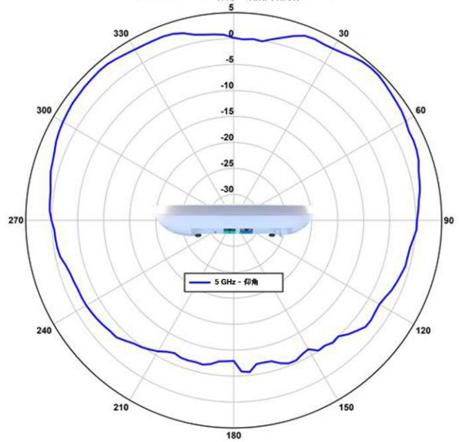
思科 C9130AXI 天线方向图 5 GHz - 仰角 - 双频天线元件
