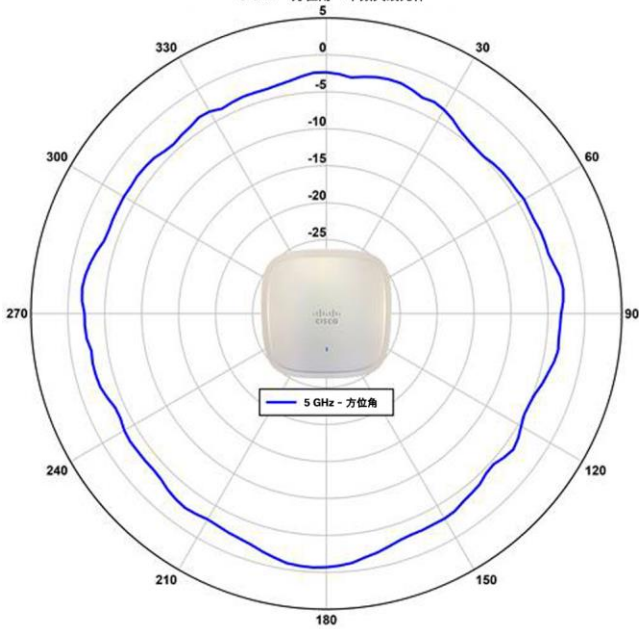
思科 C9130AXI 天线方向图 5 GHz - 方位角 - 单频天线元件
