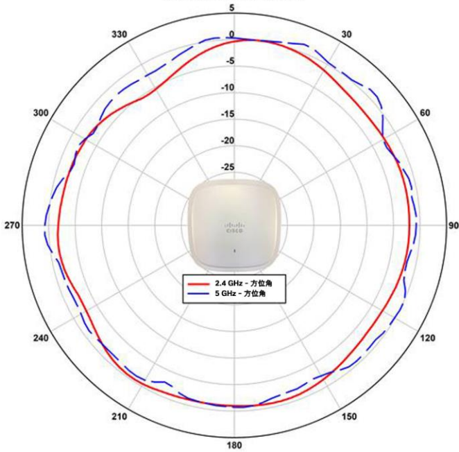
思科 C9130AXI 天线方向图 2.4 和 5 GHz - 方位角 - 辅助天线
