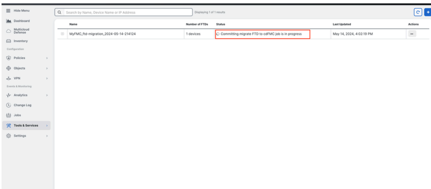
Afbeelding 15. Wijzigingen doorvoeren.
