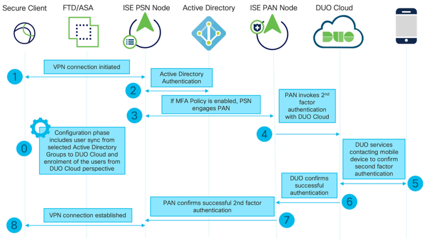
Stroomdiagram
