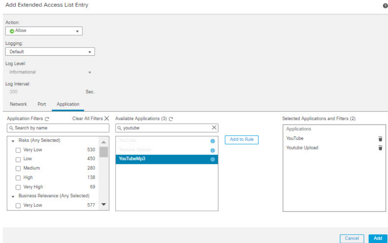
그림 2: Applications (애플리케이션) 탭
