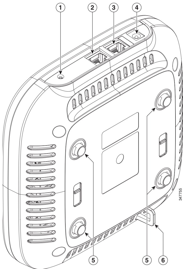
図 2 アクセスポイントのポートと接続 (底面)
