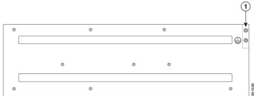
図 62: ルータの背面へのアース ラグの取り付け
