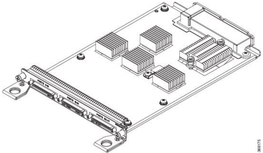
図 30: 48ポート T1/E1 の前面プレート
