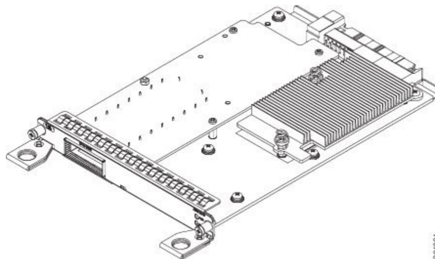
図 23: 1ポート 100ギガビットイーサネットインターフェイス モジュール
