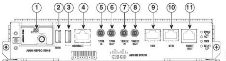
図 15: Cisco A900-RSP3C-200-S インターフェイス
