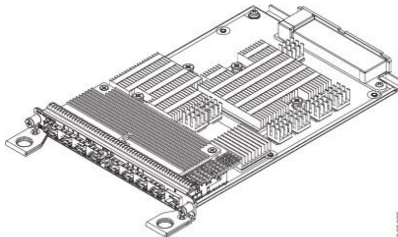
図 35: OC-192 インターフェイス モジュール
