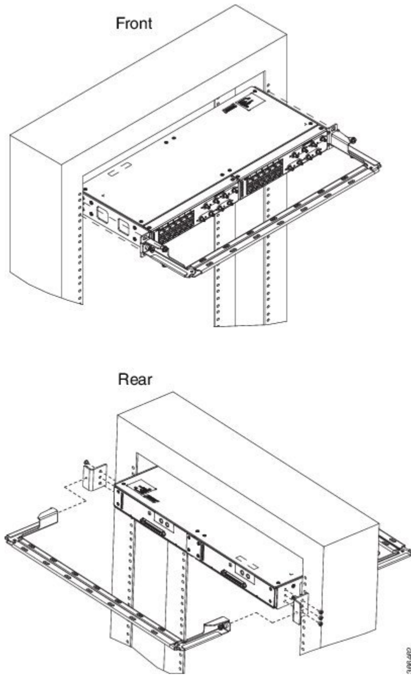
図 95: ラック (デュアル) への 19 インチ ブラケットの取り付け
