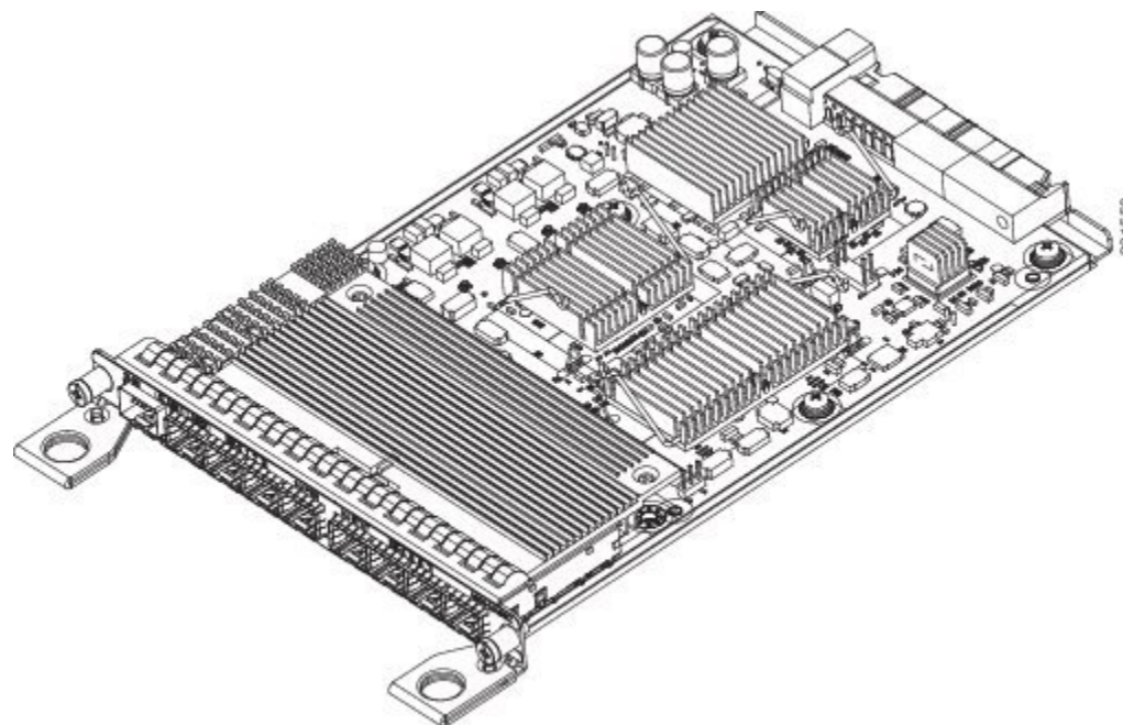
図 20: 8ポート 1 GE SFP + 1ポート 10 GE SFP+ インターフェイスモジュール
