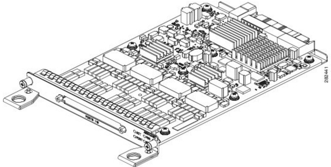
図 26: 16ポート T1/E1 インターフェイス モジュール
