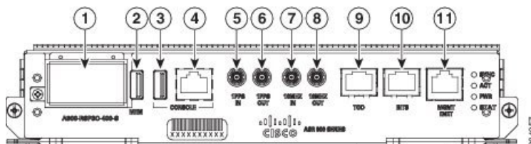
図 14: Cisco A900-RSP3C-400-S インターフェイス
