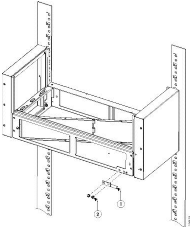
図 56: アース ラグ付きアース線の取り付け
