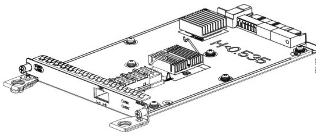
図 18: 1ポート10ギガビットイーサネットXFPインターフェイスモジュール
