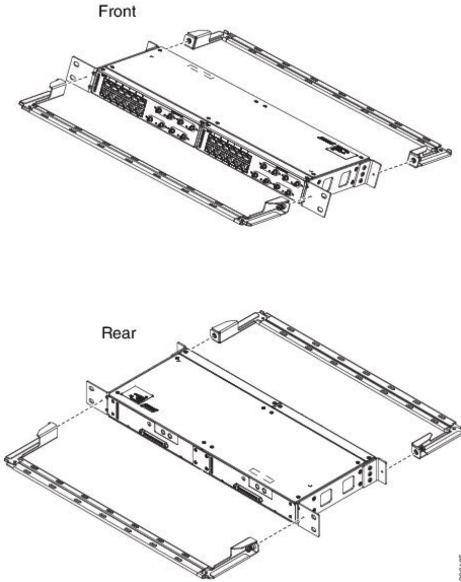
図 98: パッチパネル (デュアル) への 21 インチ ブラケットの取り付け
