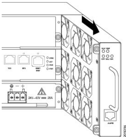
図 68: ファントレイの取り外し
