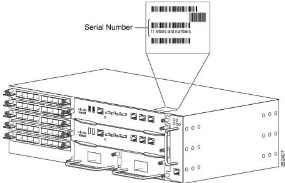
図 42: Cisco ASR 903 ルータのシリアル番号の位置
