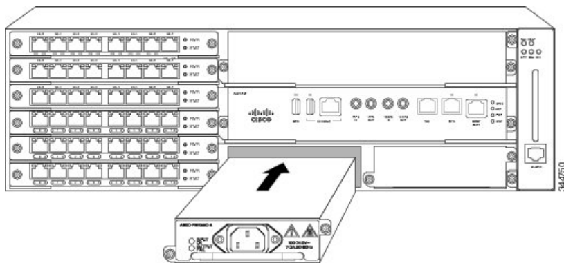
図 74: A900-PWR1200-A の AC 電源の取り付け
