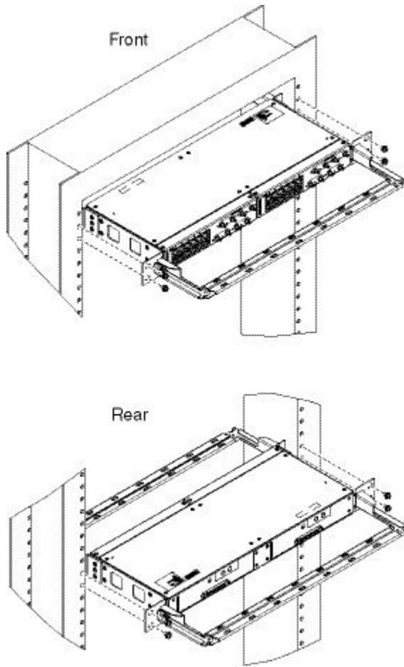
図 99: ラック (デュアル) への 21 インチ ブラケットの取り付け
