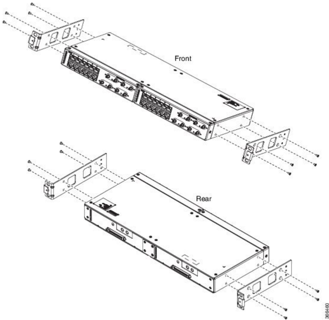
図 87: 19 インチ ラック へのパッチ パネル (デュアル) の取り付け
