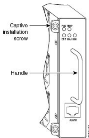
図 67: ファントレイの取り外し
