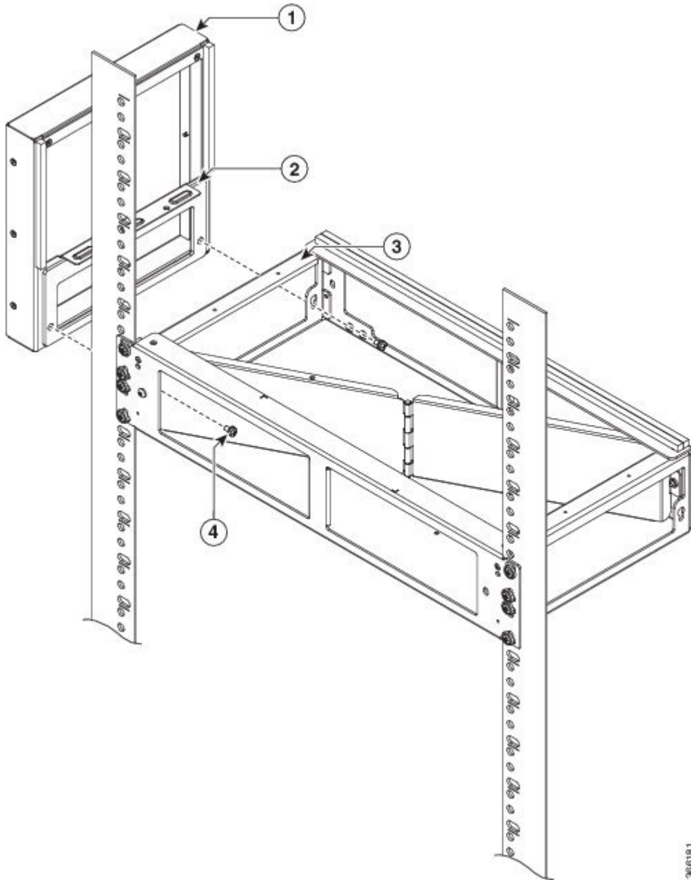
図 53: エアーバッフルトレイの固定
