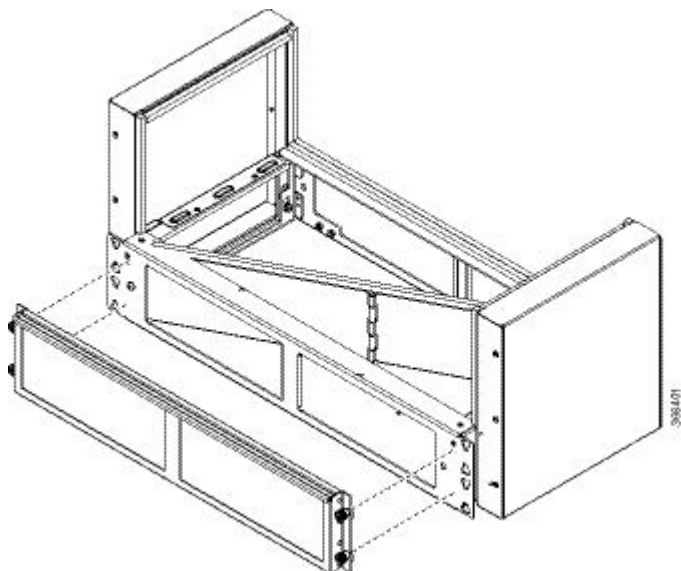
図 55: エアー フィルタ
