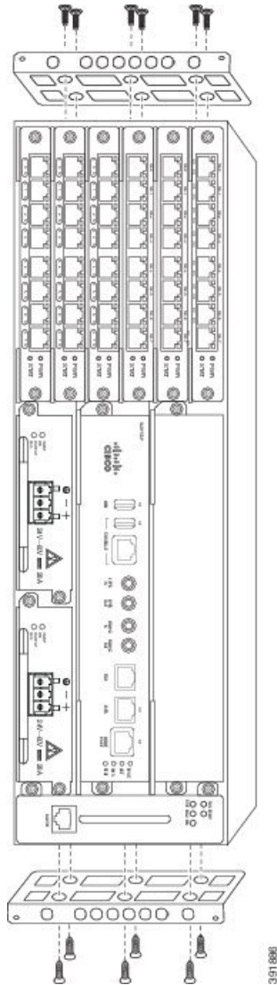
図 51: 垂直取り付け
