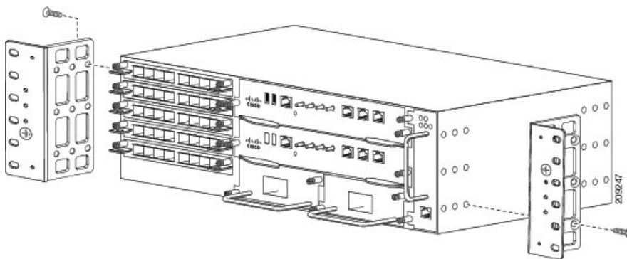
図 47: 300 mm ETSI キャビネット用のマウントブラケットの取り付け
