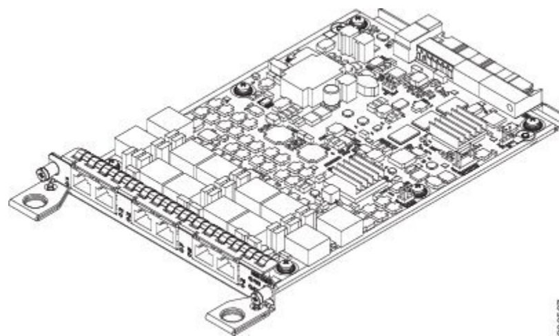
図 39: EアンドMインターフェイスモジュール
