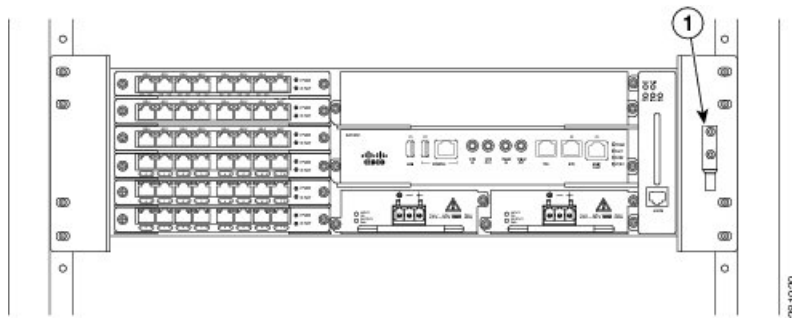
図 63: ラックマウント ブラケットへのアース ラグの取り付け
