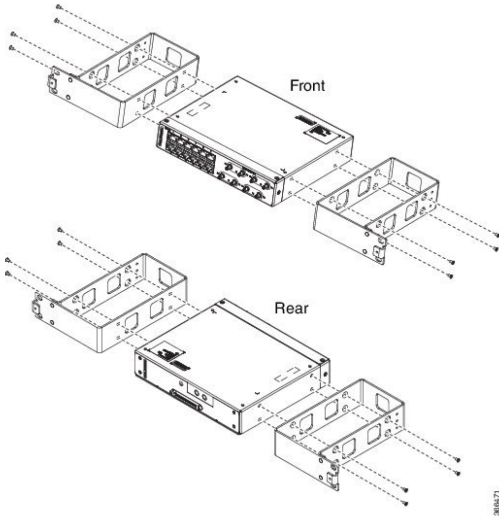
図 86: 19 インチ ラックへのパッチパネル（シングル）の取り付け
