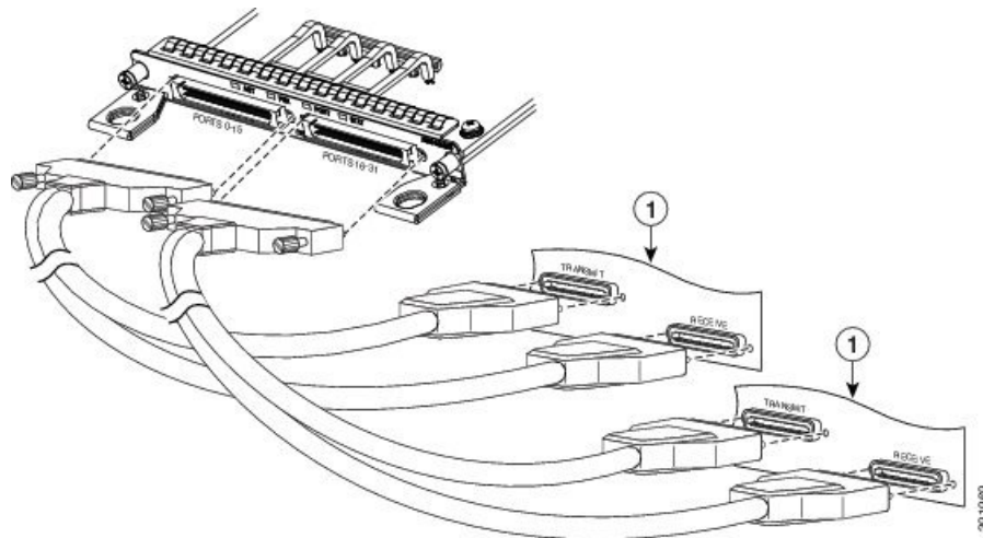
図 83: 32 x T1/E1 インターフェイスとパッチ パネル間のケーブルの取り付け
