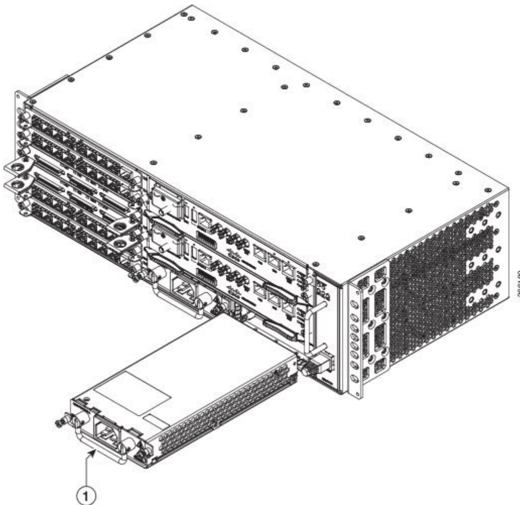
図 74: A900-PWR1200-A の AC 電源の取り付け
