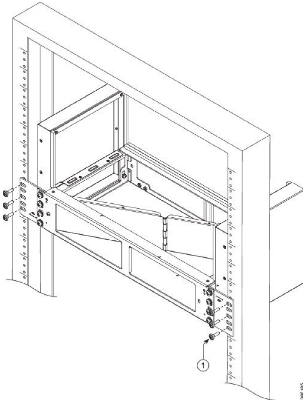
図 58: 23 インチ ラックへのプレナム アセンブリの取り付け
