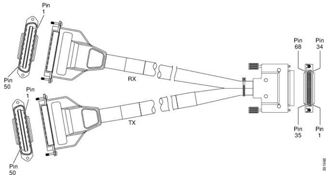
図 82: 32 x T1/E1 ケーブル コネクタ
