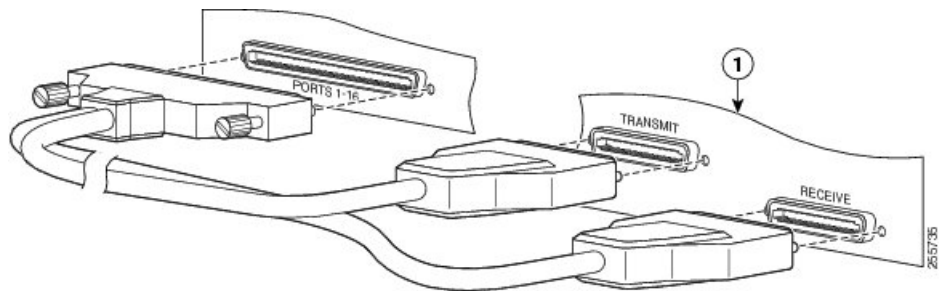
図 81: 16 x T1/E1 インターフェイスとパッチパネル間のケーブルの取り付け
