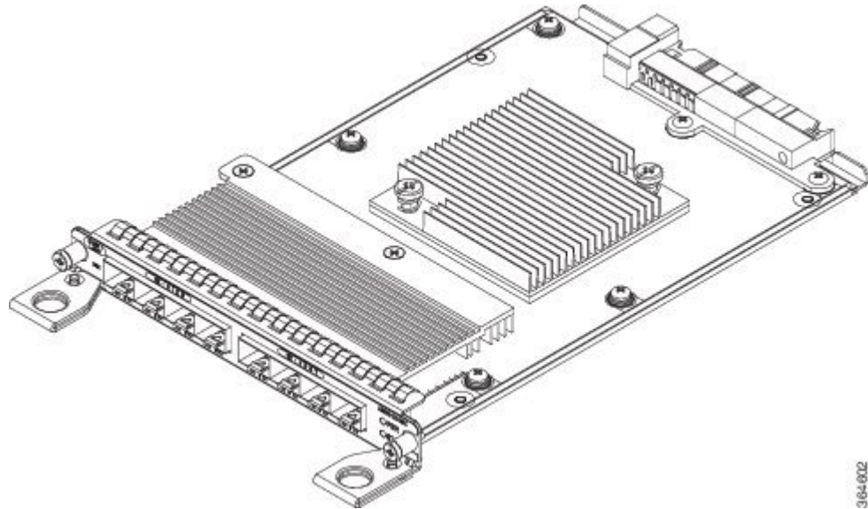
図 19: 8ポート10ギガビットイーサネットインターフェイスモジュール
