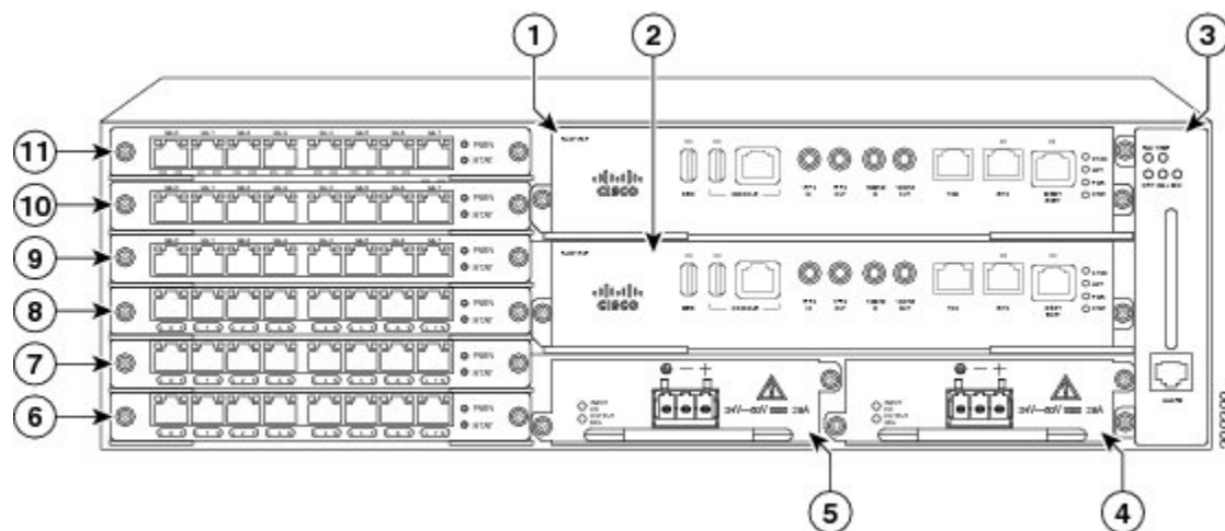
図 43: Cisco ASR 903 ルータのスロット番号
