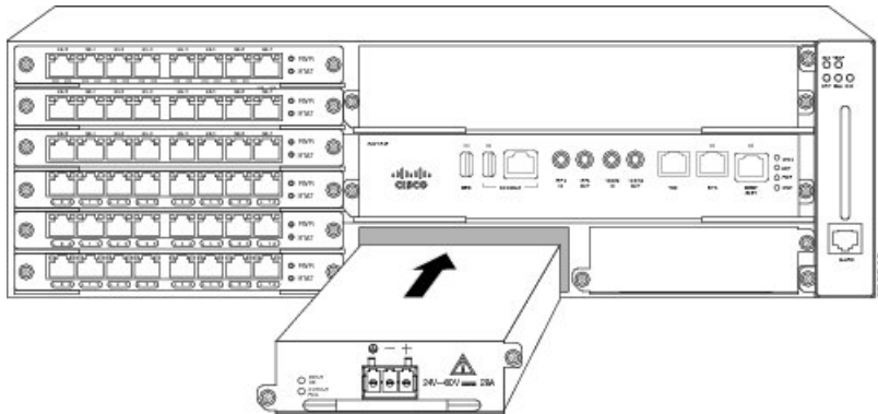
図 71: DC 電源の取り付け
