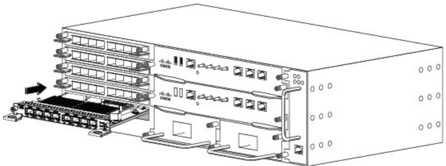
図 70: インターフェイス モジュールの挿入
