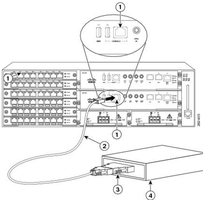
図 77: Cisco ASR 903 ルータへのモデムの接続
