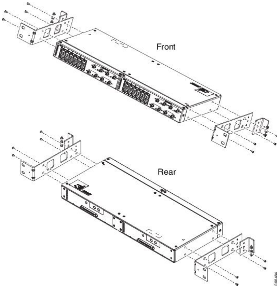
図 89: 21 インチ ラックへのパッチパネル (デュアル) の取り付け
