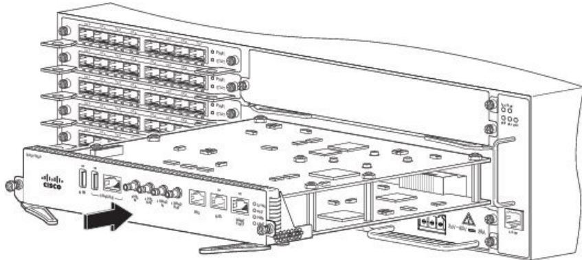
図 69: Cisco ASR 903 ルータの RSP の取り付け
