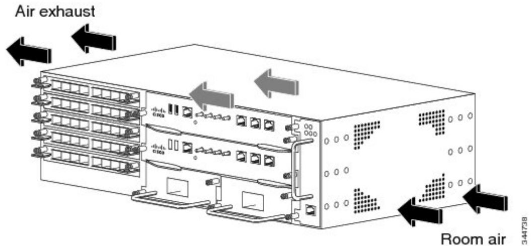
図 44: Cisco ASR 903 ルータ シャーシのエアフロー
