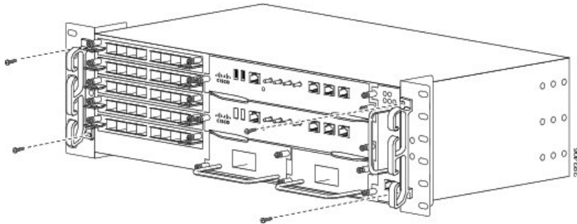
図 61: ケーブル管理ブラケット (A903-CAB-BRACKET)
