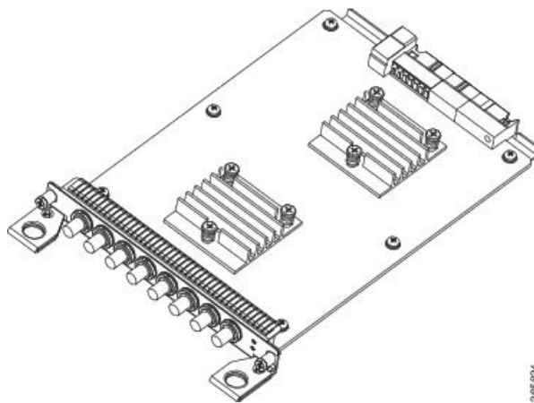
図 41: C37.94 インターフェイス モジュールの前面パネル
