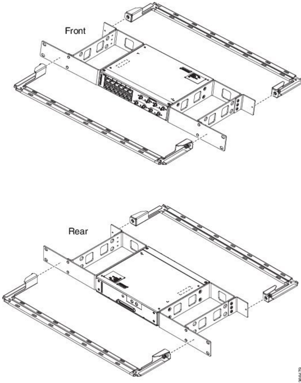
図 100: パッチパネル (シングル) への 23 インチ ブラケットの取り付け
