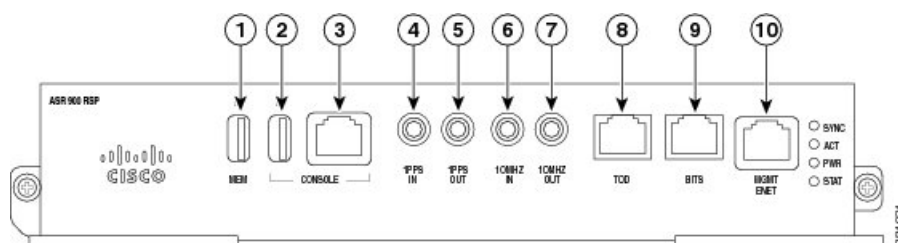
図 12: Cisco RSP1 インターフェイスの概要
