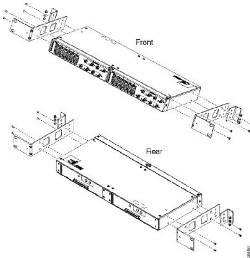
図 91: 23 インチ ラックへのパッチパネル（デュアル）の取り付け
