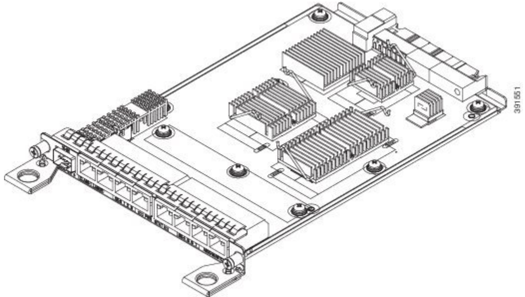
図 21: 8ポート 1 GE (RJ45) + 1ポート 10 GE SFP+ インターフェイス モジュール
