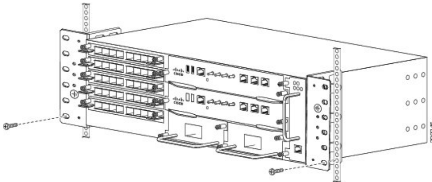
図 50: 300 mm ETSI キャビネットへのシャーシの取り付け
