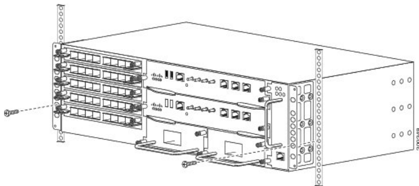
図 48: 19 インチ EIA ラックへのシャーシの取り付け
