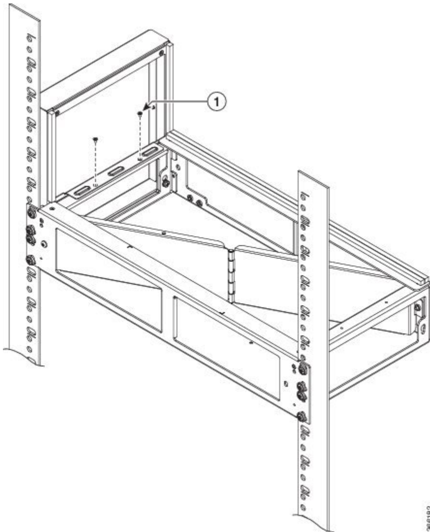
図 54: サイドプレートの固定
