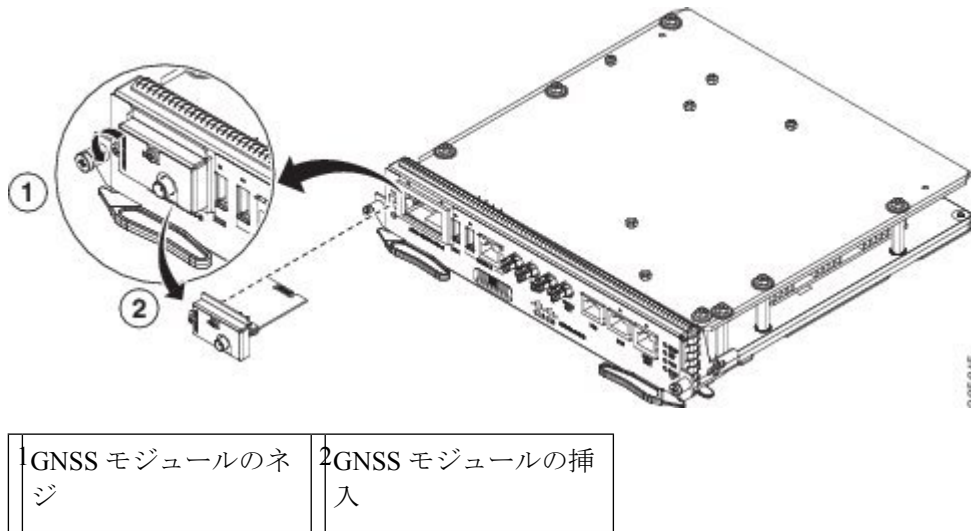
図 79: RSP への GNSS モジュールの取り付け
