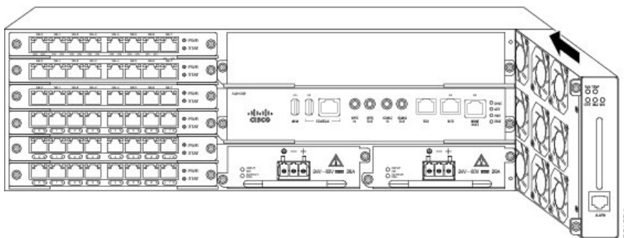
図 66:ファントレイの取り付け
