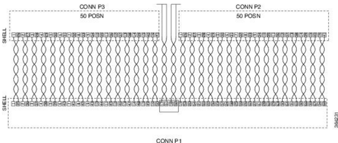
図 105: 32 T1/E1 インターフェイスとパッチパネル間のケーブルの 32 T1/E1 配線図
