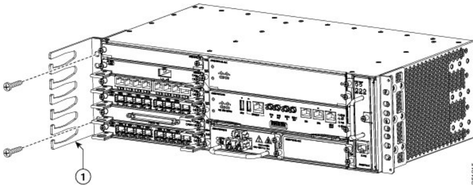
図 61: ケーブル管理ブラケット (A903-CAB-BRACKET)
