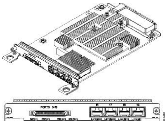
図 34: A900-IMA3G-IMSG ギガビットイーサネットインターフェイス モジュール
