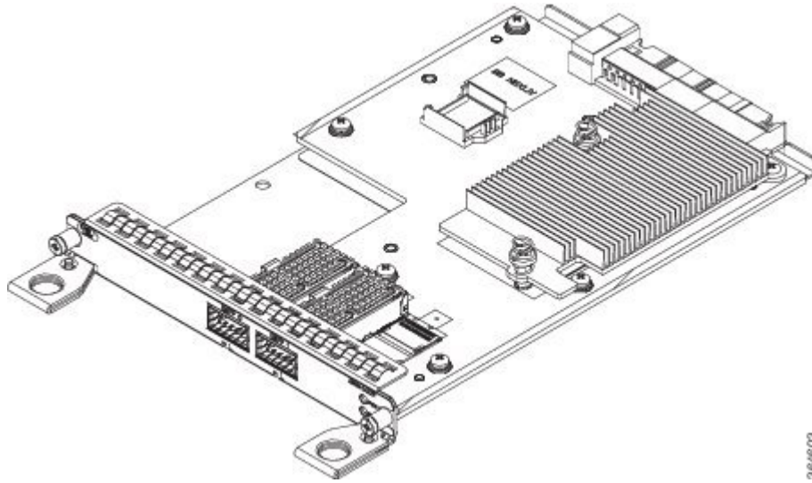
図 24: 2 ポート 40 ギガビットイーサネットインターフェイス モジュール
