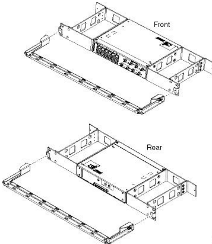
図 92: パッチパネル (シングル) への 19 インチ ブラケットの取り付け
