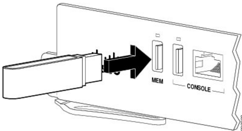
図 78: Cisco ASR 903 ルータのフラッシュ トークン メモリ スティック
