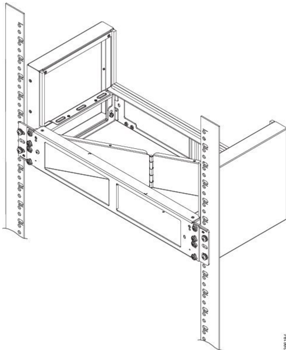
図 57: 21 インチ ラックへのプレナム アセンブリの取り付け
