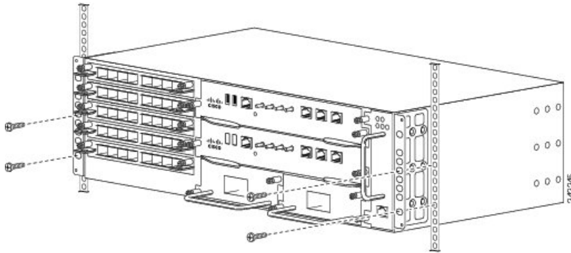
図 50: 300 mm ETSI キャビネットへのシャーシの取り付け
