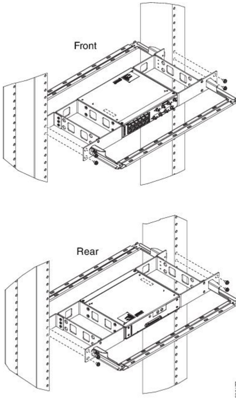
図 97: ラック（シングル）への 21 インチ ブラケットの取り付け
