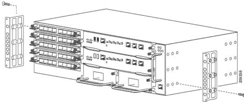
図 46: 19 インチ EIA ラック用のマウントブラケットの取り付け
