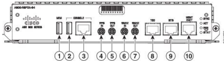
図 13: Cisco A900-RSP2A インターフェイスの概要
