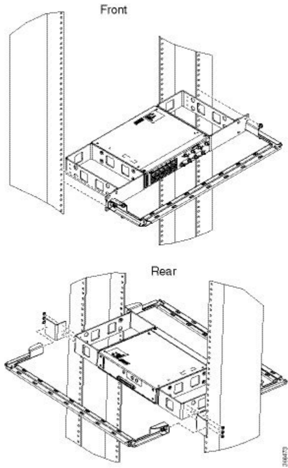
図 93: ラック (シングル) への 19 インチ ブラケットの取り付け
