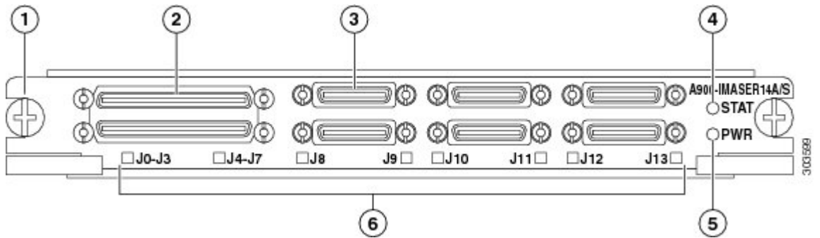
図 38: 14ポート シリアルインターフェイス モジュールの前面パネル
