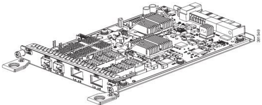
図 22: 2ポート 10ギガビットイーサネット インターフェイス モジュール
