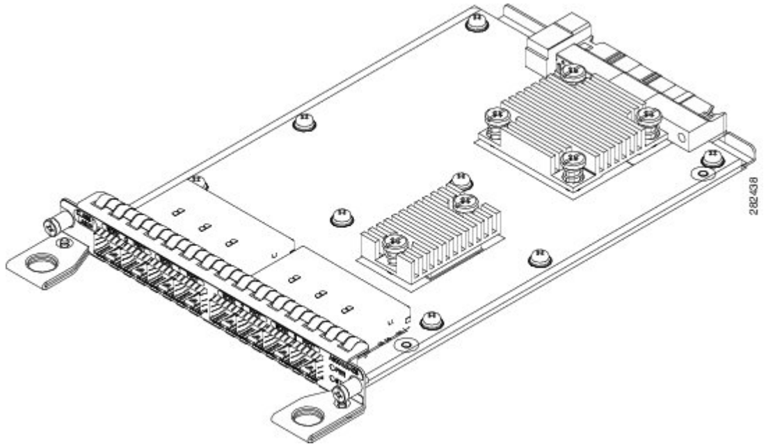
図 33: 4ポート OC-3 インターフェイス モジュール
