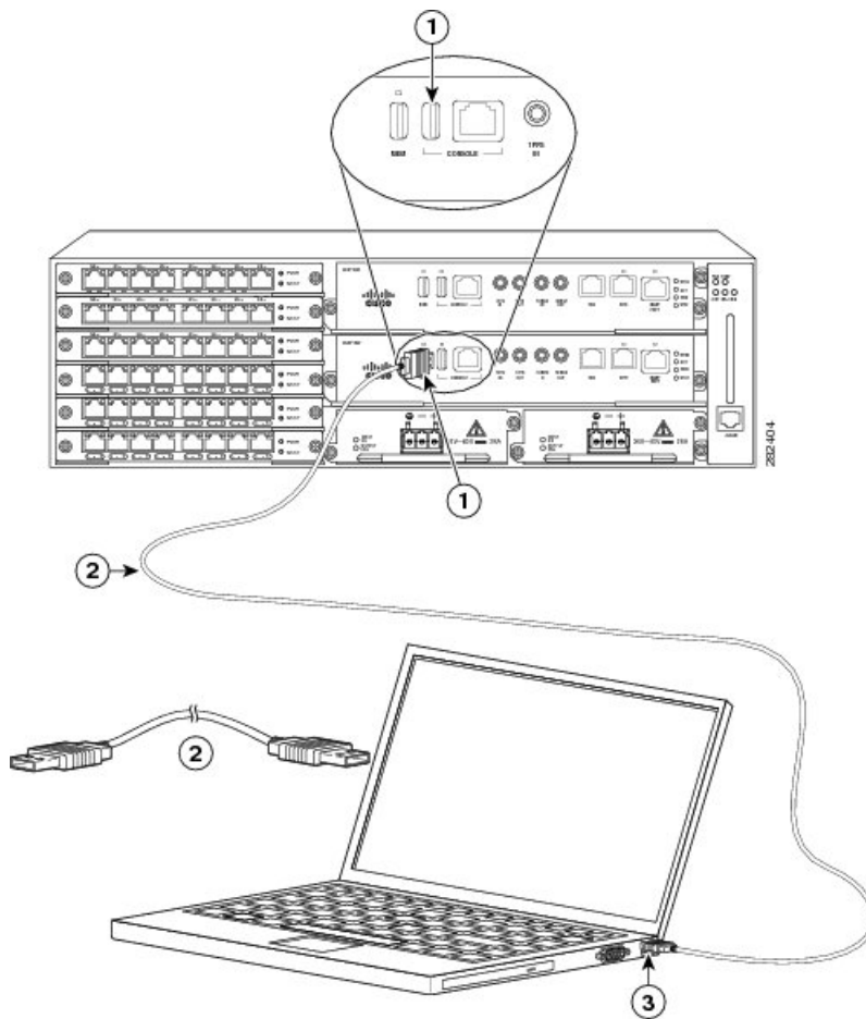
図 76: USB コンソールケーブルの Cisco ASR 903 ルータへの接続
