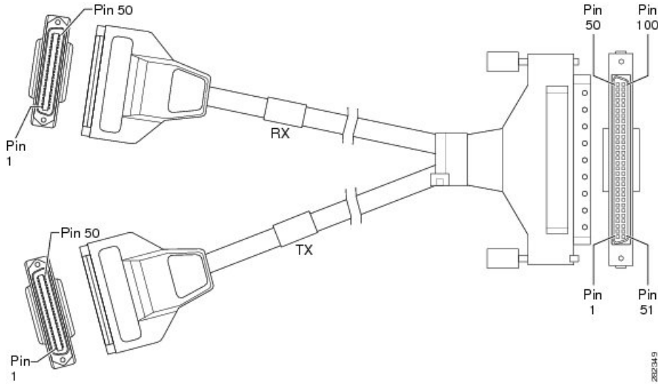
図 80: 16 x T1/E1 ケーブル コネクタ
