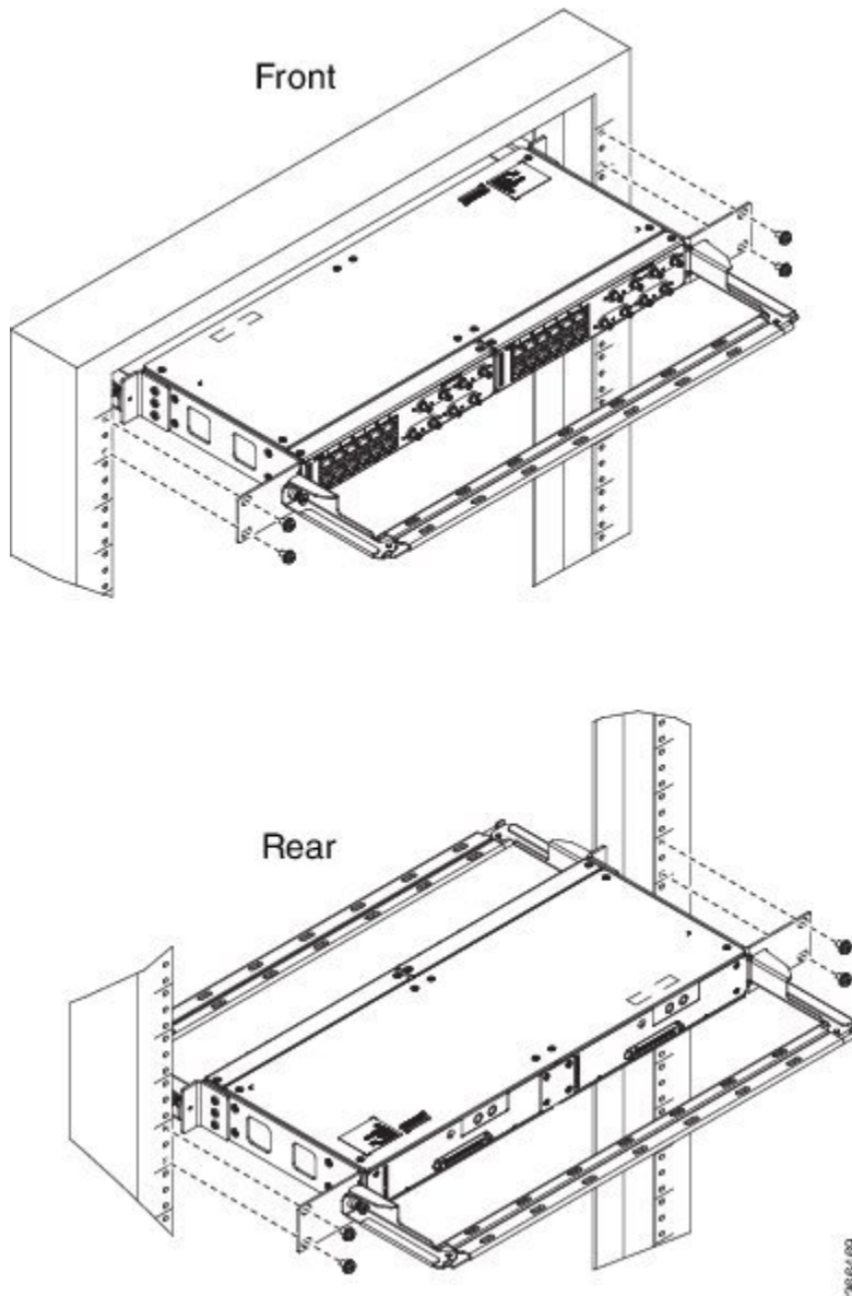
図 103: ラック (デュアル) への 23 インチ ブラケットの取り付け
