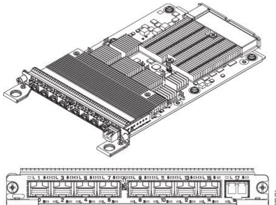
図 25: A900-IMA8CS1Z-M ギガビットイーサネットインターフェイス モジュール
