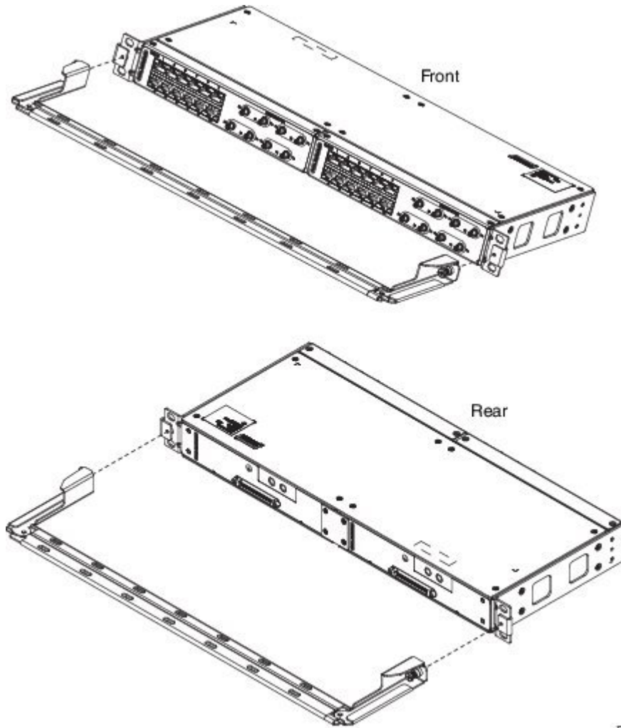
図 94: パッチパネル (デュアル) への 19 インチ ブラケットの取り付け
