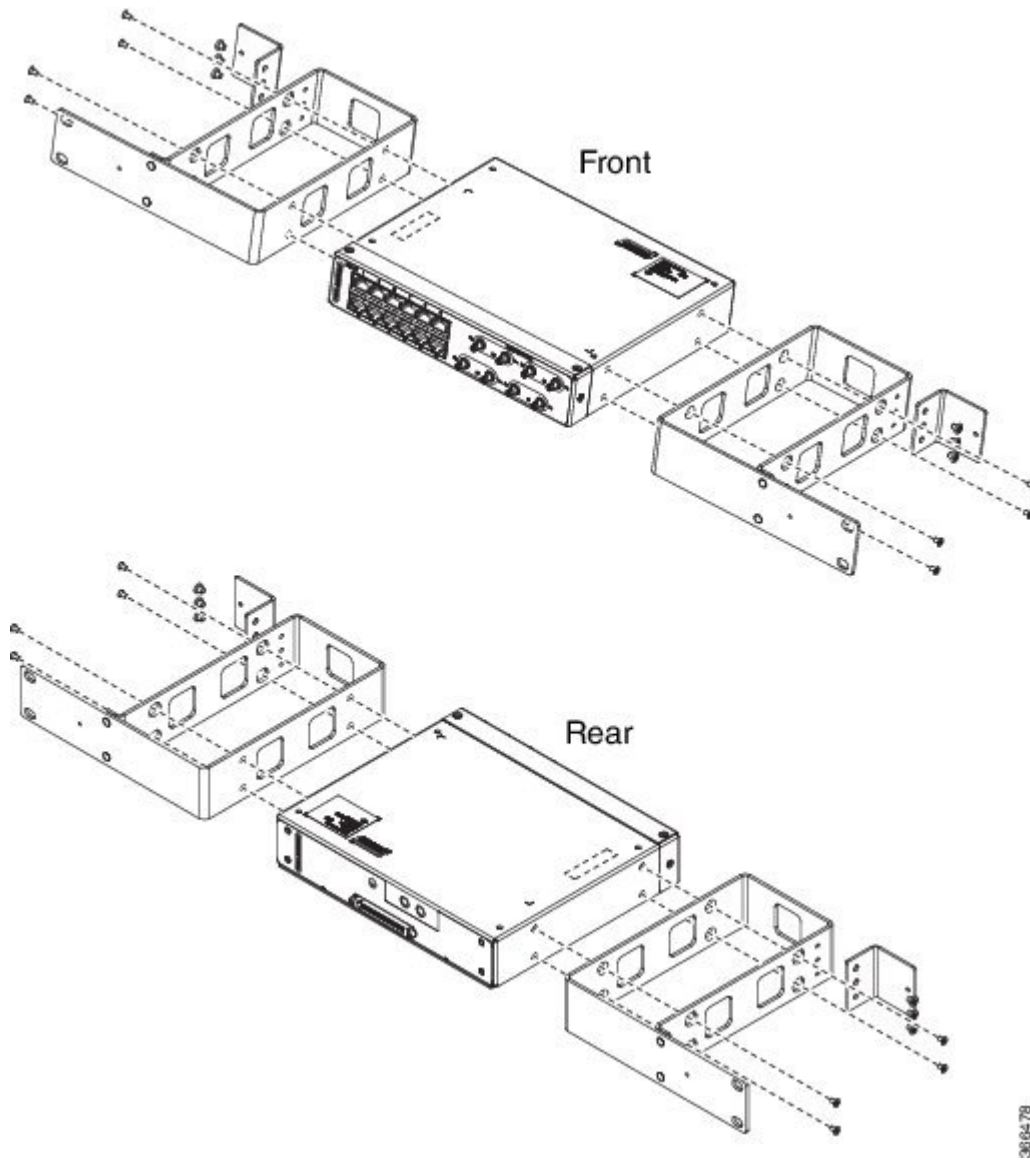
図 90: 23 インチ ラックへのパッチパネル（シングル）の取り付け
