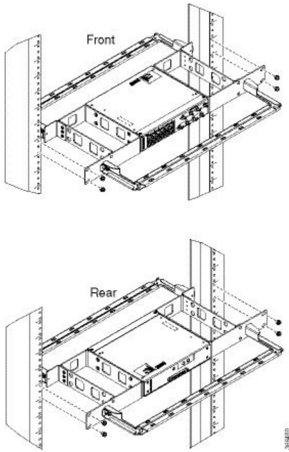
図 101: ラック (シングル) への 23 インチ ブラケットの取り付け
