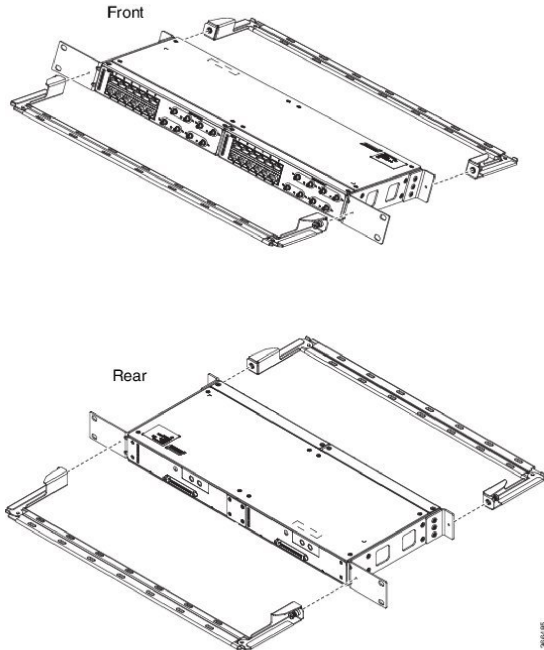
図 102: パッチパネル (デュアル) への 23 インチ ブラケットの取り付け
