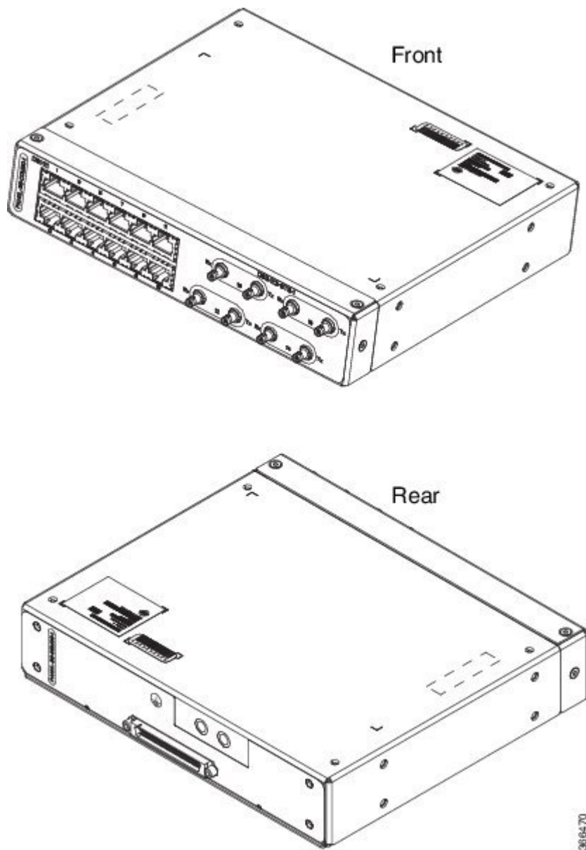
図 84: パッチパネルのアース - シングル
