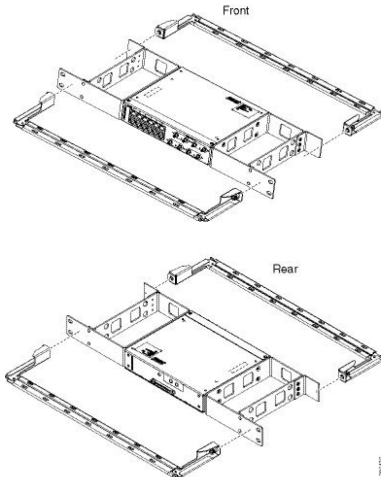
図 96: パッチパネル (シングル) への 21 インチ ブラケットの取り付け
