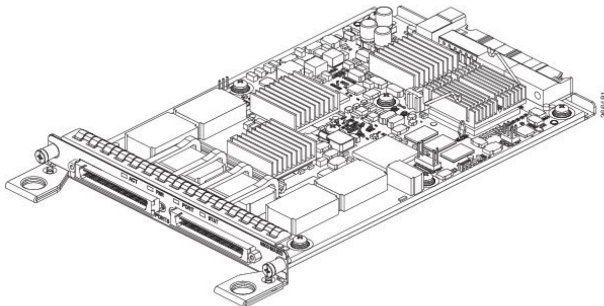
図 27: 32ポート T1/E1 インターフェイス モジュール
