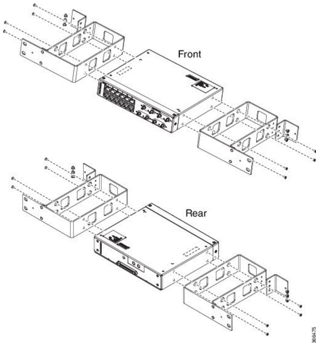
図 88: 21 インチ ラックへのパッチパネル (シングル) の取り付け
