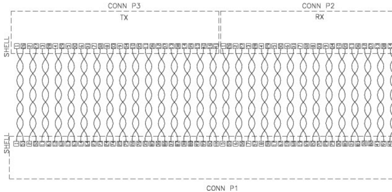
図 104: 16 T1/E1 インターフェイスとパッチ パネル間のケーブルの配線図
