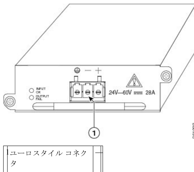
図 2: ユーロスタイル コネクタ付き DC PSU モジュール (A900-PWR550-D)
