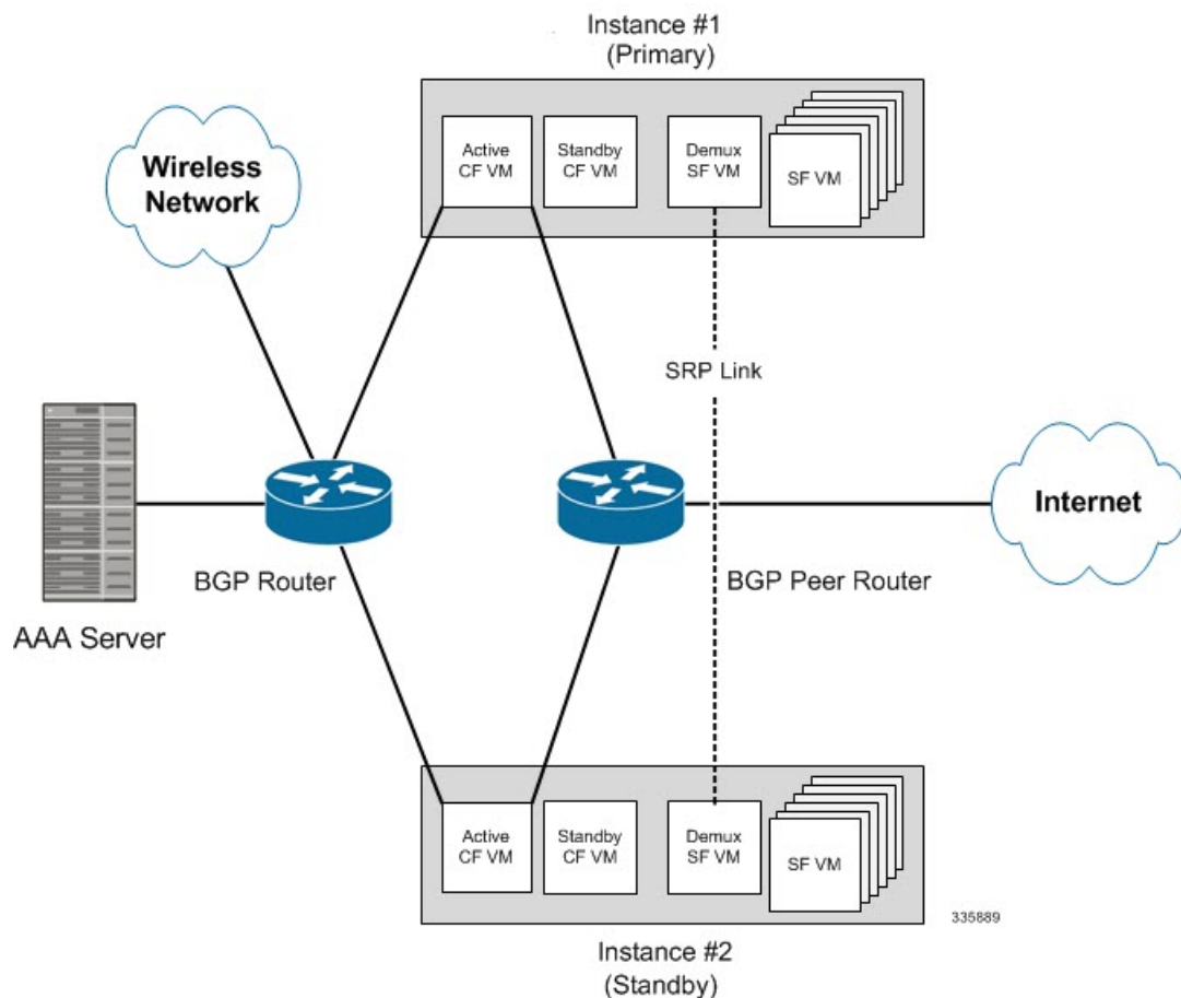
図 1: 仮想化された StarOS の ICSR のネットワーク
