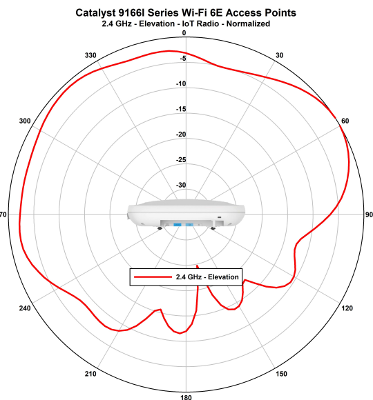
Figure 18: CW91661 - IoT (BLE) アンテナ正規化放射パターン (2.4 GHz 垂直)
