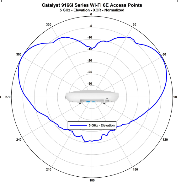
Figure 10: CW9166I - XOR 正規化放射パターン (5 GHz 垂直)
