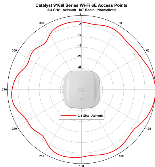
Figure 17: CW91661 - IoT (BLE) アンテナ正規化放射パターン (2.4 GHz 水平)
