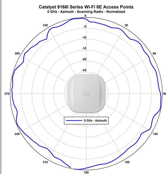
Figure 13: CW9166I - スキャン無線正規化放射パターン (5 GHz 水平)
