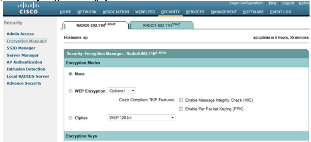
図 12-10 [Encryption Manager] ページ
