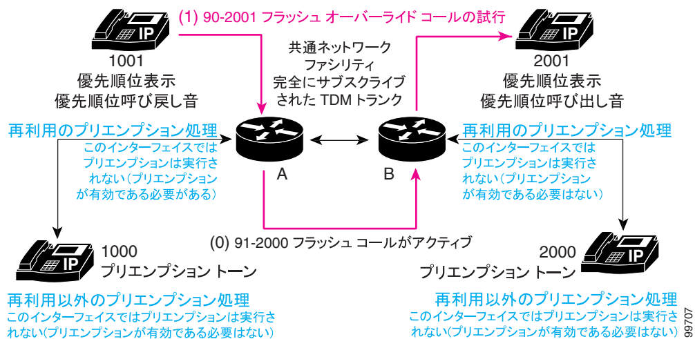
図 34-7 共通ネットワーク ファシリティ プリエンプションの例
