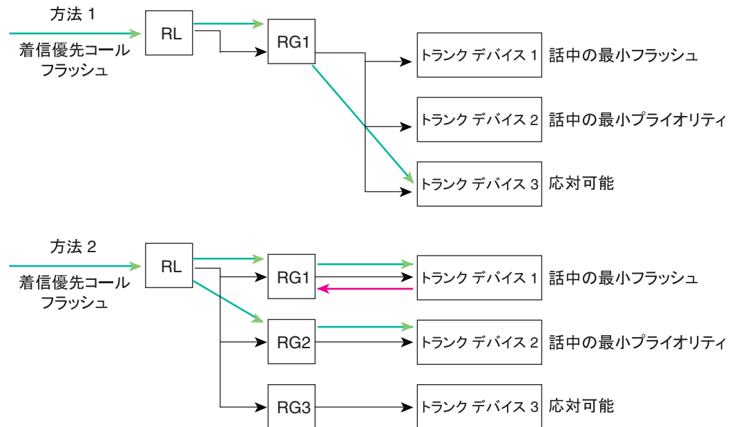
図 34-15 MLPP トランク 選択 (ハント) の例
