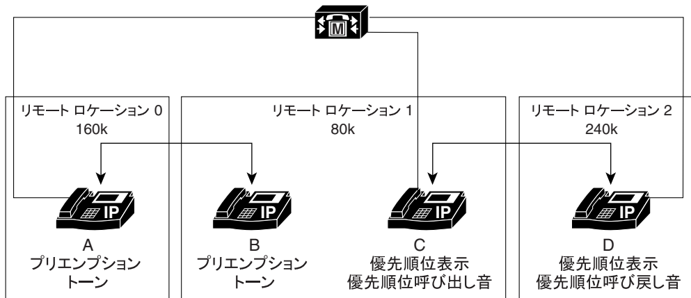
図 34-9 別のデバイスにおけるロケーションベースのプリエンプション
