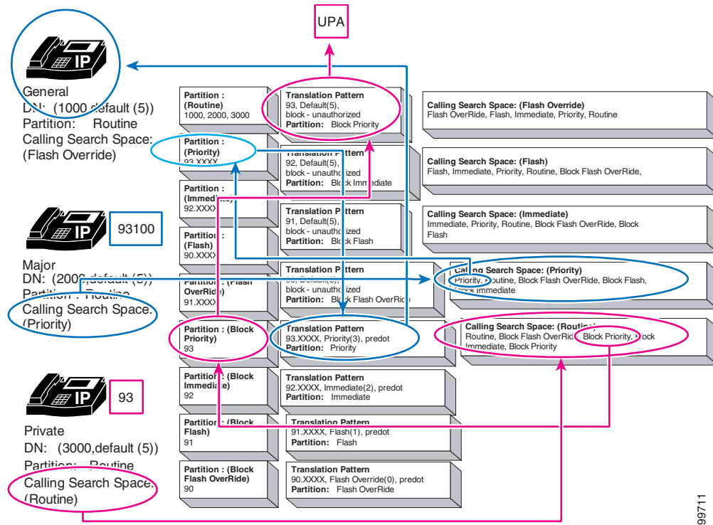
図 34-14 優先順位パターン用の MLPP 番号計画アクセス制御の例
