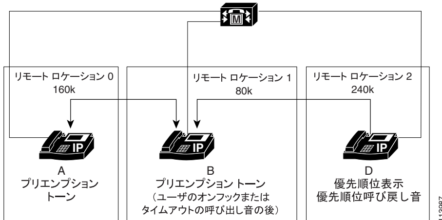
図 34-10 同一デバイスでのロケーションベースのプリエンプレッション
