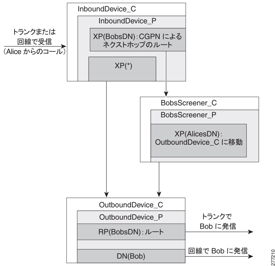
図 25-1 発信側番号ルーティングを使用したコールのスクリーニング
