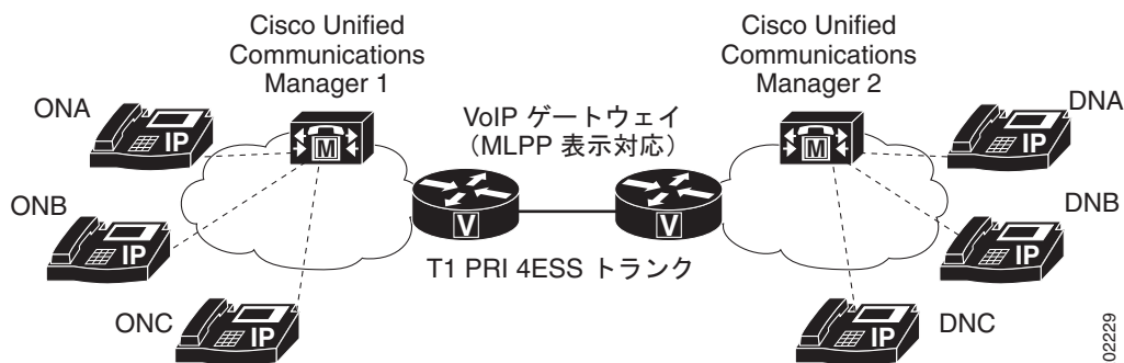
図 34-1 エクゼクティブ オーバーライド優先コールの例
