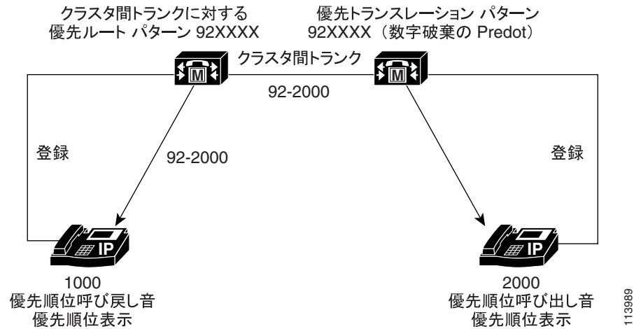
図 34-4 クラスタ間トランクの間での優先コールの設定例
