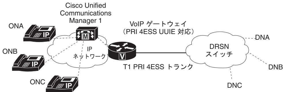
図 34-3 PRI 4ESS インターフェイス間のエクゼクティブ オーバーライド優先コール
