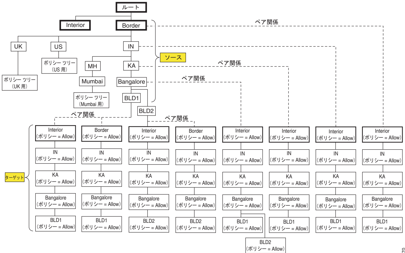
図 31-1 インドクラスタに適用される論理パーティション ポリシーのポリシー ツリーの例
