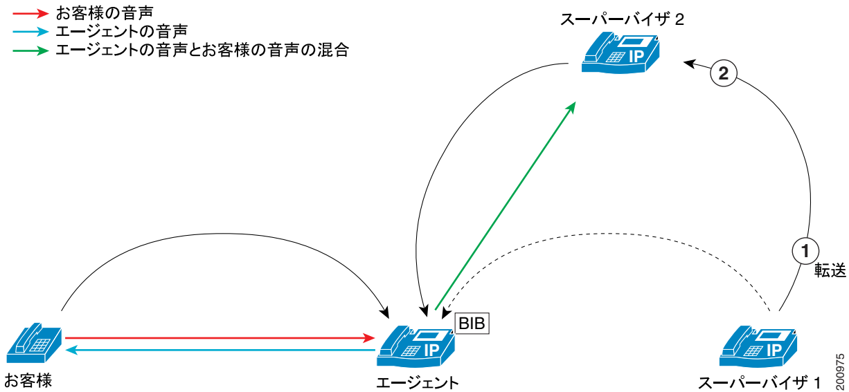
図 33-7 スーパーバイザがモニタリング コールを転送する場合
