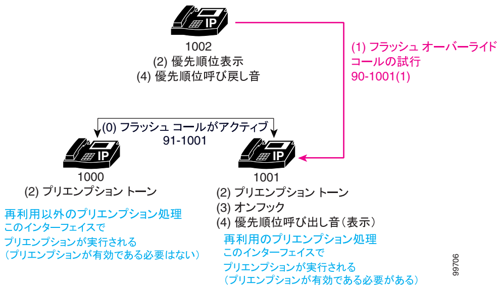
図 34-6 ユーザ アクセス プリエンブションの例
