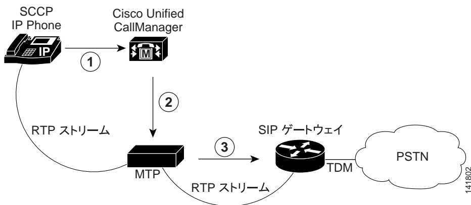
図 41-3 DTMF デジタルの生成
