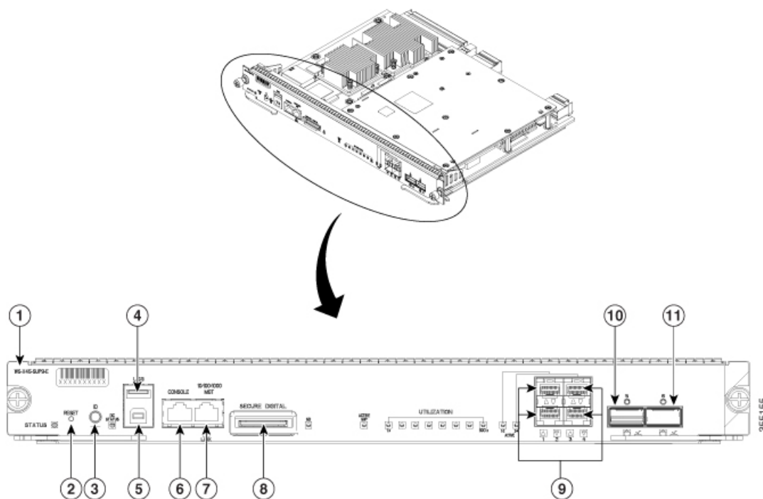
図 1: Cisco Catalyst 4500 E シリーズ Supervisor Engine 9-E
