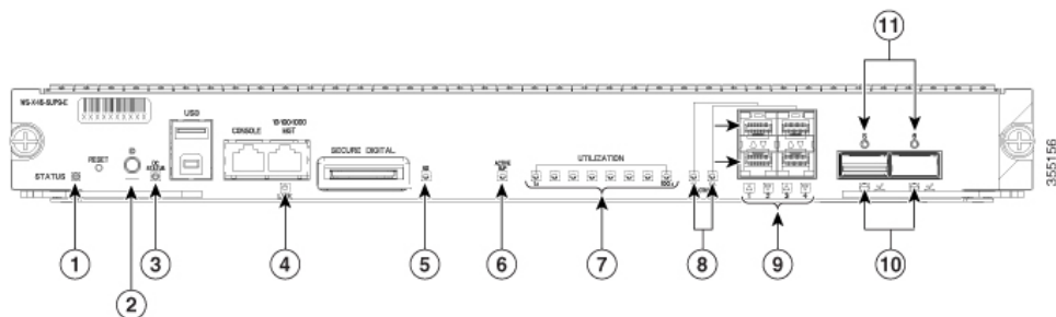
図 2: Cisco Catalyst 4500 E シリーズ Supervisor Engine 9-ELED
