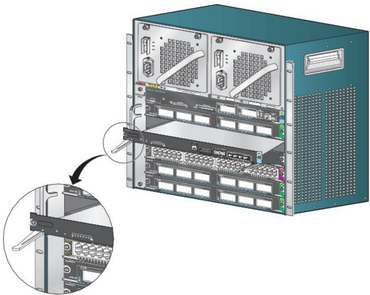
図 3: シャーシへのスーパーバイザエンジンの取り付け（図は Catalyst 4507R+E ）
