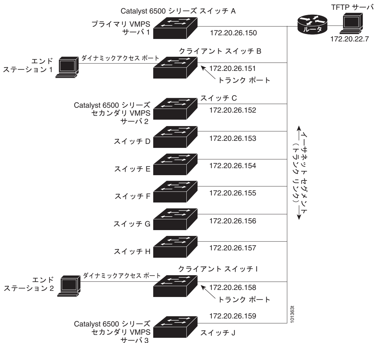
図 16-4 ダイナミック ポート VLAN メンバーシップの構成例
