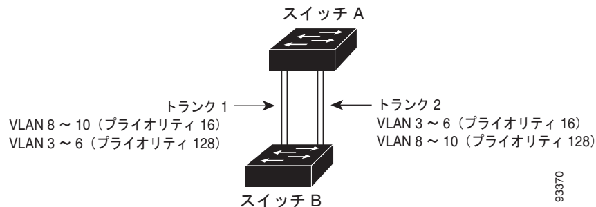
図 16-2 STP ポート プライオリティによる負荷分散
