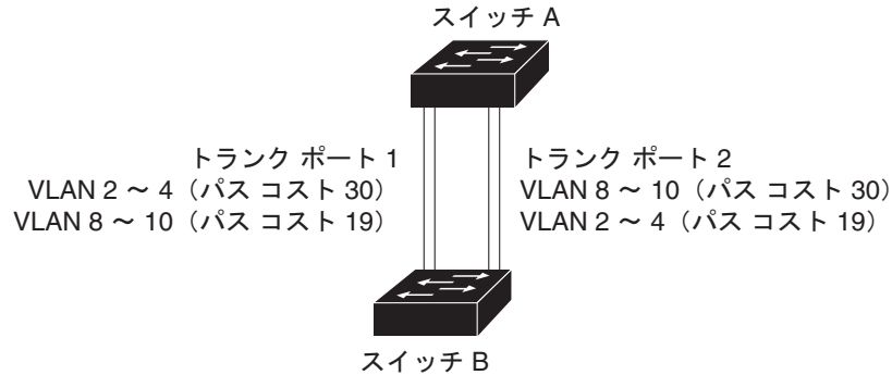
図 16-3 パス コストによってトラフィックが分散される負荷分散トランク
