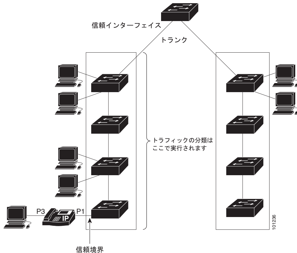
図 39-12 QoS ドメイン内のポートの信頼状態
