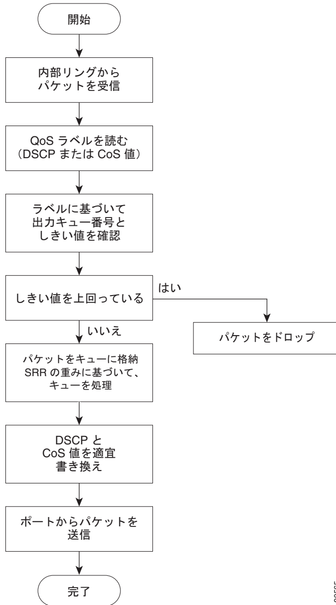
図 39-9 出力ポートのキューイングおよびスケジューリング フローチャート
