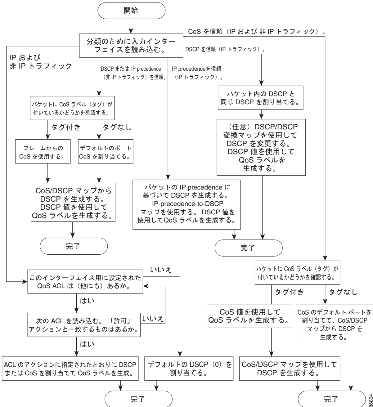
図 39-3 分類フローチャート
