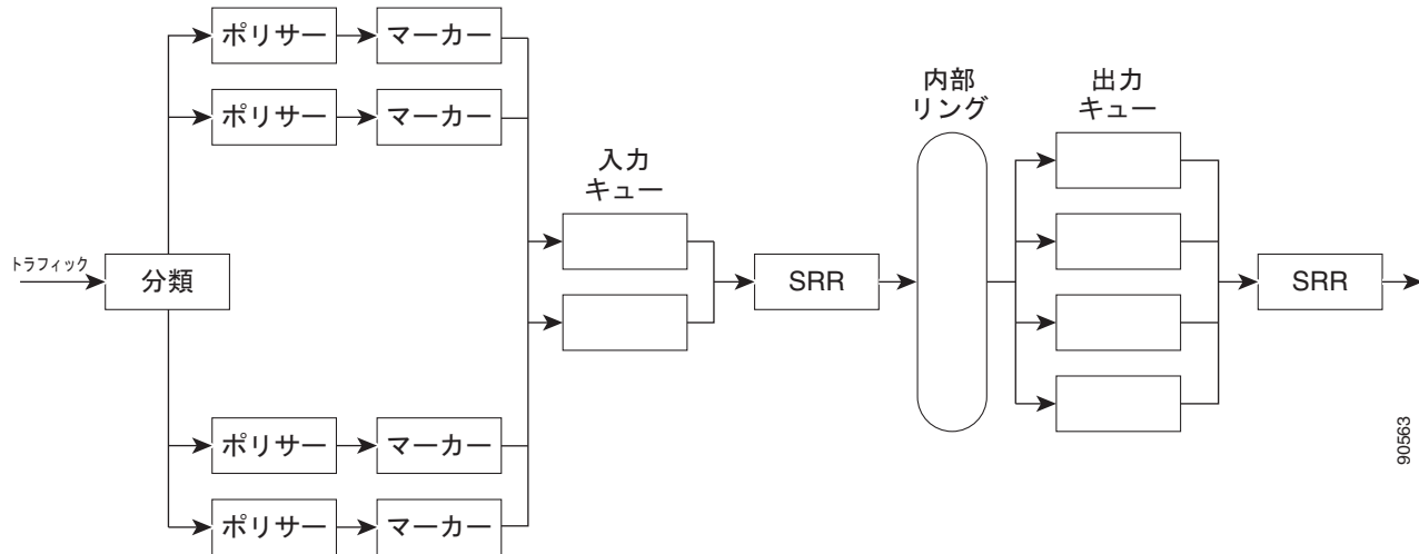
図 39-6 入力および出力キューの位置
