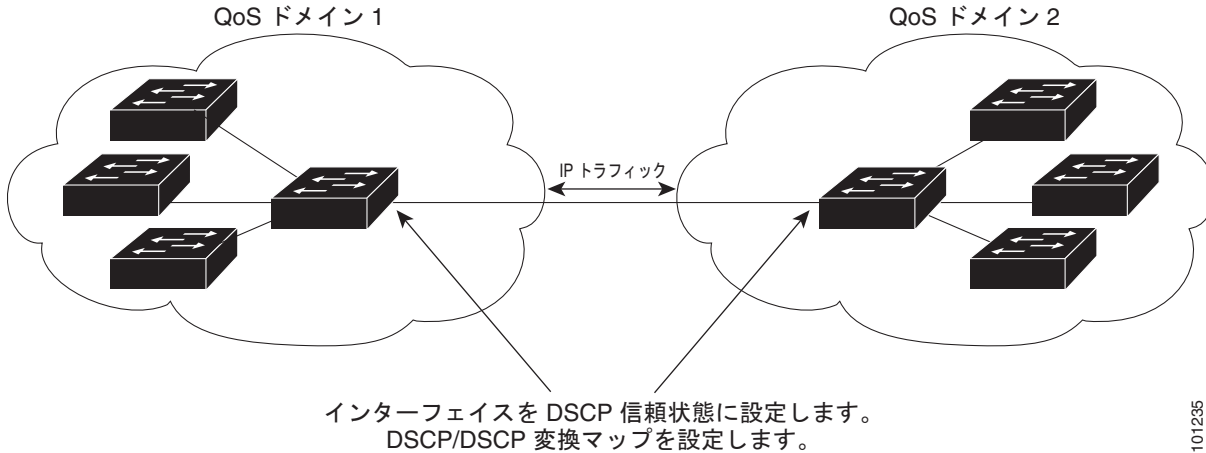
図 39-13 別の QoS ドメインとの境界ポートの DSCP 信頼状態
