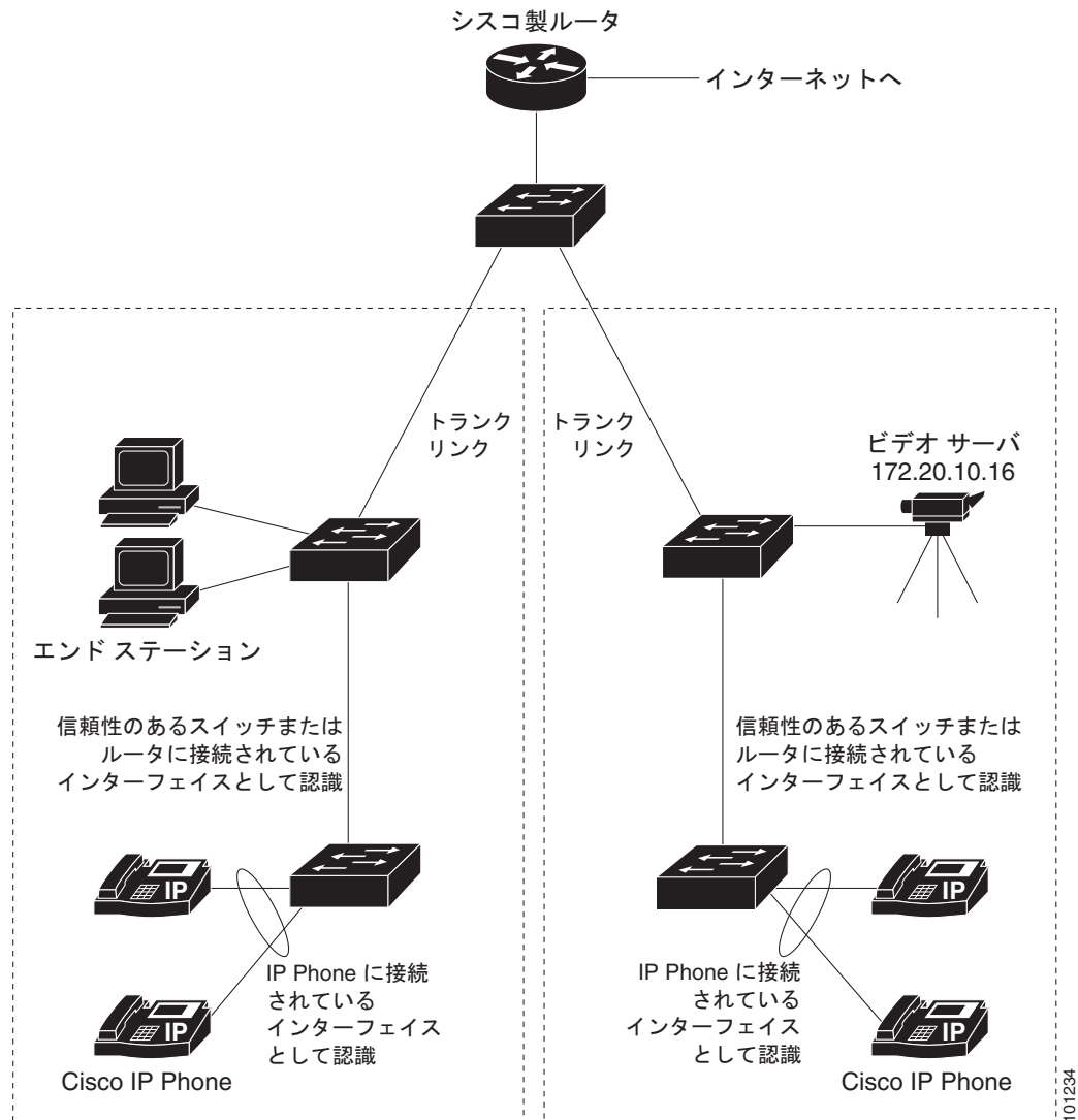
図 39-11 ネットワークでの自動 QoS の設定例
