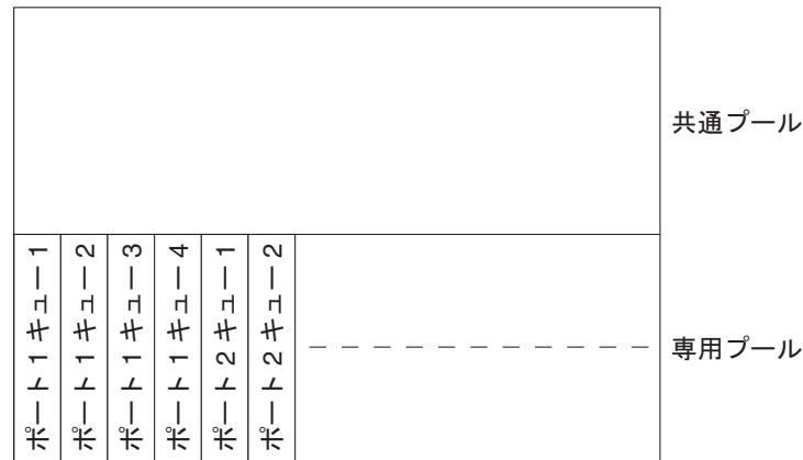
図 39-10 出力キューのバッファ割り当て
