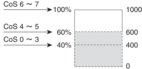
図 39-7 WTD およびキューの動作
