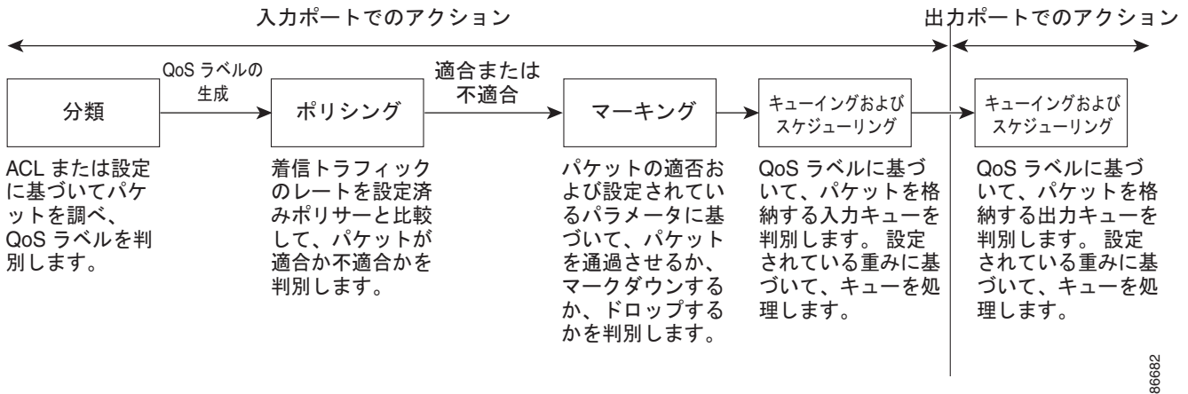
図 39-2 QoS の基本モデル
