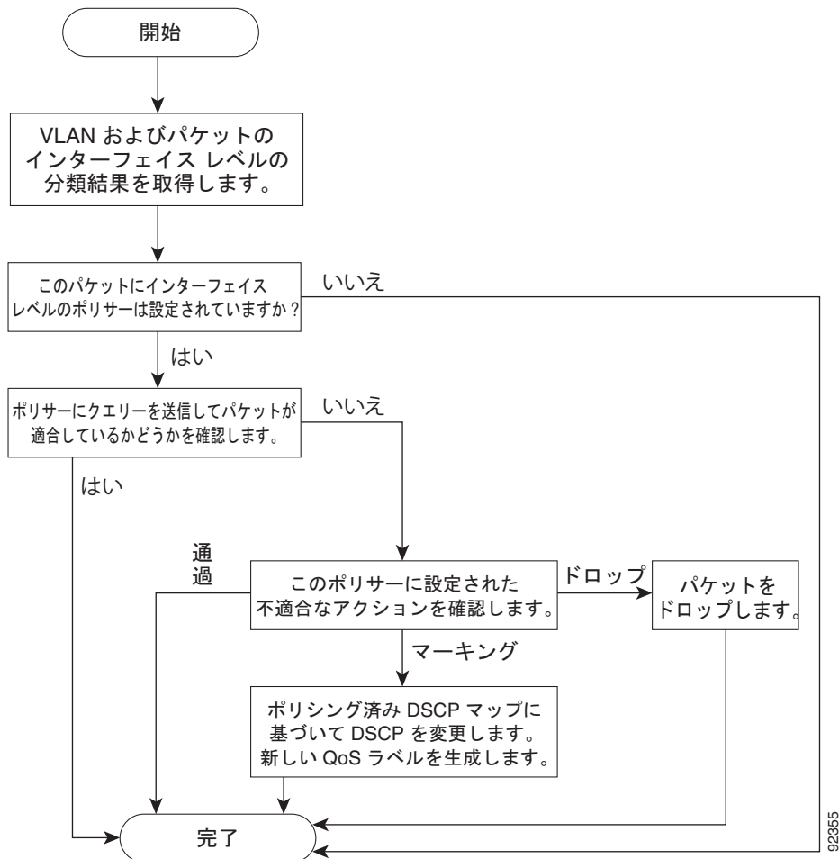
図 39-5 SVI のポリシー マップおよびマーキング フローチャート
