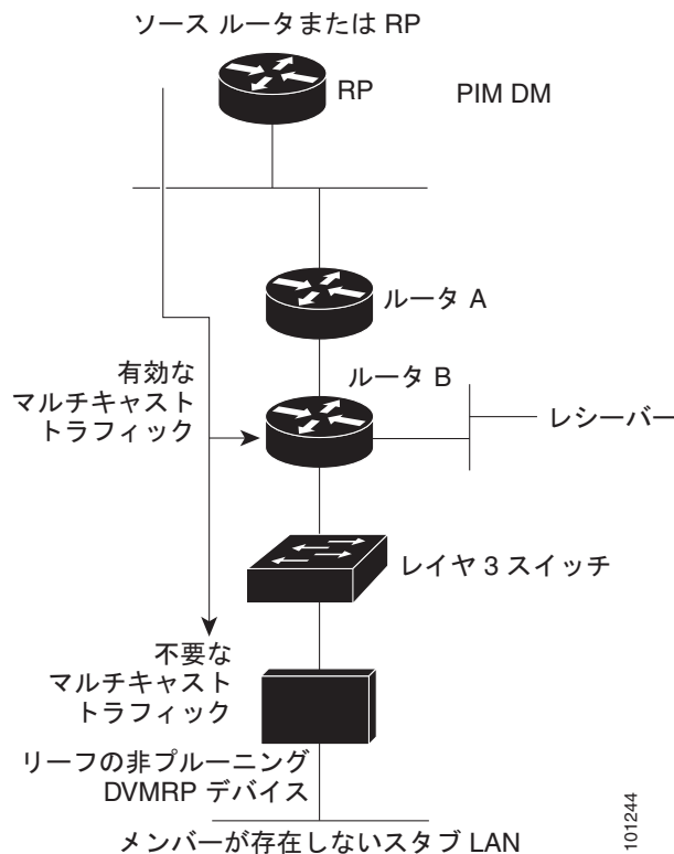
図 50-8 リーフの非プルニング DVMRP ネイバー
