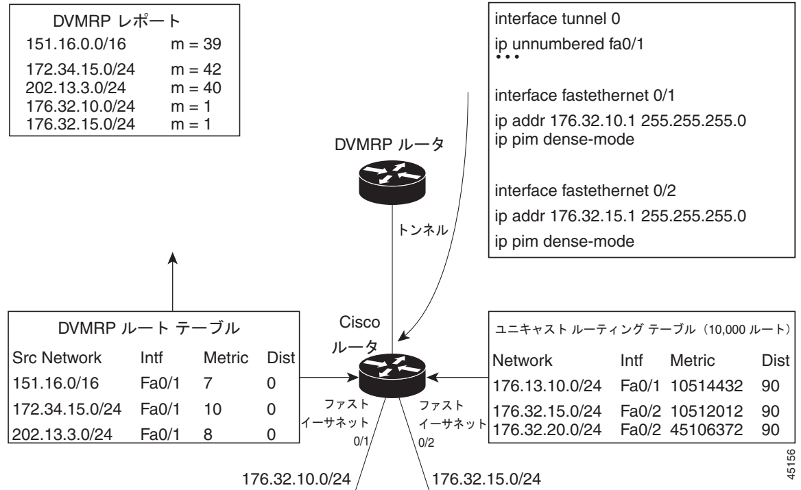
図 50-10 接続されたユニキャスト ルートにだけアドバタイズ (デフォルト) する例
