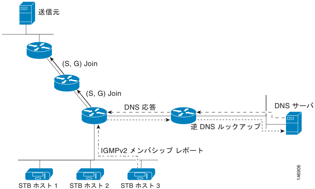
図 50-4 DNS ベースの SSM マッピング
