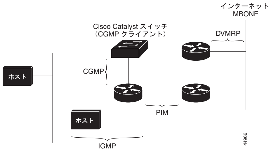
図 50-1 IP マルチキャストルーティング プロトコル
