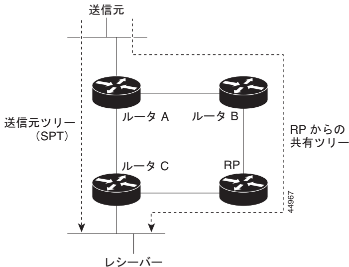
図 50-6 共有ツリーおよび送信元ツリー (SPT)
