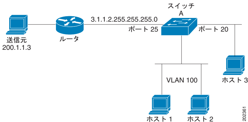
図 50-2 PIM スタブ ルータ設定
