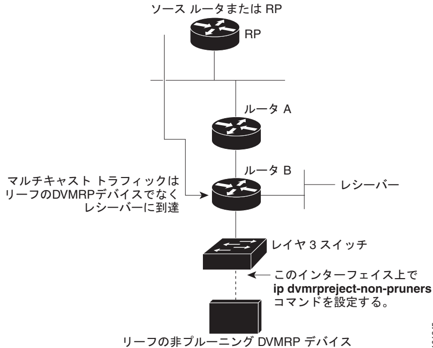
図 50-9 ルータが非プルーフ DVMRP ネイバーを拒否する例
