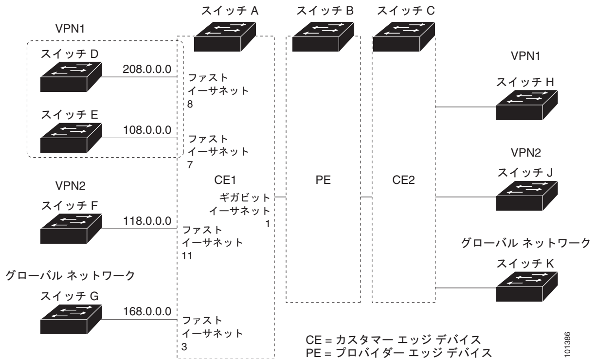
図 41-7 Multi-VRF CE の設定例
