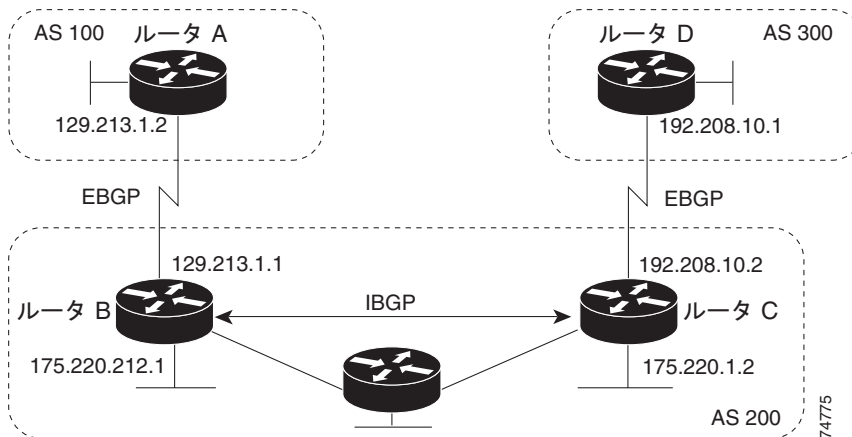
図 41-5 EBGP、IBGP、および複数の AS
