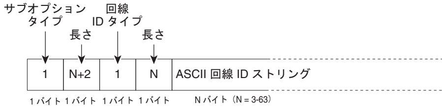
図 26-3 ユーザ設定のサブオプションの packets 形式
