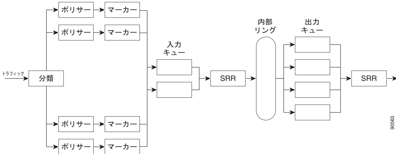
図 39-6 入力および出力キューの位置
