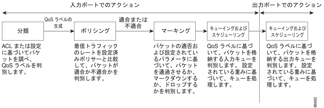
図 39-2 QoS の基本モデル
