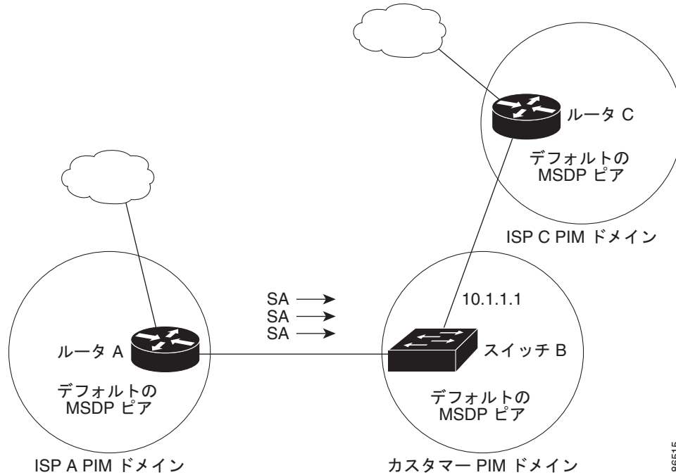
図 51-2 デフォルトの MSDP ピア ネットワーク
