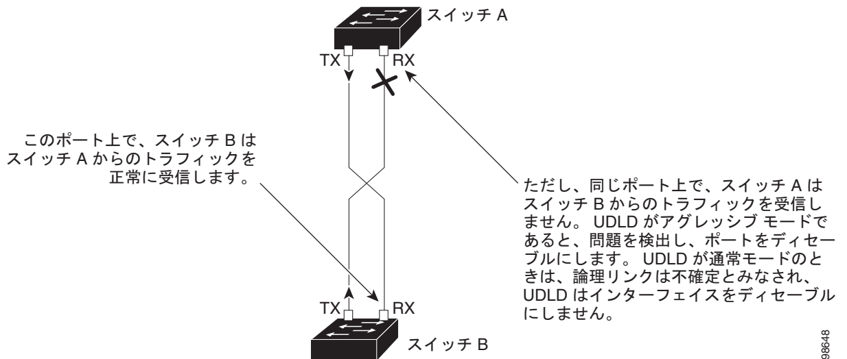
図 31-1 UDLD による単一方向リンクの検出
