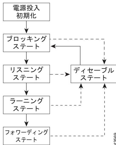
図 19-1 スパンニングツリー インターフェイス ステート
