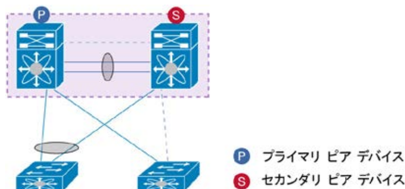
図 45. vPC ピア スイッチを使用するハイブリッド トポロジ (vPC および STP 接続されたアクセス デバイス)
