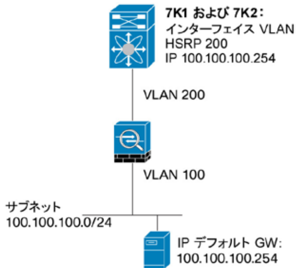
図 74. vPC ドメインに接続されているトランスペアレント モードの ASA : 論理構成図
