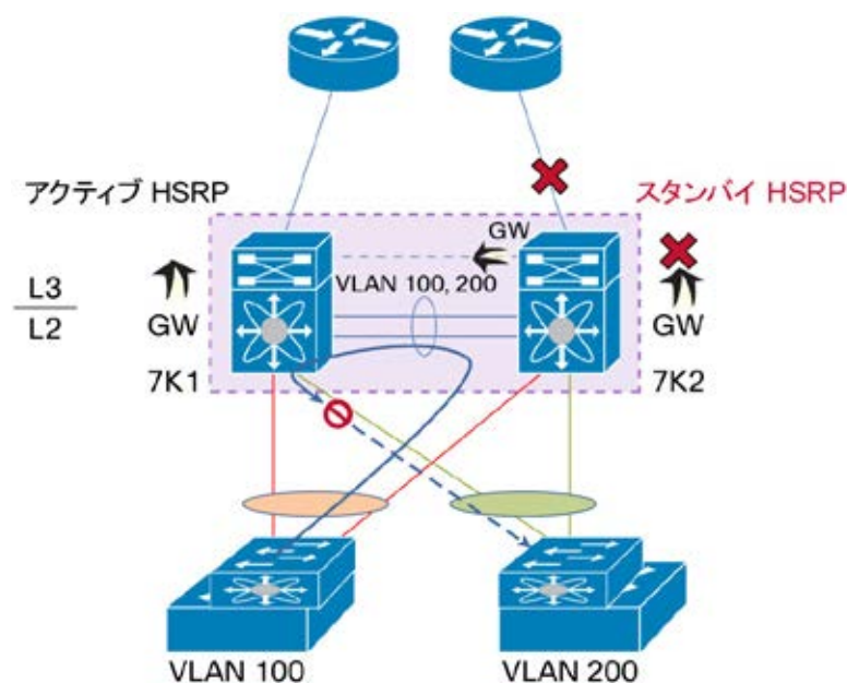
図 67. vPC 設定の HSRP/VRRP オブジェクト トラッキングの問題
