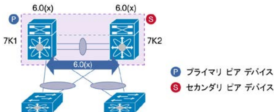
図 90. vPC の ISSU : ステップ 3
