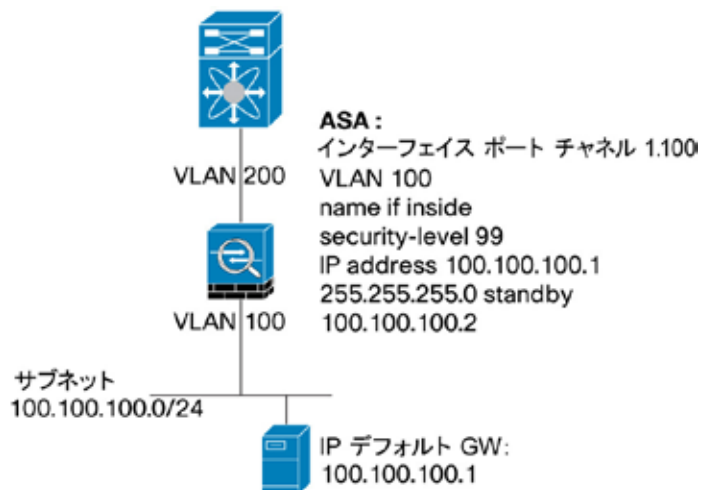
図 78. vPC ドメインに接続されているルーテッドモードの ASA : 論理構成図
