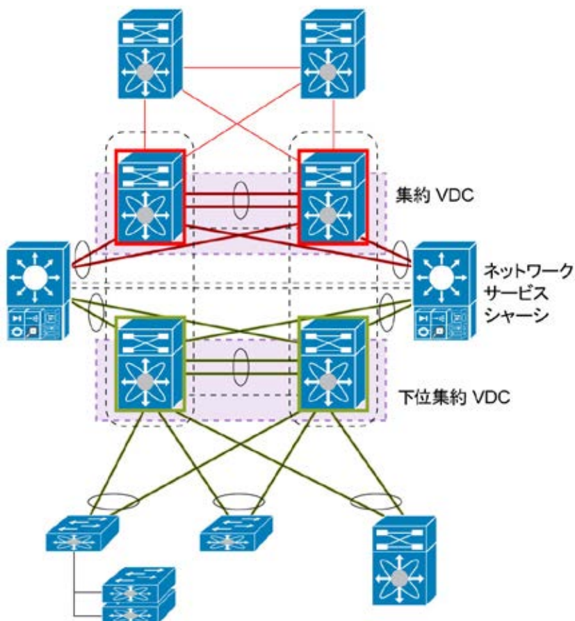
図 71. VDC サンドイッチ設計のネットワーク サービス シャーシ
