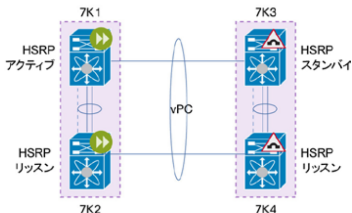
図 69. 単一 HSRP/VRRP グループの DCI : DC1 のアクティブ/アクティブおよび DC2 のリッスン/リッスン
