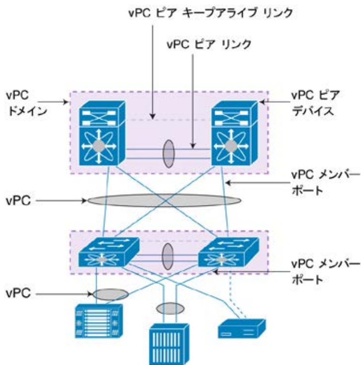
図 2. vPC コンポーネント
