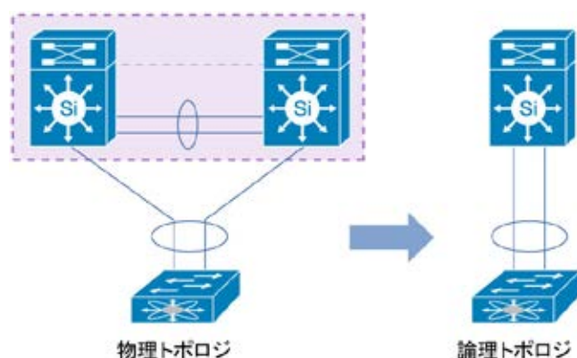
図 1. vPC (仮想ポート チャンネル) テクノロジーによる単一の論理ノードの作成
