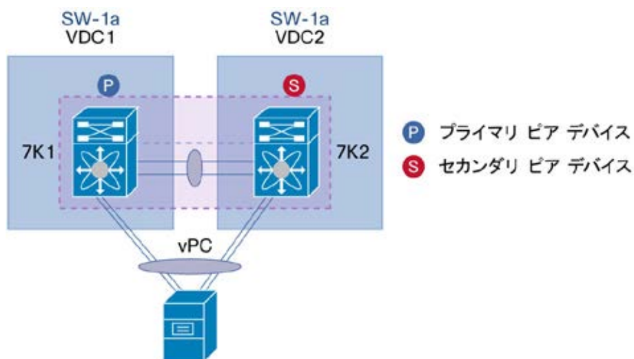
図 87. 2つの異なる VDC を使用して同じ NEXUS 7000 シャーシ内に作成された vPC ドメイン
