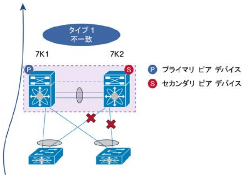
図 95. vPC グレースフル タイプ 1 チェック
