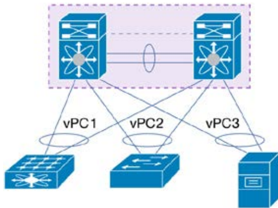
図 4. シングルサイド vPC トポロジ
