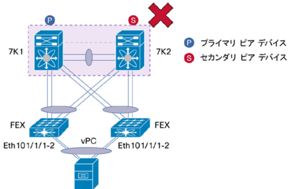
図 84. vPC の FEX : eVPC（拡張 vPC）：未サポート
