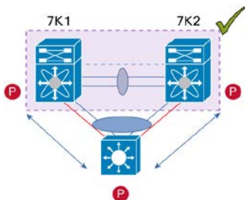
図 57. レイヤ 3 および vPC でサポートされる設計：パラレル相互接続ルーテッドポートでの外部ルータとのピアリング
