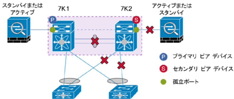
図 98. vPC 孤立ポートの一時停止
