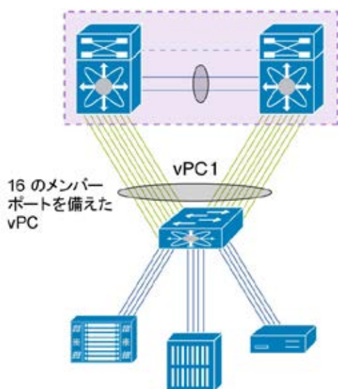
図 30. 16 方向のポート チャンネルを使用したシングルサイド vPC
