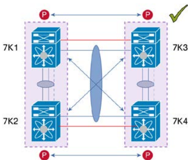
図 58. レイヤ 3 および vPC でサポートされる設計：パラレル相互接続ルーテッドポートでの vPC 相互接続 (DCI ケース) を介したピアリング
