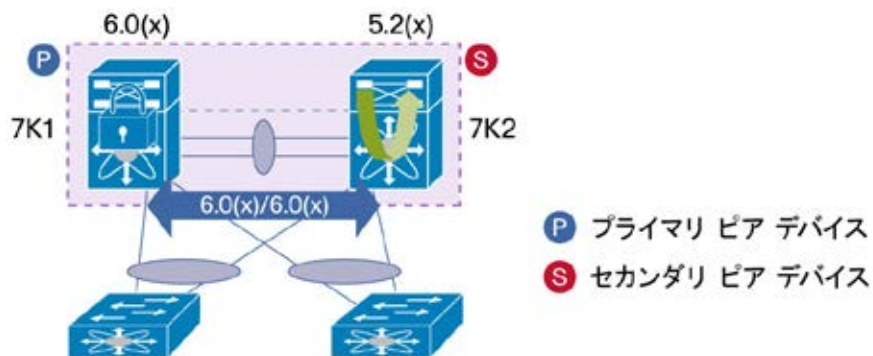
図 89. vPC の ISSU : ステップ 2
