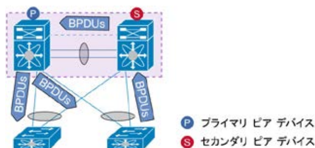
図 41. vPC およびスパンニングツリー プロトコル BPDU
