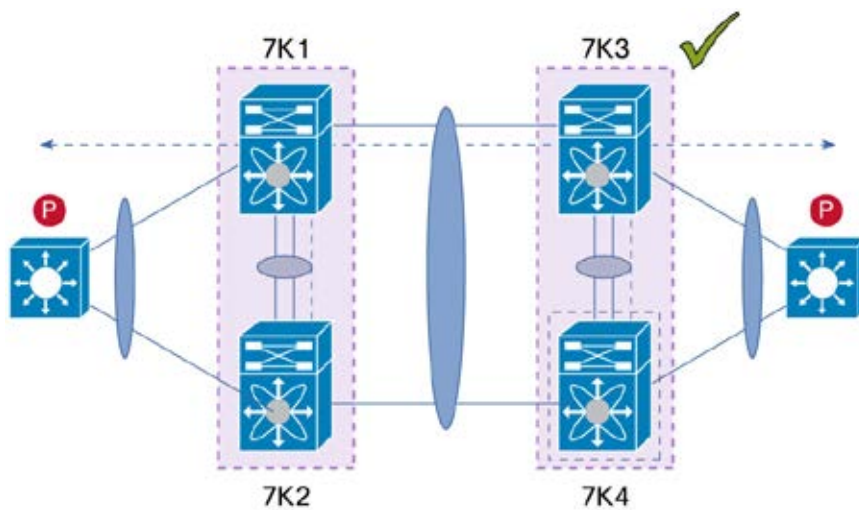
図 56. レイヤ 3 および vPC でサポートされる設計：中継スイッチとして vPC デバイスを使用した 2 ルータの間のピアリング
