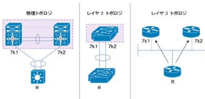
図 49. ネットワークのレイヤ 2 またはレイヤ 3 ビジョンに応じた vPC ピア デバイスの異なる構成図
