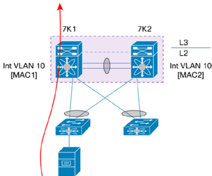
図 91. vPC ピア ゲートウェイ
