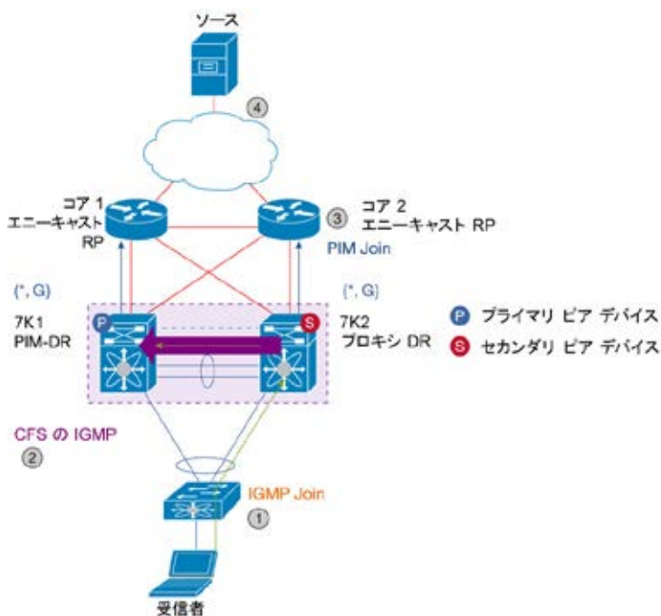
図 80. vPC でのマルチキャストの動作 (マルチキャスト パケット フロー)
