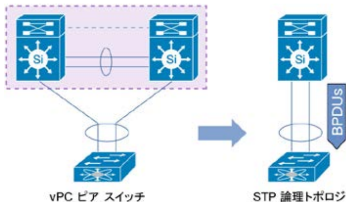
図 42. vPC ピア スイッチ
