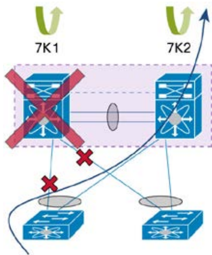
図 97. vPC 自動リカバリのリロード遅延 : vPC ピア デバイスがリロードし、7K2 のみ回復
