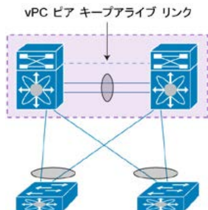
図 14. vPC ピア キープアライブ リンク
