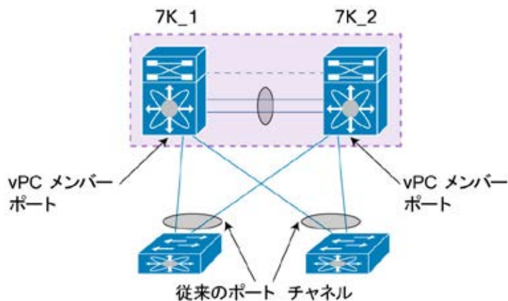
図 28. 従来のポート チャンネルおよび vPC メンバー ポート
