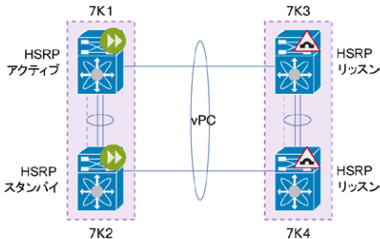
図 68. 単一 HSRP/VRRP グループの DCI : DC1 のアクティブ/アクティブおよび DC2 のリッスン/リッスン
