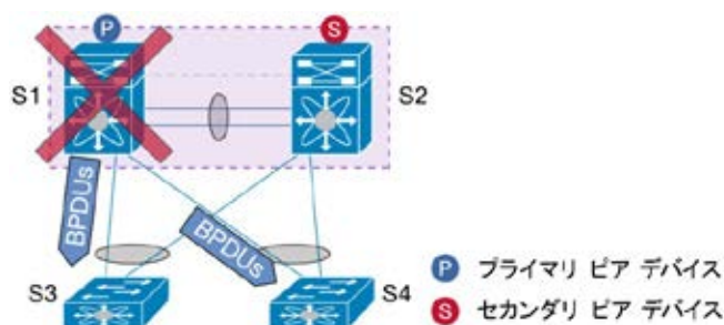
図 47. vPC での Bridge Assurance (BA) の使用
