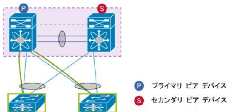
図 29. vPC ドメインにデュアル接続されたアクセス デバイス
