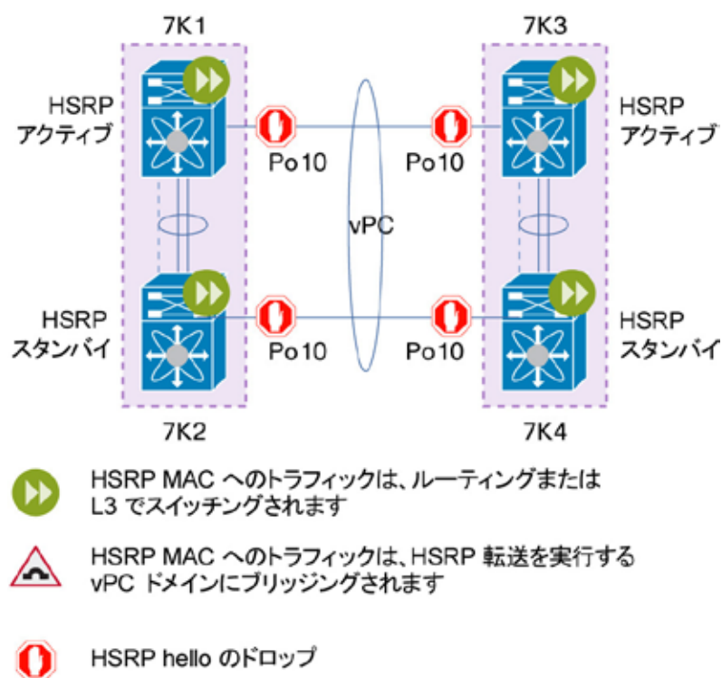
図 70. 単一 HSRP/VRRP グループの DCI : DC1 のアクティブ/アクティブおよび DC2 のアクティブ/アクティブ
