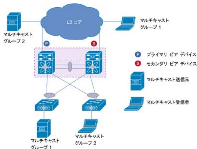
図 79. vPC でのマルチキャスト
