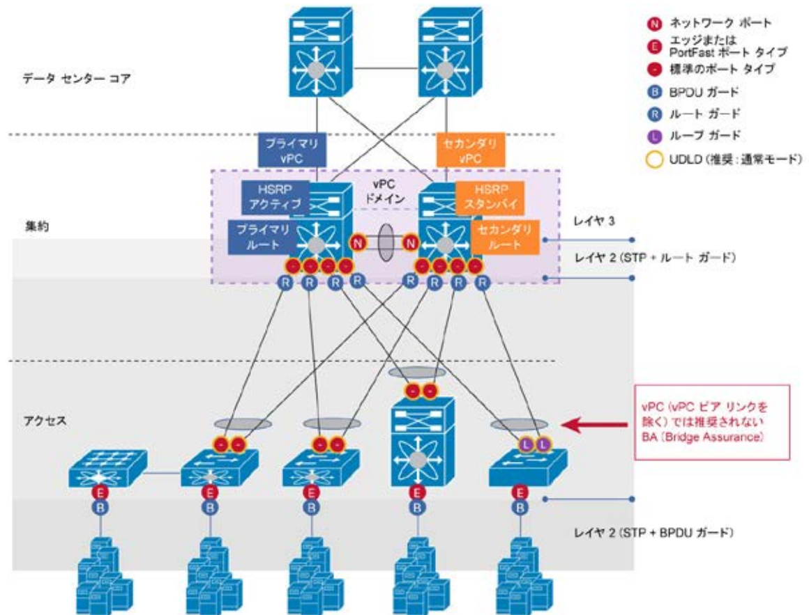
図 40. spanning-tree プロトコルおよび vPC：ポート設定の推奨事項
