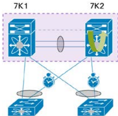
図 94. vPC の遅延復元 : 7K2 の障害および回復
